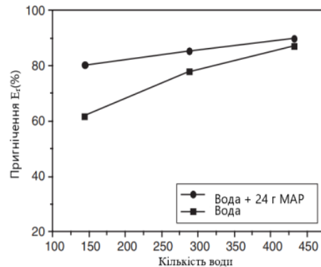
Рис. 2. Швидкість виділення енергії рекуперації горіння при використанні води та води з додаванням моноамоній фосфату. (MAP) [7]
