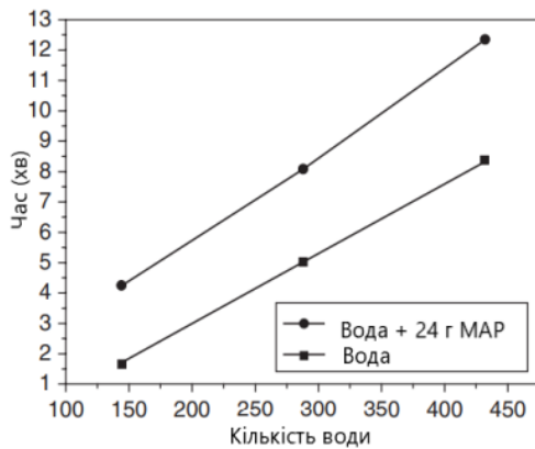
Рис. 1. Час до початку відновлення горіння при використанні води та води з додаванням моноамоній фосфату (MAP) [7]
