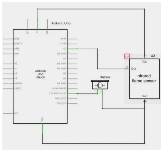
Рисунок 1– Схема підключення датчику вогню до плати Arduino
