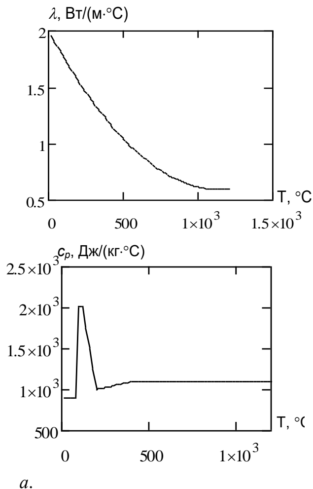
Рис. 5.5. Теплофізичні характеристики бетону: а – коефіцієнт теплопровідності; б – питома теплоємність.
