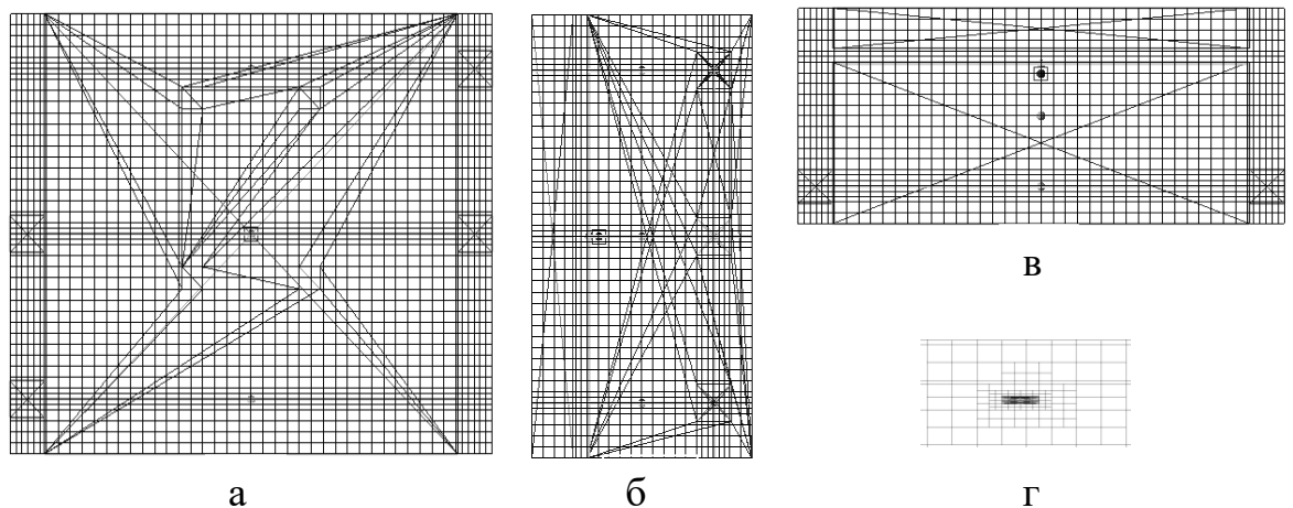
Рис. 2.4. Сіткова модель простору вертикальної печі Лаб. 2: а – вид по осі Y ; б – вид по осі X ; в – вид по осі Z ; г – адаптивна сітка для термopар (вид на бокову поверхню термopар).
