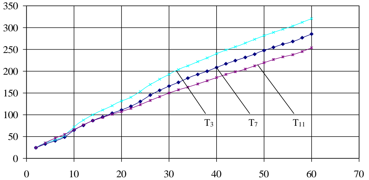
Рис. 2.11. Графік зміни температури в приарматурному шарі вертикальної конструкції при моделюванні випробувань у печі Лаб. 1: T_3 , T_7 , T_{11} – показники температури в різних частинах конструкції (рис. 7).
