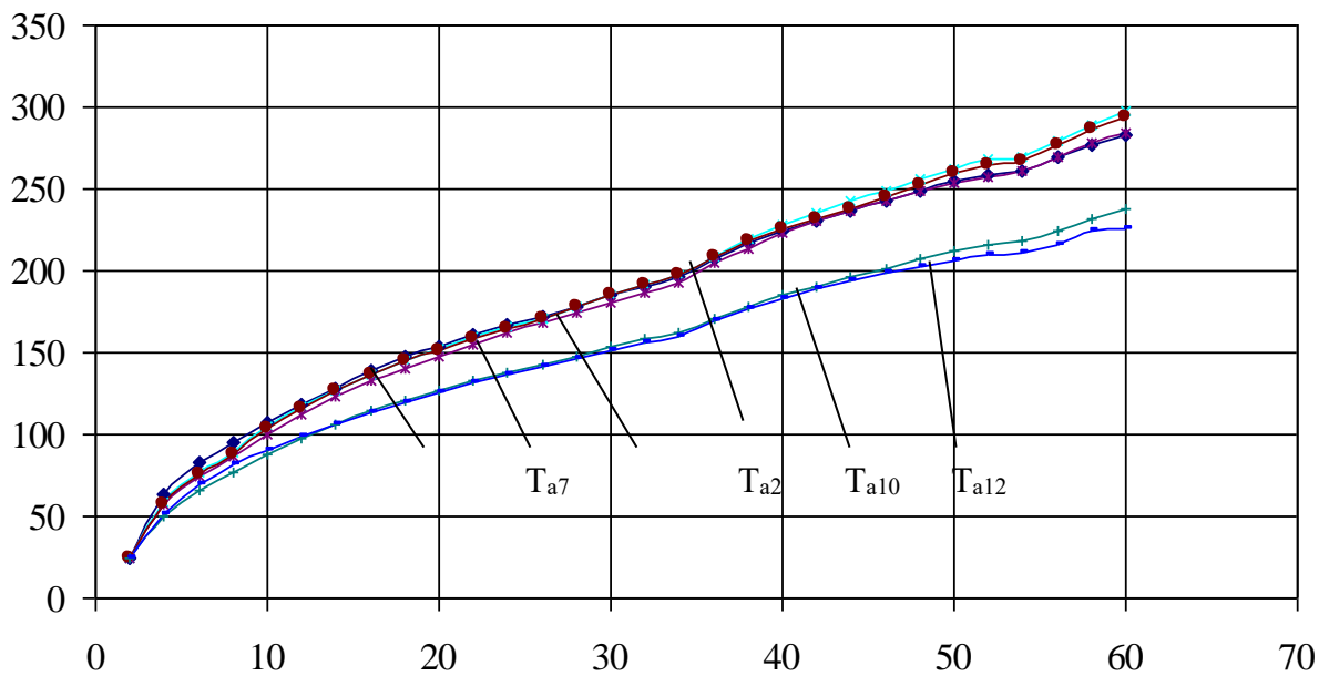
Рис. 2.12. Графік зміни температури в приарматурному шарі вертикальної конструкції при моделюванні випробувань у печі Лаб. 2: T_a , T_{a2} , T_{a4} , T_{a7} , T_{a10} , T_{a12} , – показники температури в різних частинах конструкції (рис. 8).
