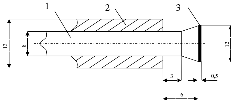
Рис. 1.3. Переносна термопара: 1 – захисний кожух; 2 – теплозахисна оболонка; 3 – мідний диск.
