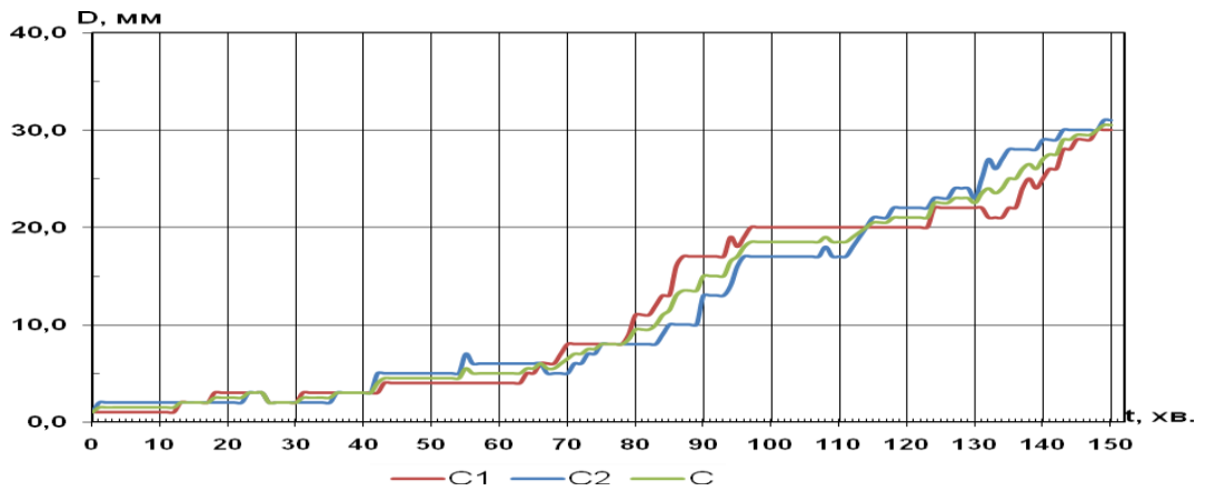
Рис. 3.6. Залежності вертикальної деформації зразка від часу.
