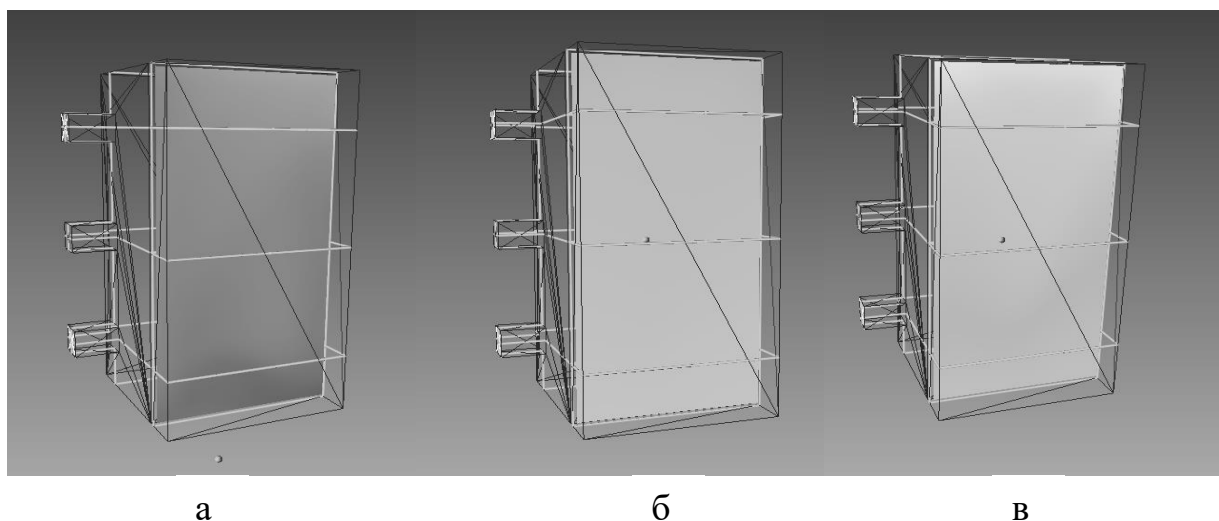
Рис. 2.13. Розподіл температур на обігрівальній поверхні плити: а – 10-та хвилина випробувань; б – 30-та хвилина випробувань; в – 60-та хвилина випробувань.
