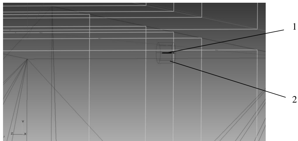
Рис. 2.5. Циліндричний регіон адаптації сітки для термопар в камері печі: 1 – модель термопар; 2 – циліндричний регіон адаптації.
