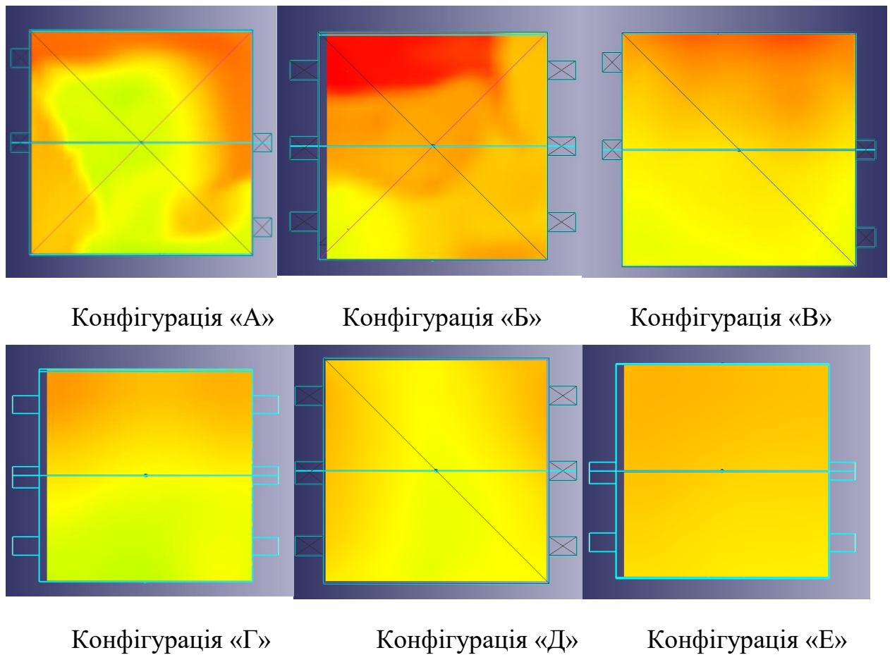
Рис. 4.2 – Градієнт температур по обігрівальній поверхні змодельованих конструкцій.
