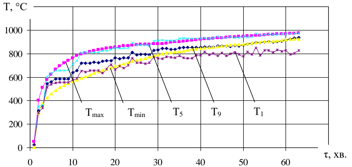
Рис. 2.9. Графік зміни температури в різних місцях камери печі Лаб. 1: T_{\max} – верхня межа випробувань; T_{\min} – нижня межа випробувань; T_5 – показники температури у верхній частині печі; T_9 – показники температури в середній частині печі; T_1 – показники температури в нижній частині печі (рис. 2.6).
