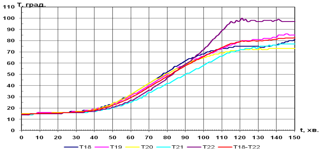
Рис. 3.4. Залежності температури від часу на необігрівальній поверхні зразка.
