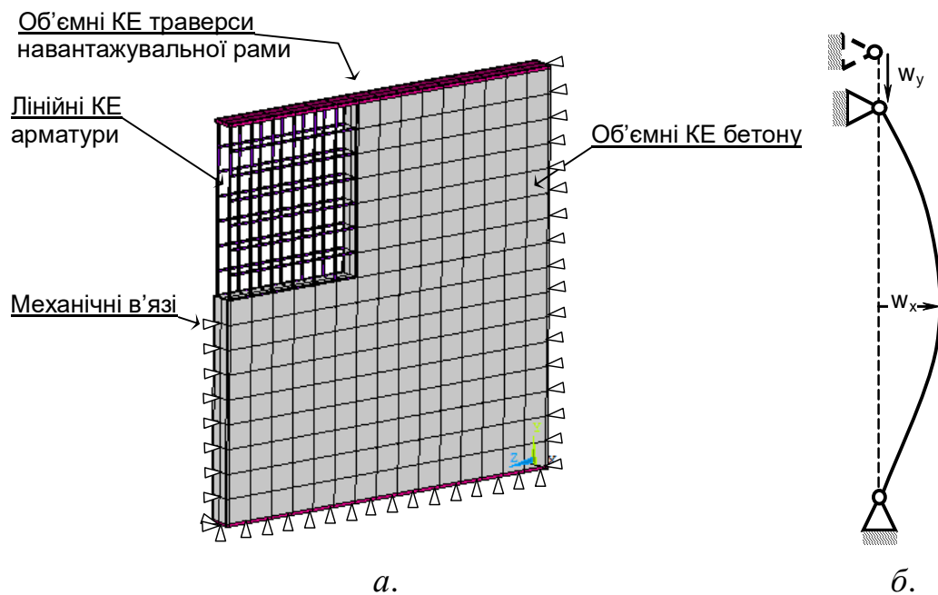
Рис. 5.10. Кінцево-елементна схема залізобетонної стіни та накладеній на її вузли механічні в'язі (а) та розрахункова схема закріплення стіни (б).
