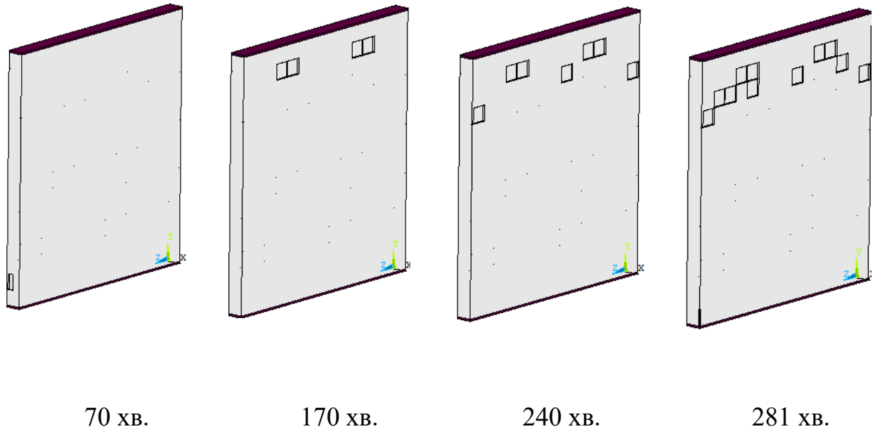
Рис. 5.13. Положення повністю роздроблених кінцевих елементів у залізобетонній стіні у різні моменти часу її вогневих випробувань
