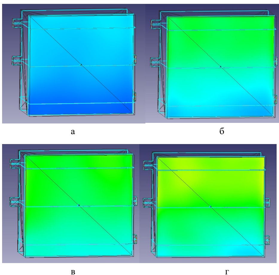
Рис. 2.14. Розподіл температур на обігрівній поверхні плити: а – 10-та хвилина випробувань; б – 30-та хвилина випробувань; в – 60-та хвилина випробувань.
