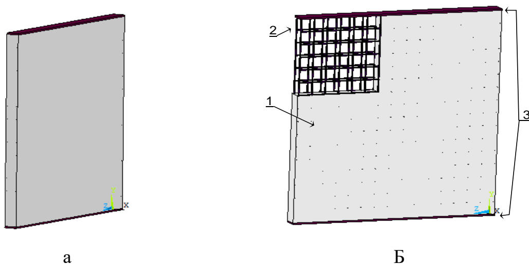
Рис. 5.1. Схема розрахункової області залізобетонної несучої стіни для проведення розрахунку межі вогнестійкості (а – загальний вигляд, що використовують під час обчислювального експерименту, б – схема армування): 1 – бетон, 2 – робочий арматурний каркас d = 16 мм, 3 – траверси навантажувальної рами.
