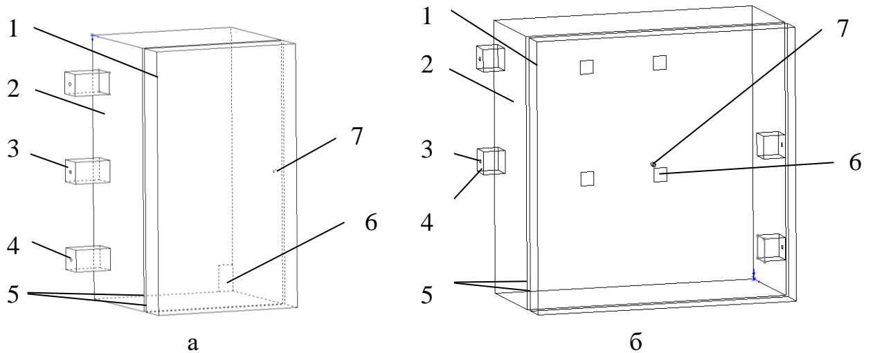
Рис. 2.1. Геометрична конфігурація вертикальних печей (а – ПП «Випробувальний центр «ТЕСТ» (далі – Лаб. 1) (зображено лише симетричну половину) та б – ТОВ «ПожТест» (далі – Лаб. 2): 1 – огороження печі; 2 – фрагмент стіни; 3 – регіон вдуву; 4 – регіон форсунки; 5 – поверхні, що сполучаються; 6 – регіон виходу продуктів горіння; 7 – розрахункова область термопар.
