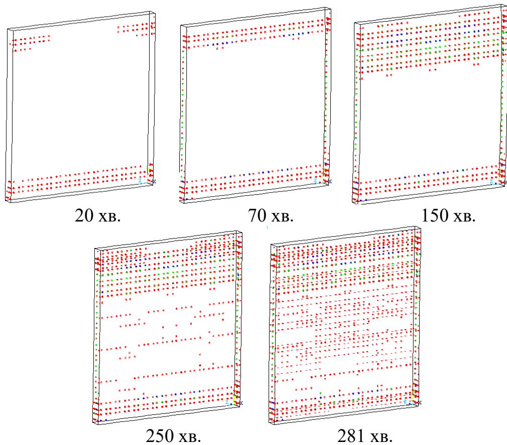
Рис. 5.11. Розподілення тріщин у залізобетонній стіні у різні моменти часу випробування
