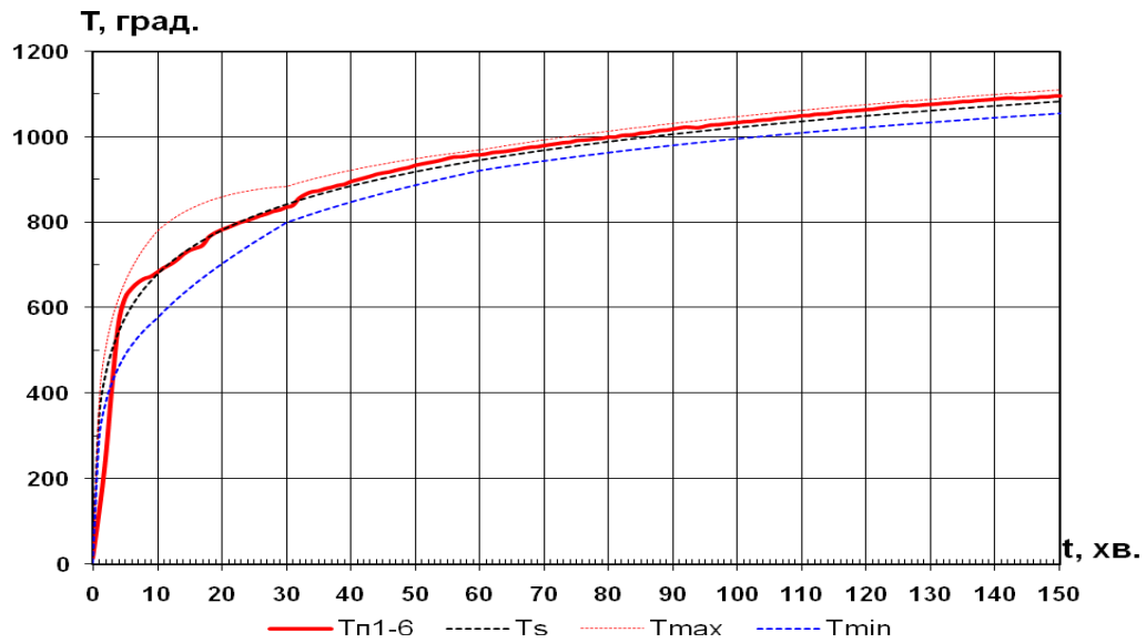
Рис.3.3 Температурний режим в печі під час випробування зразка.
