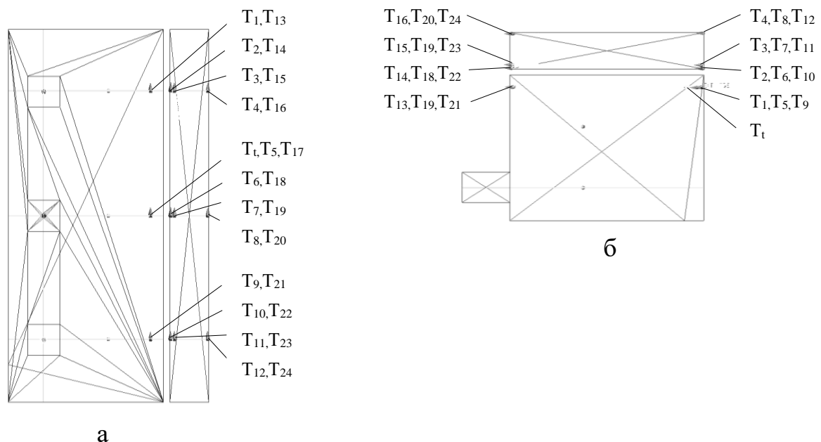
Рис. 2.6. Місця де відбувався контроль температури при моделюванні печі Лабораторії 1 (показано лише симетричну половину): T_t , T_1 - T_{24} – місця де відбувалося зняття температури; а – вид по осі X; б – вид по осі Z;.
