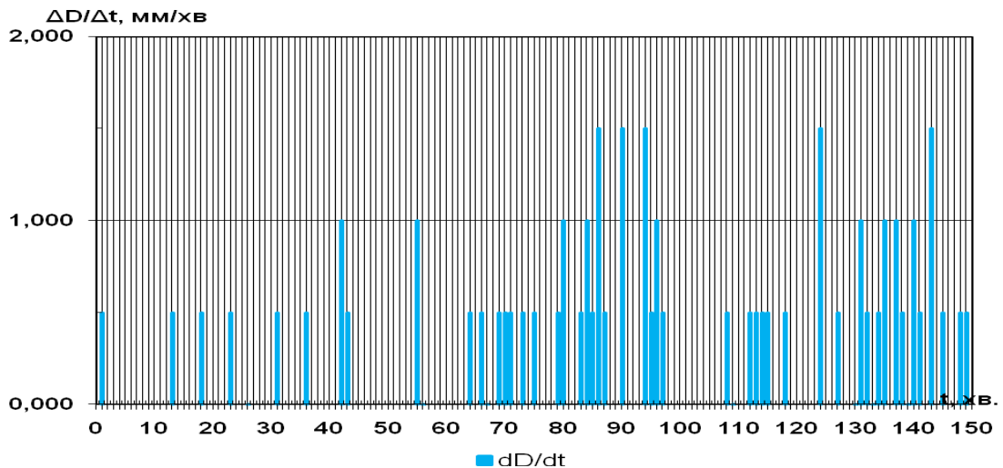
Рис. 3.7. Залежність поздовжнього зміщення навантаженого кінця зразка від часу зразка.
