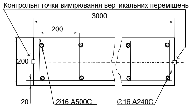
Рис. 5.2. Геометрична конфігурація перерізу залізобетонної стіни.
