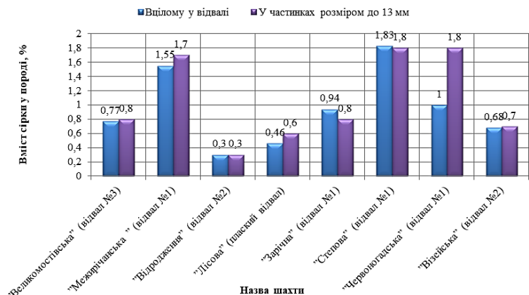
Рисунок 3.18 – Середній вміст сірки у породі не діючих відвалів
