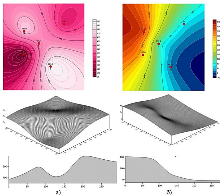
Рисунок 3.36 – Поширення \text{Cu} ( \text{мг/кг} ) у едафічних горизонтах породного відвалу шахти «Надія»: а) 0-15 \text{см} ; б) 0-20 \text{см}
