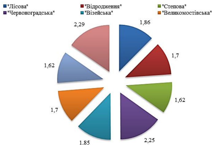
Рисунок 3.16 – Об'ємна густина породи діючих відвалів т/м³
