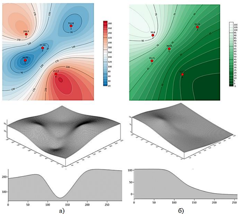
Рисунок 3.34 – Поширення \text{Co} (мг/кг) у едафічних горизонтах породного відвалу шахти «Надія»: а) 0-15 см; б) 0-20 см
