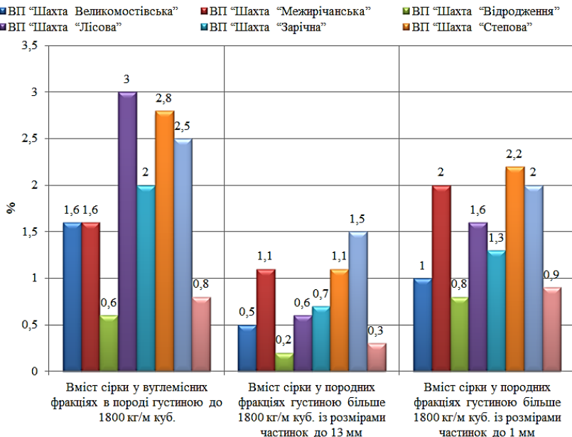
Рисунок 3.22 – Вміст сірки в породних відвалах залежно від гранулометричного складу та густини породи
