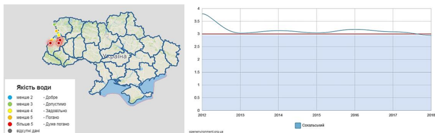
Рисунок 3.40 – Показники якості води у басейні річки Вісла (територія функціонування Львівсько-Волинського вугільного басейну) та біологічне споживання кисню (БСК) у водоймах Сокальського району Львівської області
