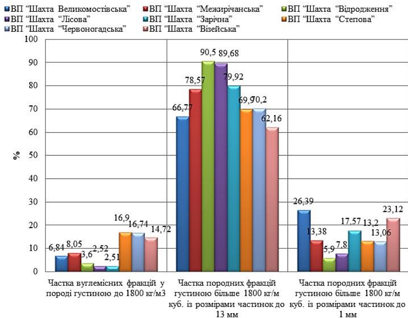
Рисунок 3.20 – Частки вуглемісних та породних фракцій в породних відвалах
