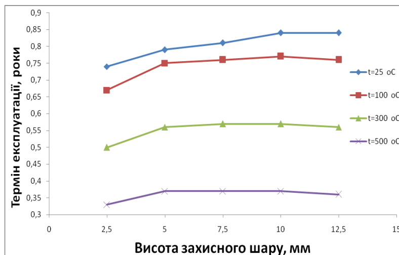
Рис. 1. Залежність терміну експлуатації мембрани від висоти захисного шару при різних температурах експлуатації: t=25 °С; t=100 °С; t=300 °С; t=500 °С.
