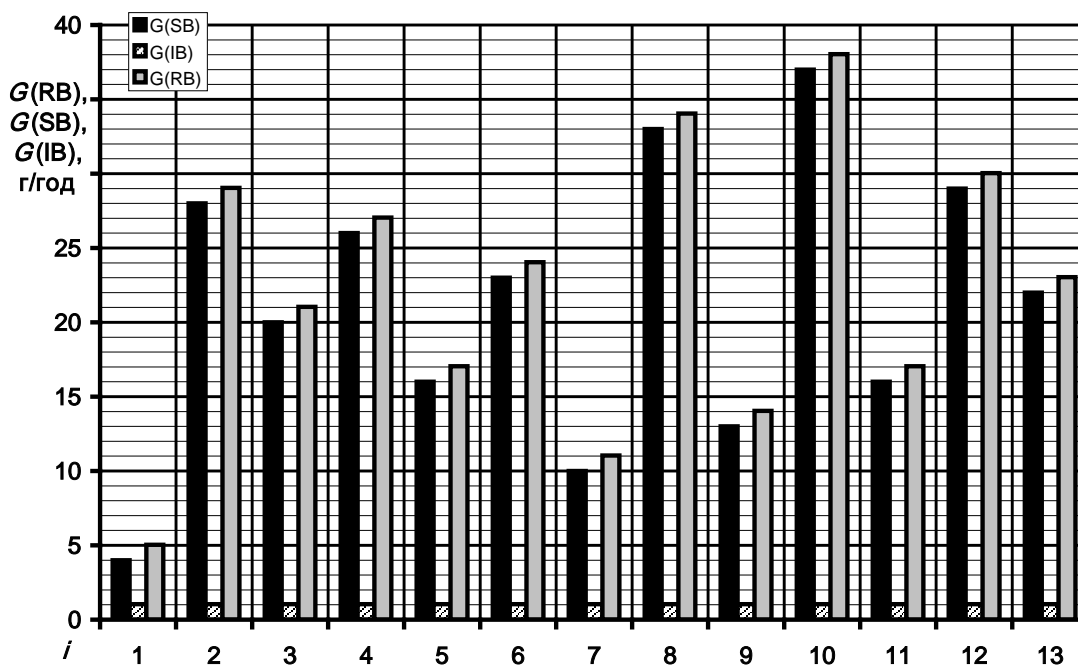
Рисунок 2. Розподіл величин значень G(RB) , G(SB) та G(ІВ) по режимах випробувального циклу ESC для автотракторного дизеля 2Ч10,5/12
