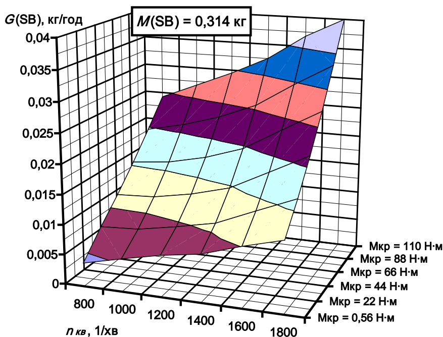
Рисунок 1. Розподіл величин значень G(SB) по області режимів роботи автотракторного дизеля 2Ч10,5/12
