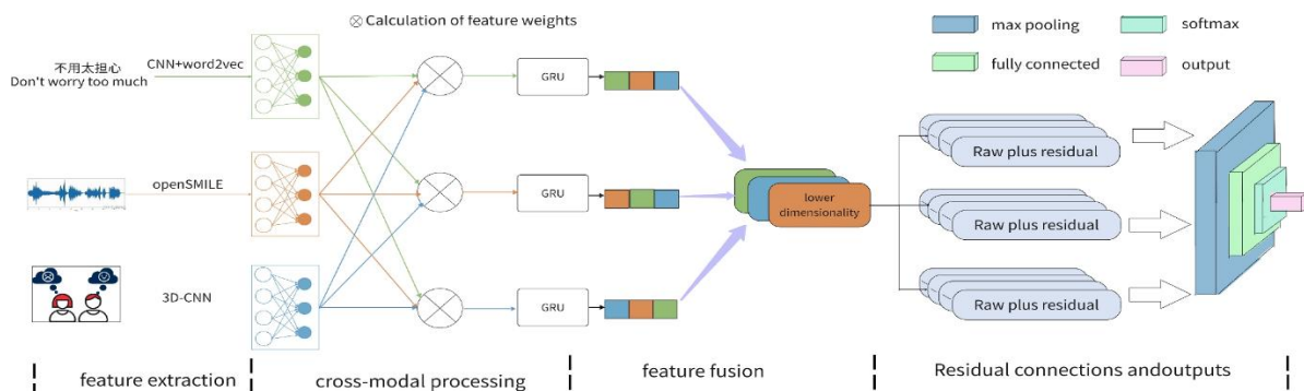
Рис. 1. Архітектура гібридної мультимодальної моделі з механізмами крос-модальної уваги для класифікації емоцій
