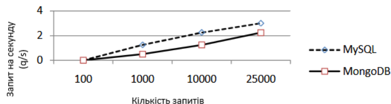
Рис. 4 Insert запити за секунду у відношенні на збережені записи у MySQL та MongoDB
