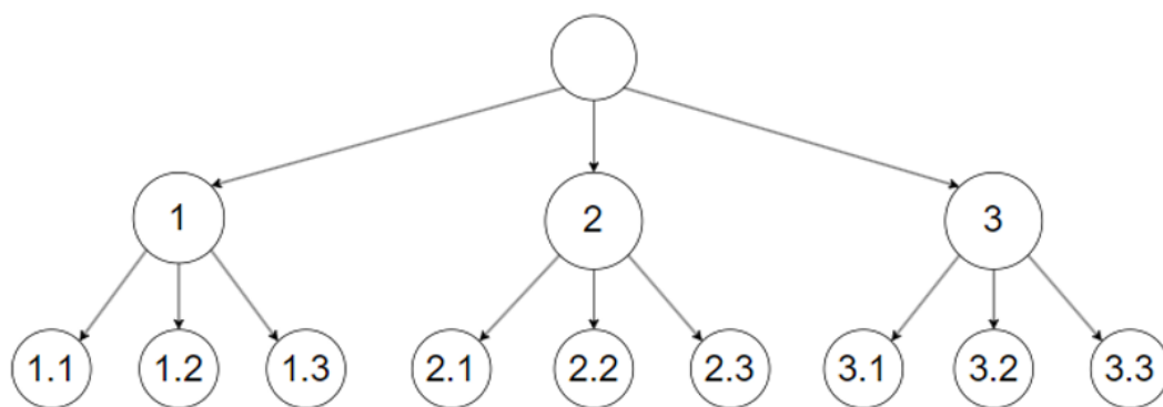
Рис. 1 Дерево проблем
