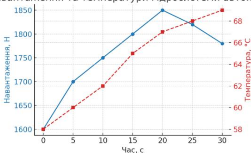
Зміна навантаження та температури гідросистеми автокрана у часі
