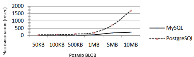
Рис. 1 Виконання BLOB insert запитів у MySQL та PostgreSQL
