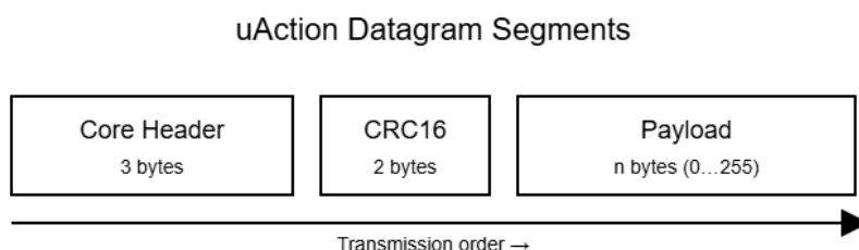
Рис. 2. Формат пакета uAction
