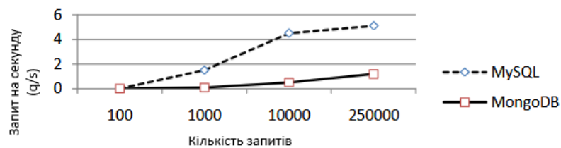
Рис. 3 Select запити за секунду у відношенні на повернені записи у MySQL та MongoDB
