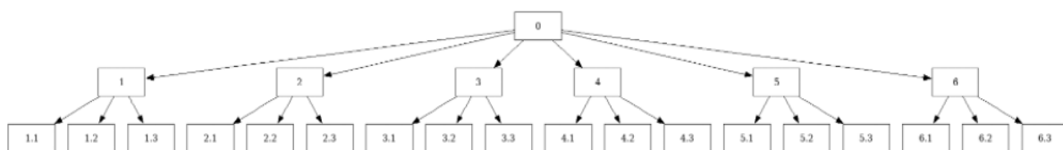
Рис. 2 Дерево цілей
