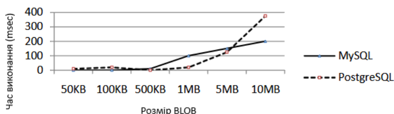
Рис. 2 Виконання BLOB select запитів у MySQL та PostgreSQL
