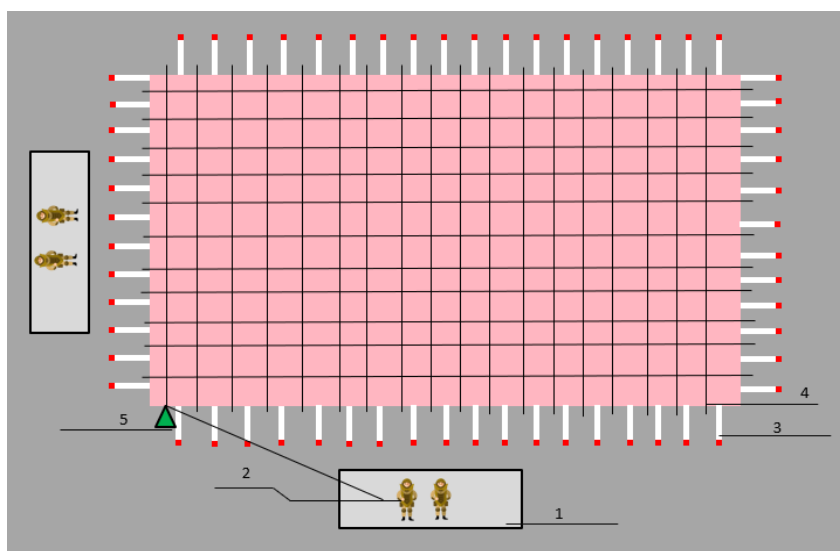
Рис. 1. Розроблена схема тралення 1 – окоп, 2 – сапер (піротехнік), 3-маркування небезпечної території, 4- маршрут тралення, 5 – механізм для зміни напрямку тралення
