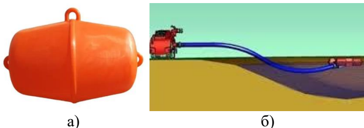
Рис. 1. Принцип використання буя: а) «поплавков» для всмоктуючої сітки; б) практичне використання «поплавка» при заборі води з водойми
