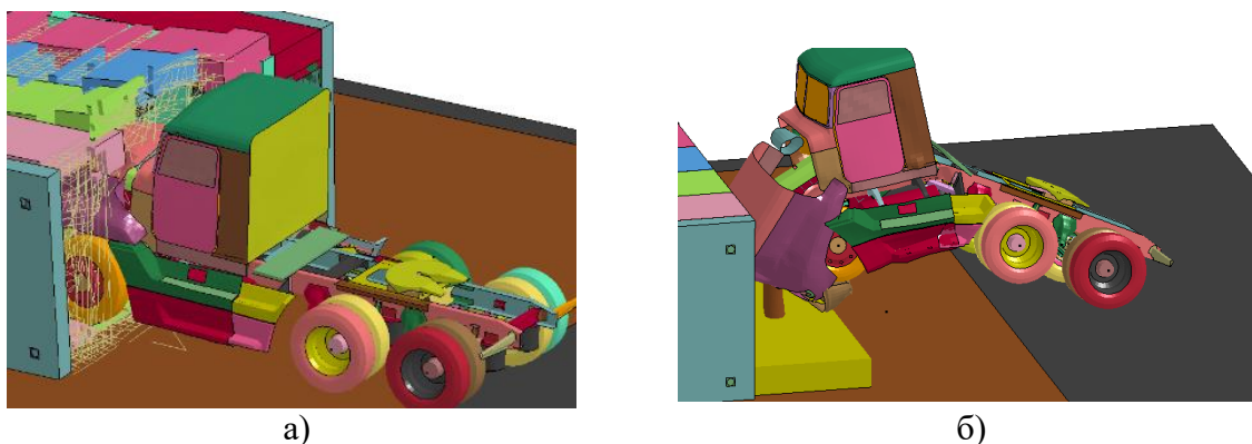
Рис. 1. Зіткнення автомобіля з модульним укриттям (а) та із захисною системою (б).
