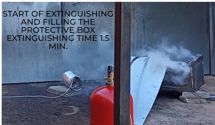
Рисунок 1 – Модельне вогнище з випробування вогнегасних речовин для гасіння літій-іонних акумуляторів
