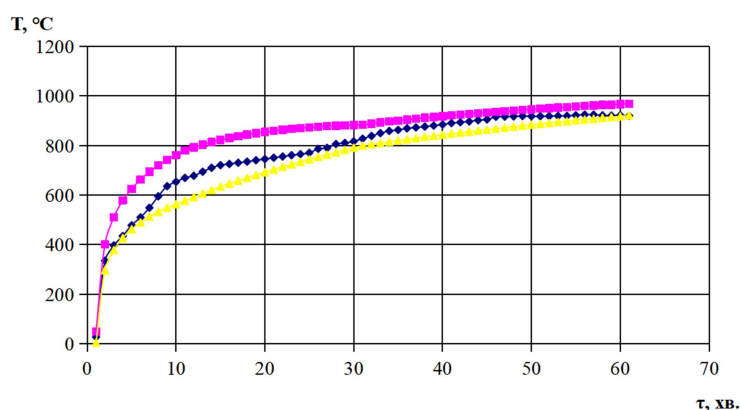
Рисунок 2 – Лінійна швидкість нагрівання камери печі під час нагрівання фрагменту залізобетонної колони: T_{\min} , T_{\max} – граничні межі випробувань за стандартним температурним режимом пожежі; T_{\text{ср}} – середній показник термопар у ході вогневих випробувань у камері вогневої печі
