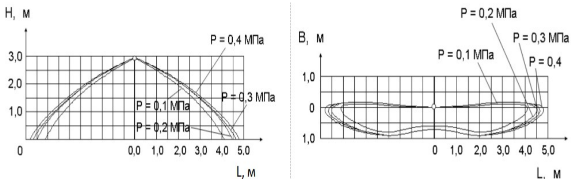
Рисунок 2 – Епюра та карта зрошення зрошувача «Завіса»
