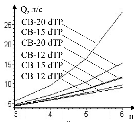
Рисунок 2 – Залежність витрати ріdkої ВР від кількості зрошувачів на рядку РМ
