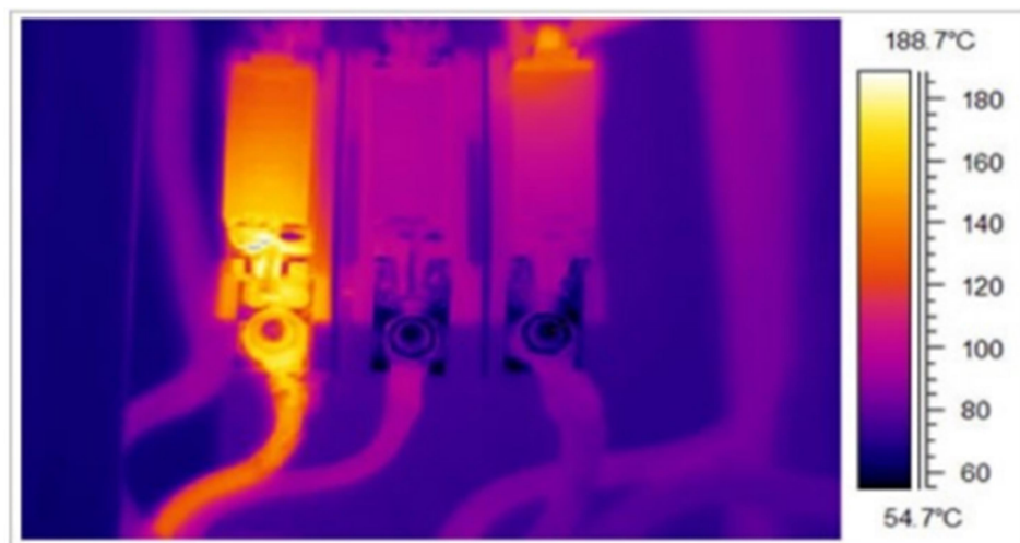
Рисунок 1 – Приклад термограми апаратів захисту та провідників з перегрівом
