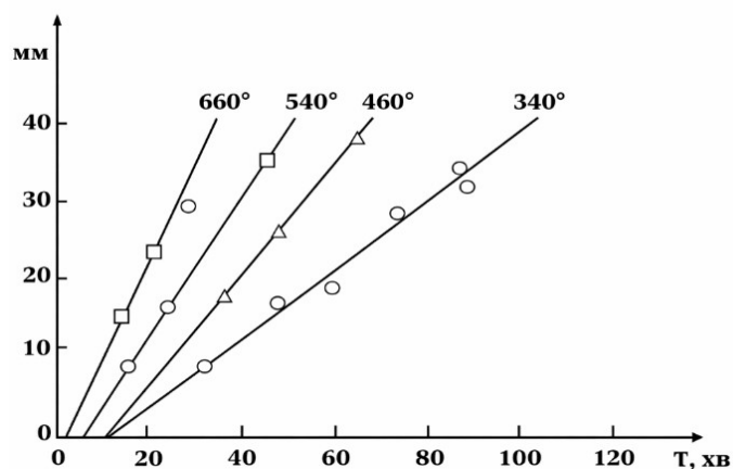
Рисунок 1 – Глибина обвуглювання деревини
