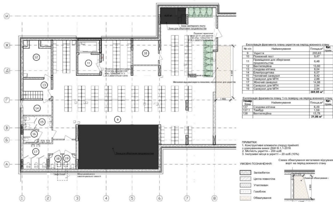
Рисунок 1 – Схема приміщення захисної споруди цивільного захисту
