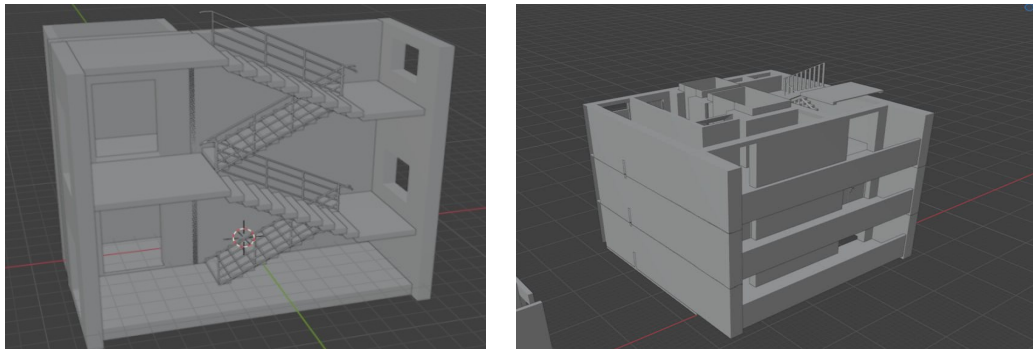
Рисунок 1 – Приклад моделювання сходових кліток типу СК1, Н1
