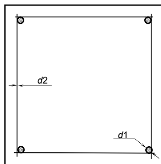
Рисунок 1 – Схема армування фрагменту для проведення випробування, де: d_1 – робоча арматура більшого діаметру, d_2 – робоча арматура меншого діаметру
