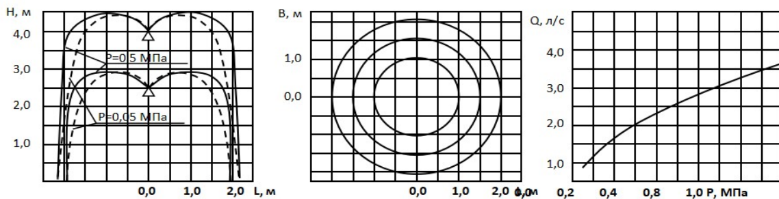
Рисунок 1 – Епюра та карта зрошення зрошувача ДВВ-10
