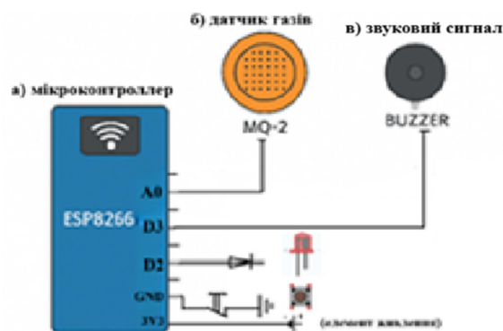
Рисунок 1 – Схема побудови пристрою (портативного смарт-детектора небезпечних газів)
