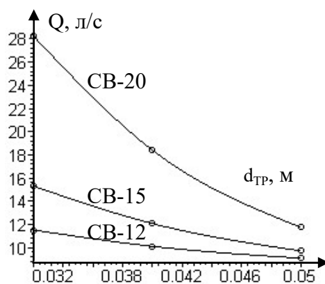
Рисунок 1 – Залежність витрати ріdkої ВР від діаметра рядка РМ
