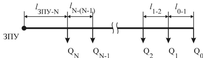
Рисунок 1 – Схема живильного і розподільчого трубопроводу дренчерної системи водяного пожежогашіння.
