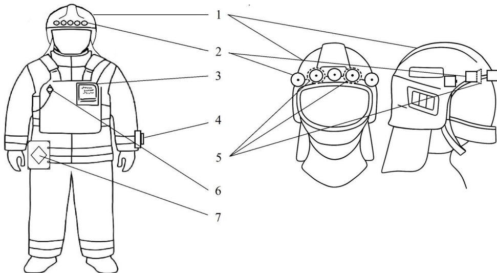
Рисунок 1 – Схема будови системи для орієнтування в середовищі з незадовільним візуальним контролем
