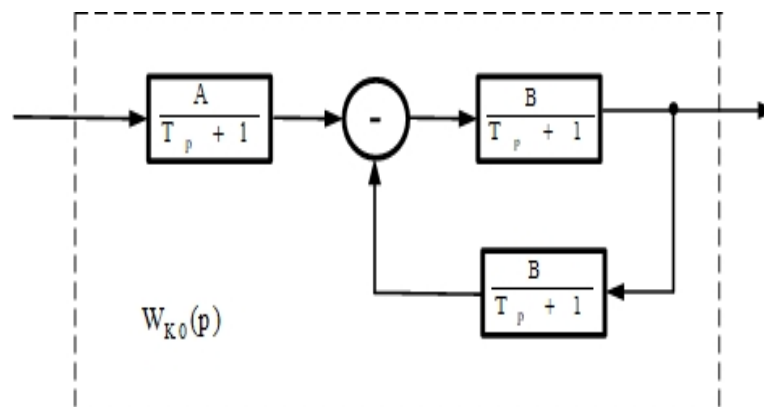
Рисунок 1 – Структурно динамічна схема динамічного елемента із передаточною функцією
