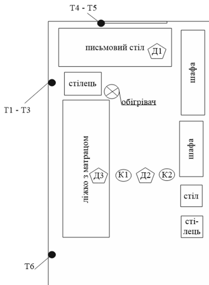
Рисунок 2 – Схему приміщення та місця встановлення засобів метрології: Т1–Т6 – термопари; Д1–Д3 – димові пожежні сповіщувачі; К1–К2 – теплові пожежні сповіщувачі
