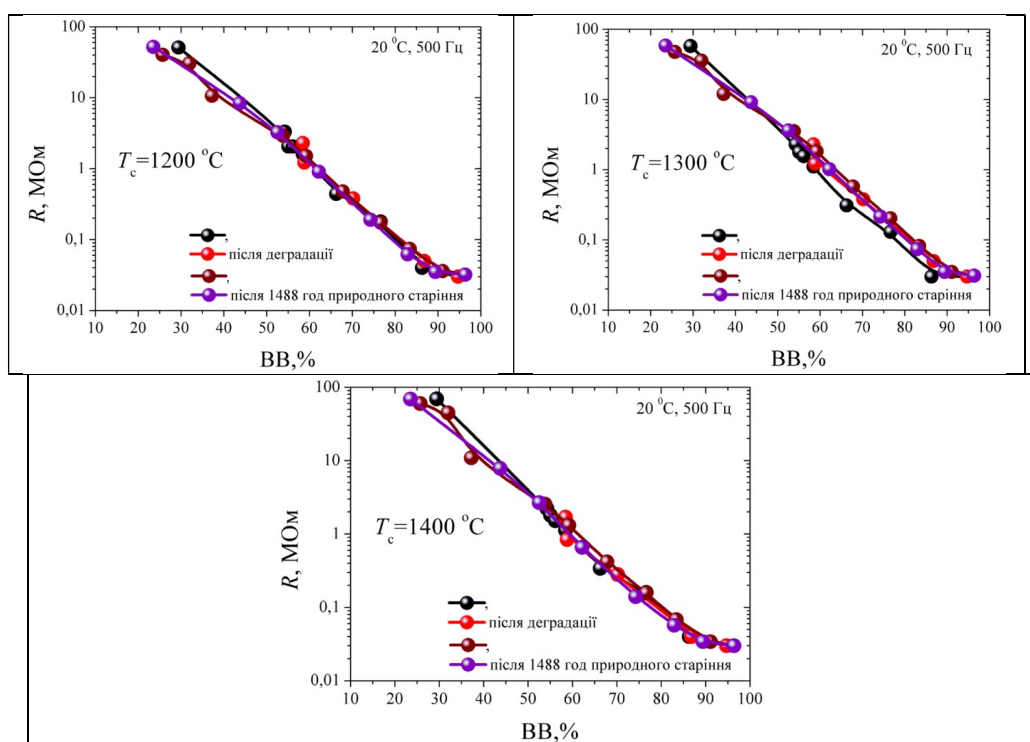
Рисунок 1 – Порівняння залежностей опору від відносної вологості для кераміки \text{MgAl}_2\text{O}_4 , спеченої за 1200, 1300 та 1400°C, одержаних після деградаційних випробувань (240 год. за 40°C та BV = 95\% ) та природного старіння (температура вимірювань 20°C, частота вимірювань 500 Гц)
