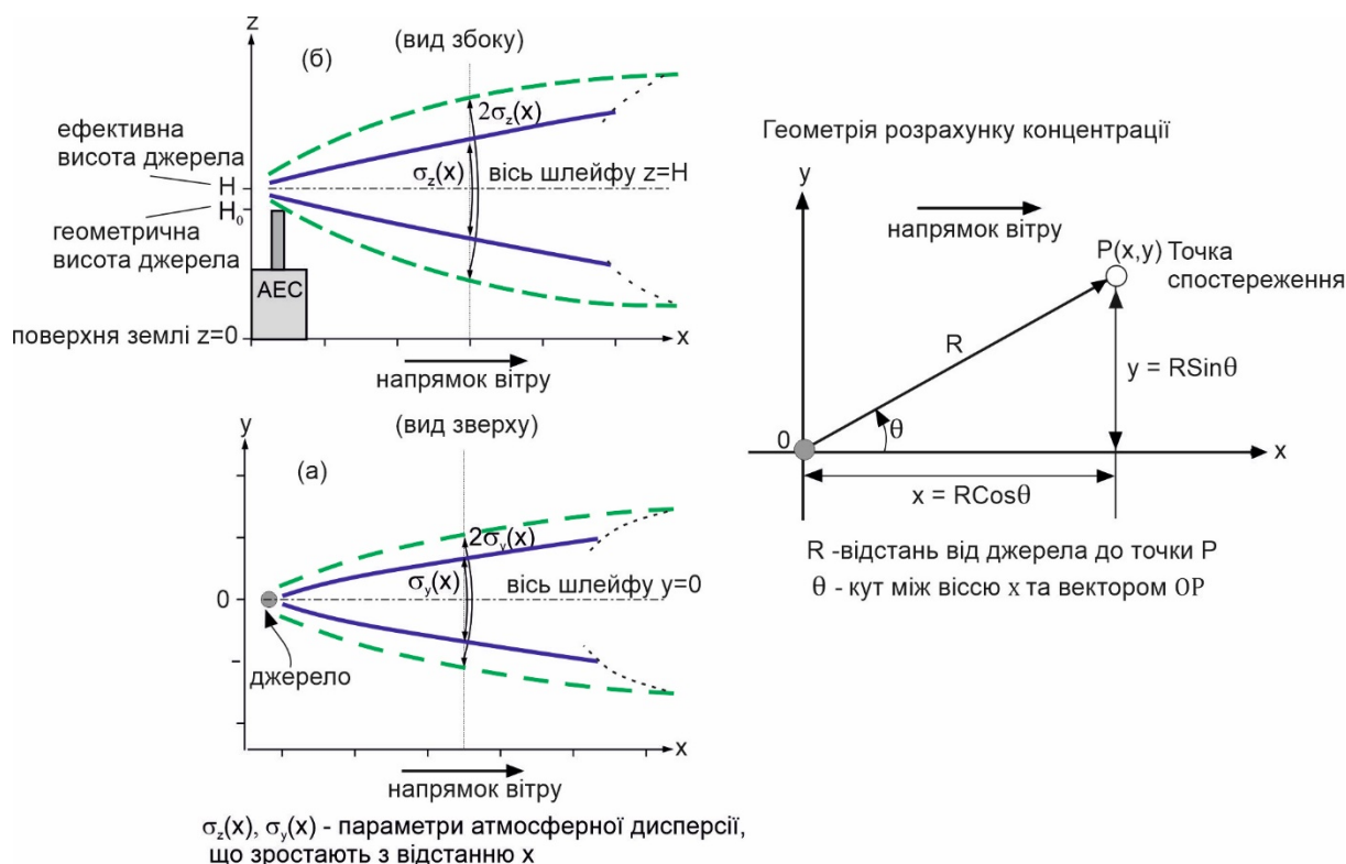
Рисунок 1 – Схема поширення радіоактивного шлейфу в гаусовій моделі атмосферної дифузії: (а) горизонтальний переріз шлейфу в площині x-y ; (б) вертикальний переріз у площині x-z ; праворуч - геометрія визначення координат точки спостереження. Параметри \sigma_y(x) і \sigma_z(x) є стандартними відхиленнями гаусового розподілу концентрації домішки у поперечному та вертикальному напрямках, відповідно. Величини 2\sigma_y(x) і 2\sigma_z(x) умовно характеризують ширину шлейфу, в межах якої зосереджена основна частина домішки (для гаусового розподілу – близько 95 %).
