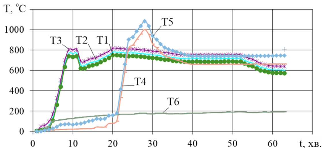
Рисунок 4 – Температурний режим під час пожежі у житловому приміщенні в зимовий період
