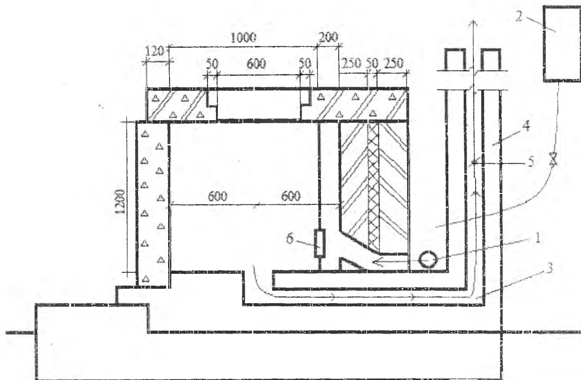
Рис. 2. Конструктивна схема роботи печі для вогневих випробувань фрагментів будівельних конструкцій та вогнезахисних покриттів: 1- паливна форсунка; 2- бак з паливом; 3- димовий канал; 4- димохід; 5- засувка; 6- розсікач полум'я
