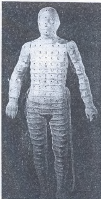
Рисунок 3 - Манекен, який використовується для випробувань захисного одягу.
