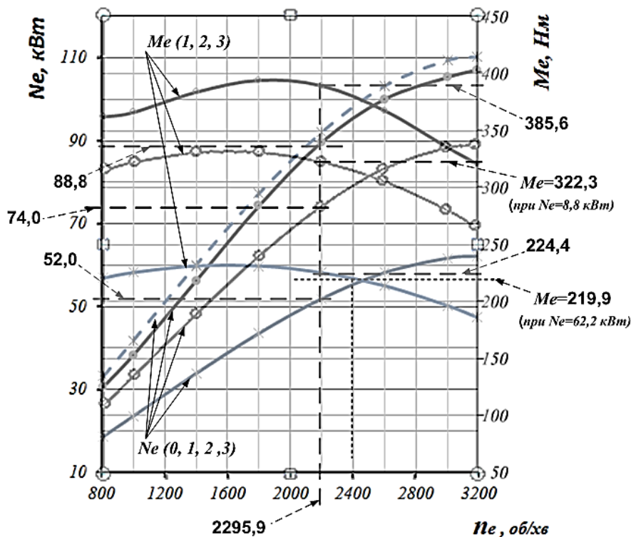
Рис.5. Розрахункові параметри зовнішньої та часткової швидкісних характеристик двигуна автомобіля ЗиЛ-131: 0 - при Ne = 110 кВт; 1 - при Ne = 107 кВт; 2 - при Ne = 88,8 кВт; 3 - при Ne = 62,2 кВт;
