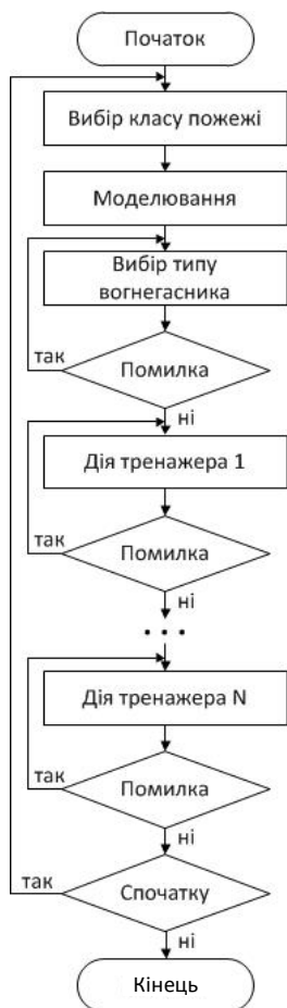
Рисунок 3 – Алгоритм дії тестування з використанням мобільної інтерактивної діалогової
