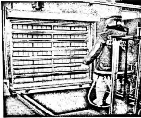
Рисунок 1 – Стенд теплових панелей, який використовується для випробування захисного одягу
