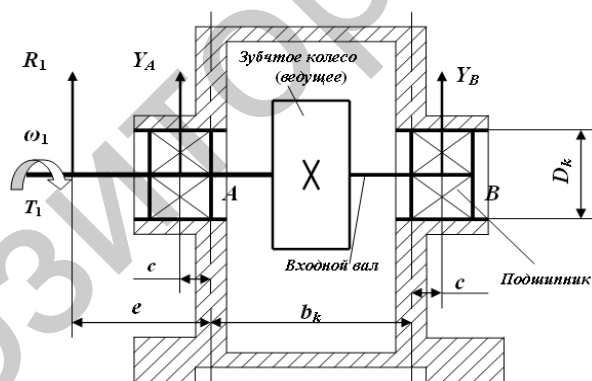
Рис. 2 – Поперечное сечение корпуса редуктора и схема его нагружения
