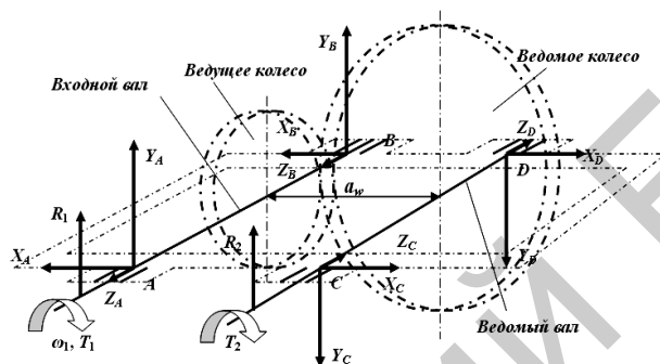
Рис. 1 – Схема нагружения одноступенчатого редуктора
