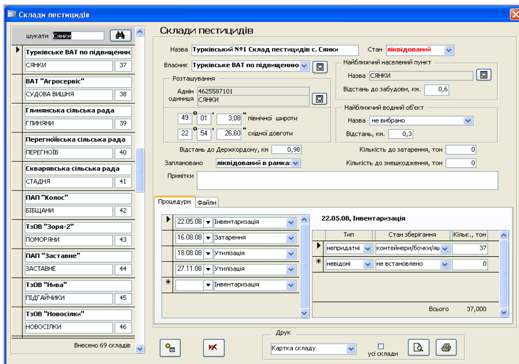
Рис.2. Елемент бази даних складів пестицидів.
