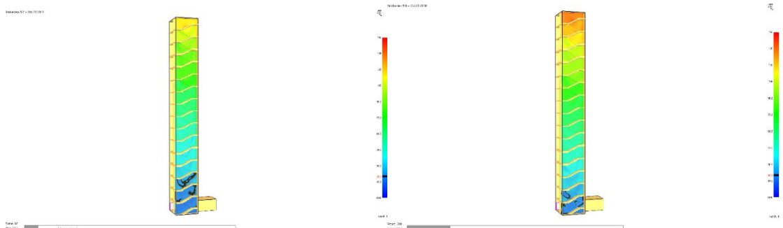
Рис. 3. – Поля давлений в лестничной клетке Н2 на 60 и 180 секундах (черная зона – зона давления 20 Па).
