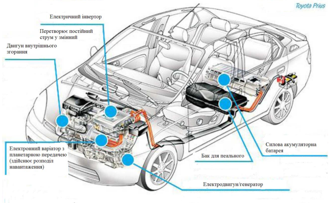
Рис. 1. – Схема гібридного авто.
