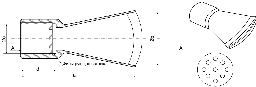
Рисунок 1 – Насадок на пожарный лафетный ствол для распыления ОВ плоскими струями
