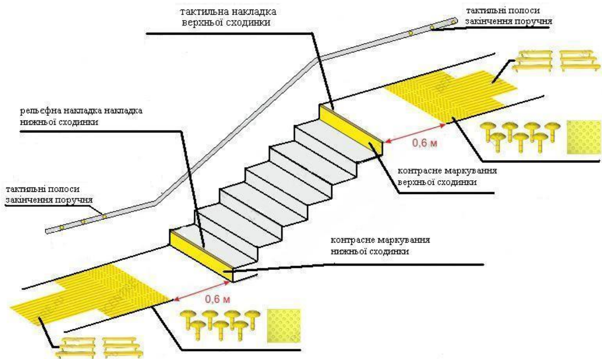
Рисунок 1 – Схема влаштування рельєфно-точкових індикаторів.
