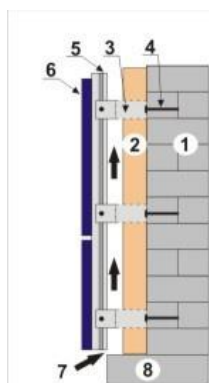
Рис. 3. Типова схема вентильованої фасадної безпеки.
