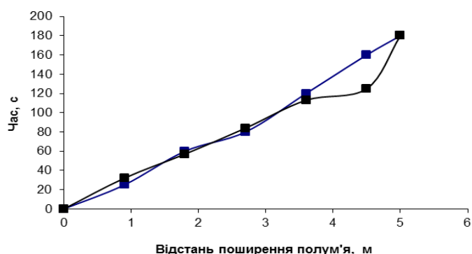
Рис. 2 Залежність відстані поширення полум'я від часу горіння
