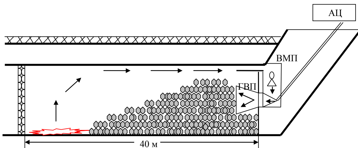
Рис. 2. Схема ізолюваної ділянки дослідної штольні для проведення експериментів по подачі піни на основі продуктів горіння
