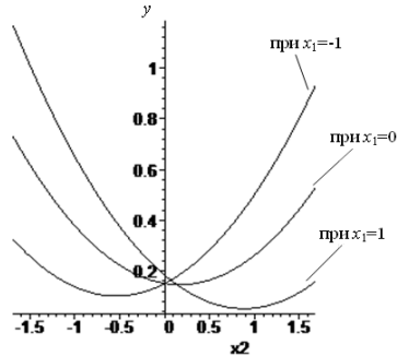
Рис. 1 – Залежність втрат напору в рукаві y від відстані між манометрами x_2 при напорі в мережі x_1 на мінімальному, середньому та максимальному рівнях
