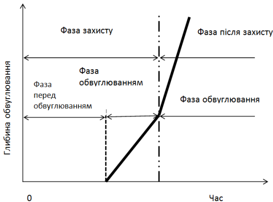
Рис. 1. Фази обвуглювання захищеної деревини
