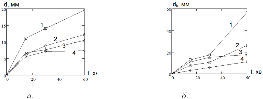
Рис. 3. Залежності бічних (а) і торцевих товщин (б) обвугленого шару від часу експонування зразків: 1 – без просочення; 2 – з вогнезахисним просоченням I типу; 3 – з вогнезахисним просоченням II типу; 4 – з вогнезахисним просоченням III типу.
