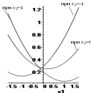
Рис. 2 – Залежність втрат напору в рукаві y від напору в мережі x_1 при відстані між манометрами x_2 на мінімальному, середньому та максимальному рівнях
