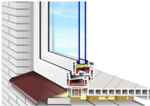
Рисунок 1. Віконні системи та складові до неї
