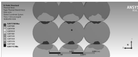
Рисунок 4 – Места подверженные наибольшему температурному воздействию при деформации (модель в разрезе)
