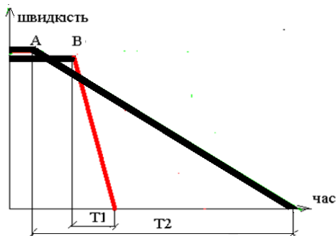
Рисунок. Моделювання зіткнення автомобіля із огороженням та бетонною стіною, де A – зіткнення із огорожею, B – зіткнення із бетонною опорою, T2 – час руйнування огорожі, T1 – час дії на людину при зіткненні із бетонною опорою.
