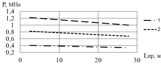
Рис. 2. Залежність необхідного тиску на ПКК від довжини розмотаної з котушки частини рукава та витрати на пожежогашіння:
