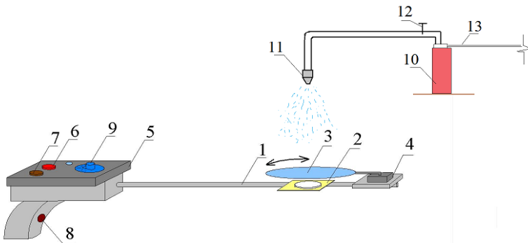
Рис. 1. Загальна схема пробовідбірника крапель тонкорозпиленої ВВР.
