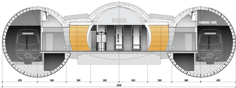
Рисунок 25.1 - Триплатформні станції
