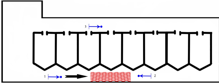
Рисунок 16.3 - Черговість та напрямки введення стволів під час гасіння пожежі в підсилосному приміщенні
