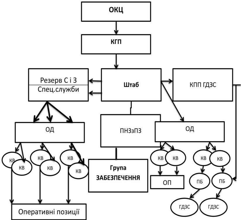
Рисунок 8.3 - Система управління силами та засобами на пожежі при створенні штабу.
