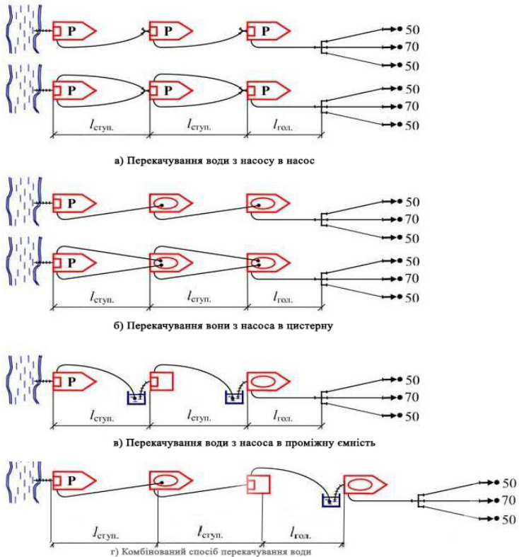
Рисунок 10.1 - Способи перекачування води на пожежу
