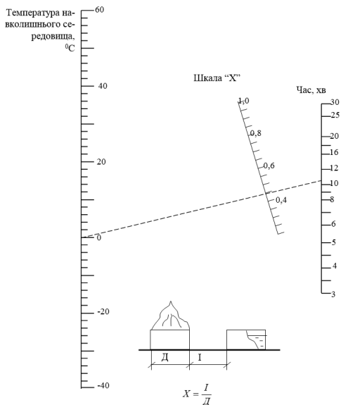
Рисунок 17.2.2 – Номограма для визначення максимально припустимого часу введення сил і засобів для охолодження резервуарів, які розташовані поряд з резервуаром, що горить
