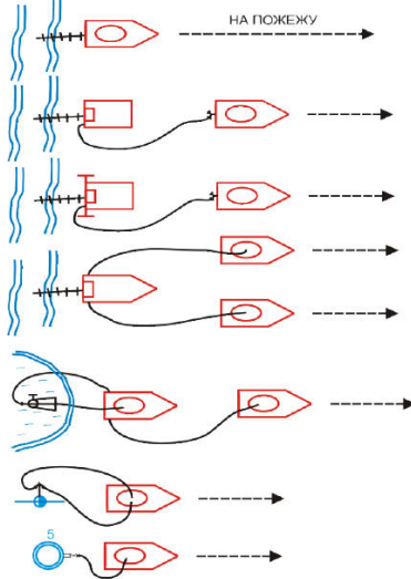
Рисунок 10.3 - Основні способи заправки автоцистерн від вододжерел
