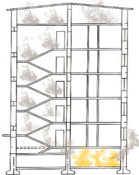
Рисунок 11.2 - Задимлення сходової клітини при пожежі в підвалі
