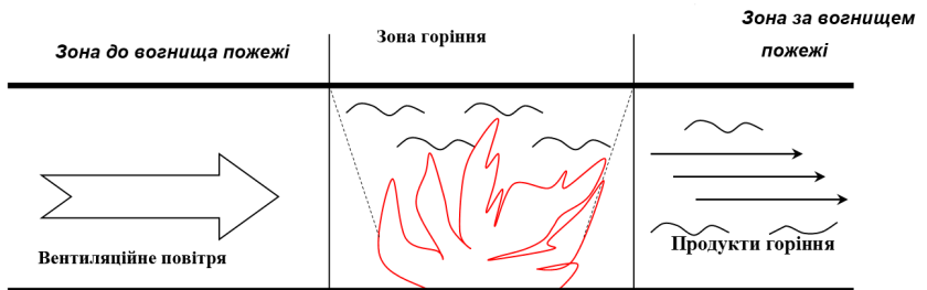
Рисунок 25.2 - Схема поширення пожежі в тунелі
