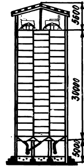
Рисунок 16.1. - Силосний корпус у розрізі.
