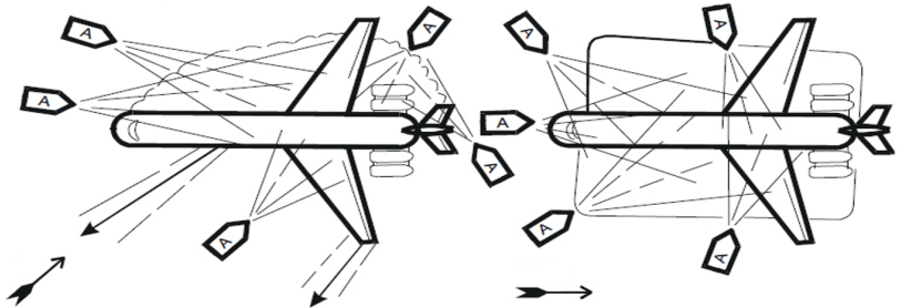
Рисунок 26.1 - Схеми гасіння пожежі розлитого авіаційного палива
