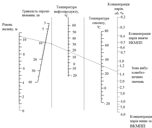
Рисунок 17.2.3 – Номограма для визначення вибухонебезпеки середовища в резеруарі, розташованого поряд з резервуаром, що горить
