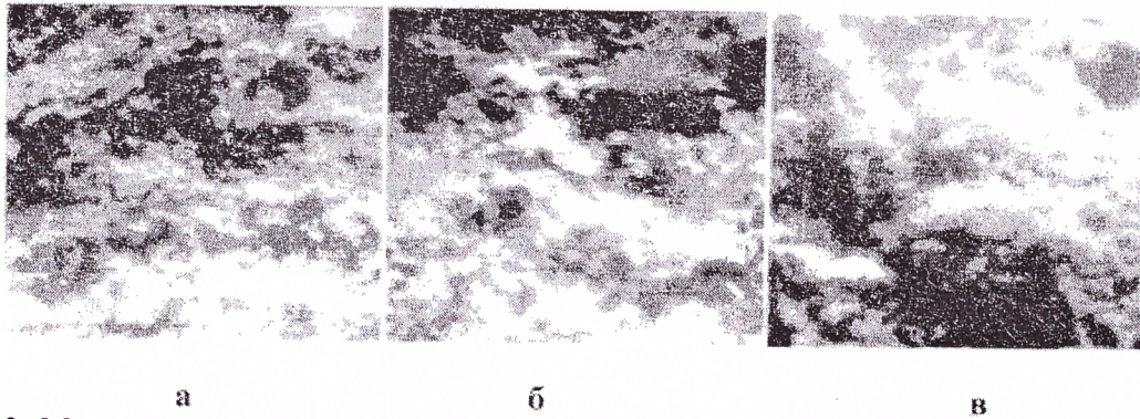
Рис. 2. Мікроструктура поверхні захисного покриття (склад № 5) після випробувань: а – вихідна; б – у сухих умовах; в – у вологих умовах (x 1000)
