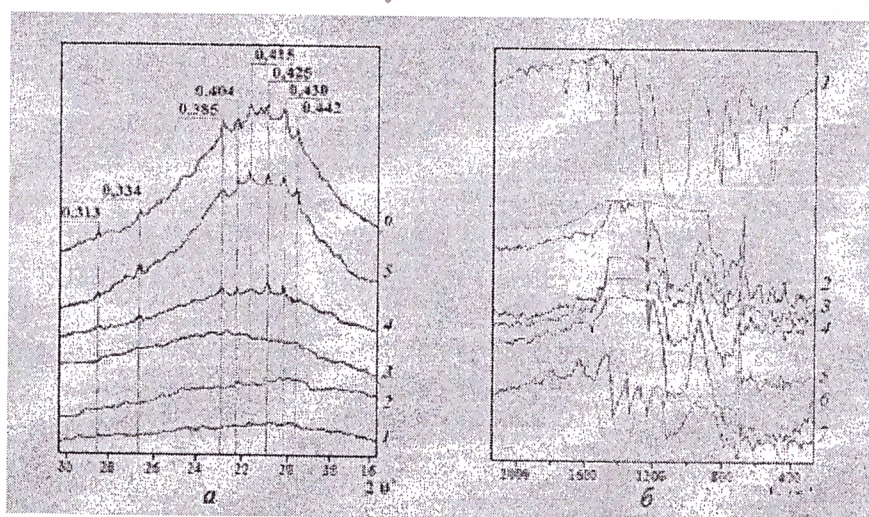
Рис. 1. Результати рентгенофазового аналізу (а) та ГЧ-дослідження (б): а – ПМФС в процесі нагрівання в інтервалі 273 (1)...1373 (6) К; б – композиції КО-08-Al 2 O 3 - ZrO 2 в процесі механо-хімічної обробки.
