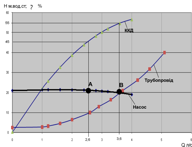
Рисунок – 2 Спільна робота насоса та внутрішнього протипожежного водопроводу
