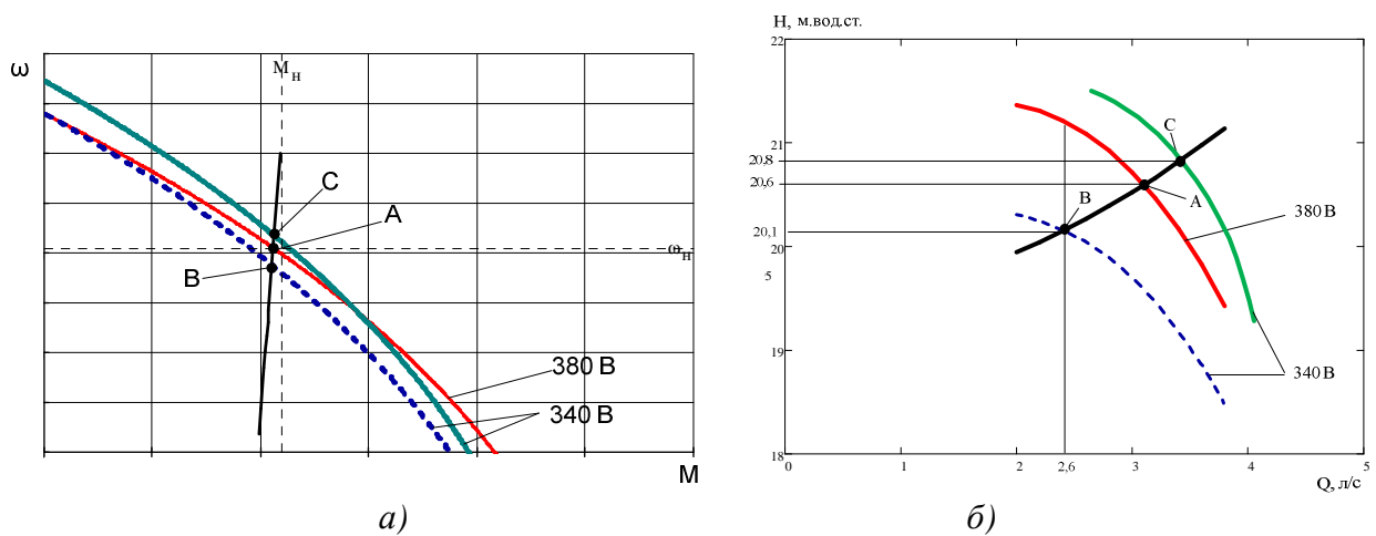
Рисунок –б а) залежність кутової швидкості АД від моменту (точка С при f=50,5\text{Гц} ); б) робоча точка внутрішнього протипожежного водопостачання (точка С при f=50,5\text{Гц} )
