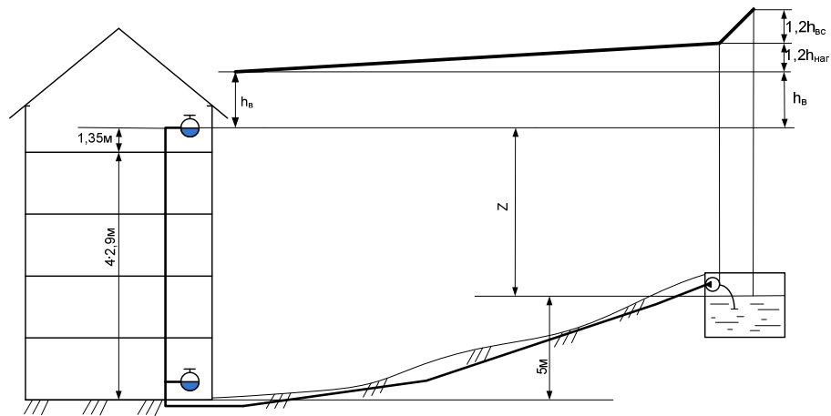
Рисунок – 1 Схема водопровідної мережі: h_B – висота компактної частини струменя (6 м); h_{НАГ} – висота підйому води у нагнітальній мережі (7,95 м); h_{BC} – висота підйому води у всмоктувальній мережі
