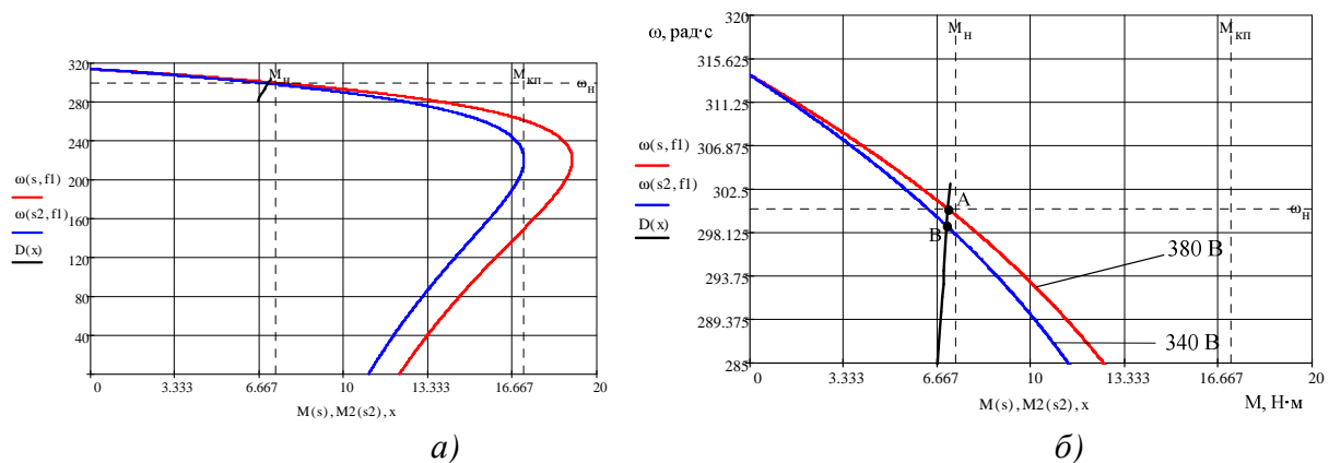
Рисунок – 3 Механічні характеристики АД та водяного насоса: а) загальний вигляд, б) фрагмент в зоні навантаження
