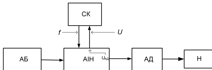
Рисунок – 5 Структурна схема керованого живлення асинхронного двигуна
