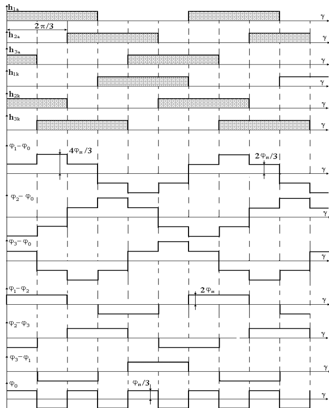
Рисунок 1 – Діаграма роботи вентилів АИН та криві напруг
