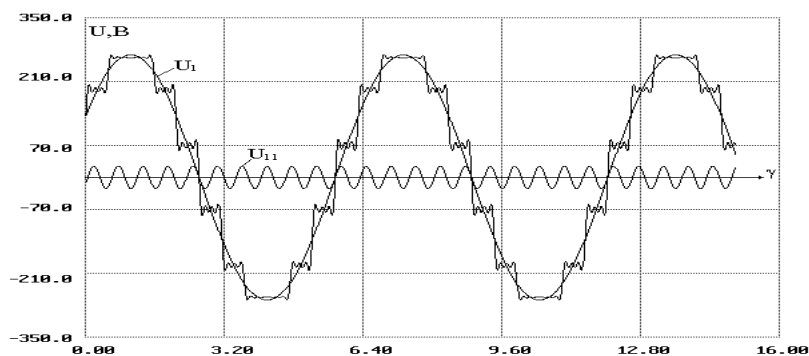
Рисунок 6 – Залежності напруги і 1-ї та 11-ї гармонік (К2АІН-АД)
