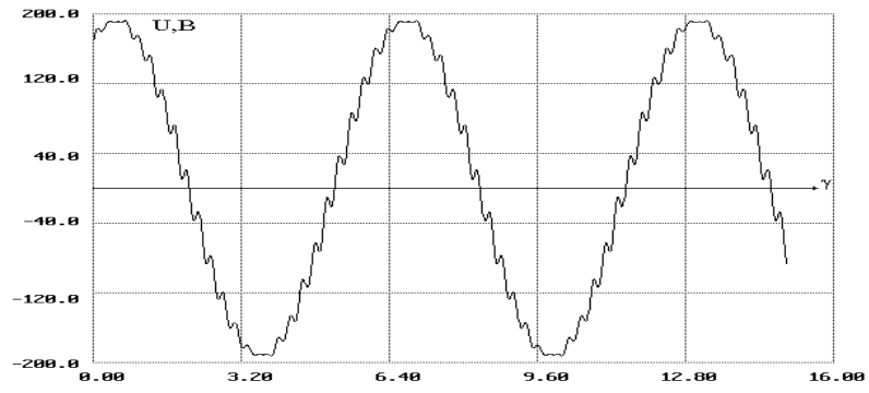
Рисунок 7 – Залежність фазної напруги (К:2К2АІН-АД)
