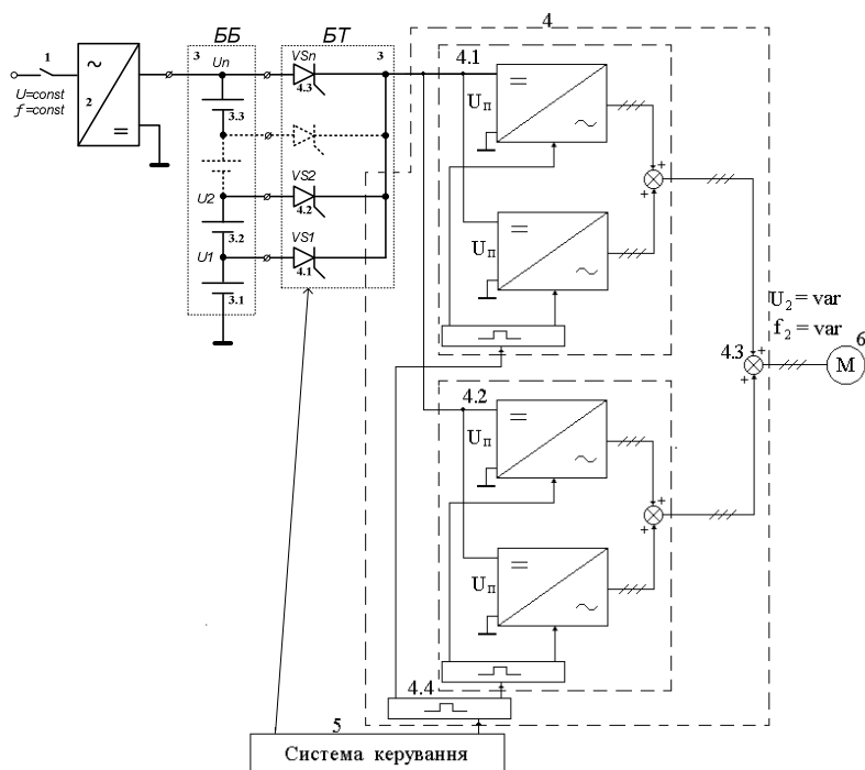
Рисунок 3 – Блок-схема електропривода з КІН (К:2К2АИ-АД)
