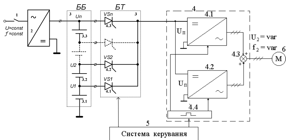
Рисунок 2 – Блок-схема електропривода з КИП (K2AИН-АД)
