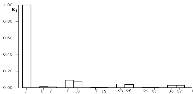
Рисунок 9 – Гістограма гармонічного складу напруги (К2АІН, Y/Y-Y/Y)
