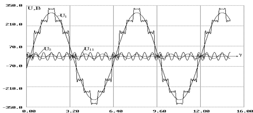
Рисунок 5 – Залежності напруги і 1-ї, 5-ї та 11-ї гармонік (К2АІН-АД, Y/Y-Y/Y)
