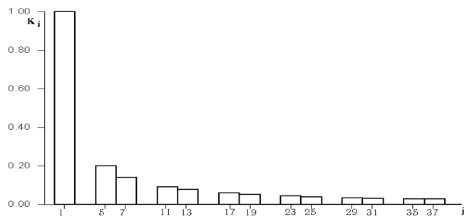
Рисунок 8 – Гістограма гармонічного складу напруги (АІН)
