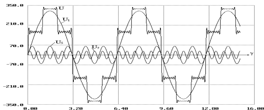
Рисунок 4 – Залежності напруги і 1-ї, 5-ї та 7-ї гармонік (АІН)
