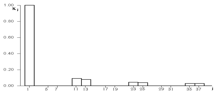
Рисунок 10 – Гістограма гармонічного складу напруги (К2АІН)
