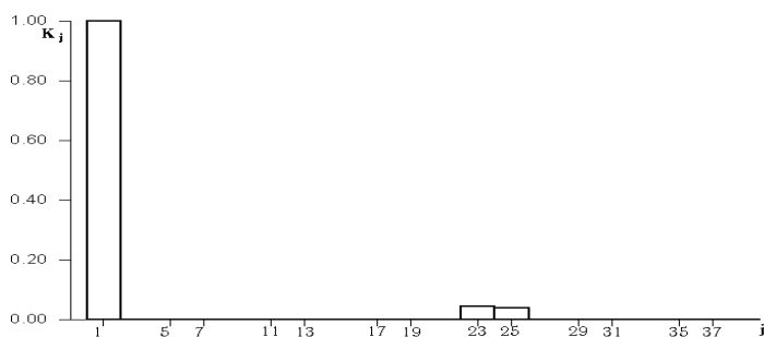
Рисунок 11 – Гістограма гармонічного складу напруги (K:2K2A1H)
