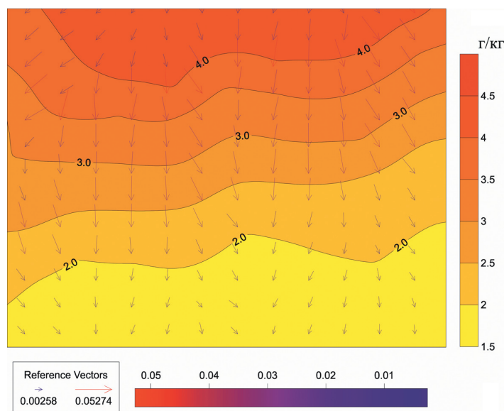
Рисунок. Розподіл умісту нафтопродуктів у пробах ґрунтів з дослідженої ділянки (кольором та ізолініями позначено концентрацію нафтопродуктів, стрілками – градієнт концентрації, більша довжина стрілки відповідає більшому градієнту)
