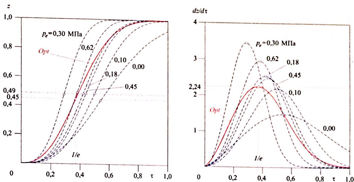
Рис. 2. Порівняння гіпотетично оптимальної діаграми теплотворення з тими, що апроксимують реальні
