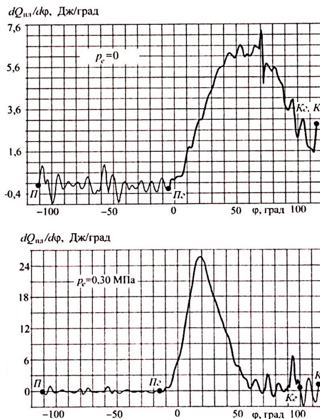
Рис. 1. Приклади діаграм теплотворення в бензиновому двигуні внутрішнього згоряння
