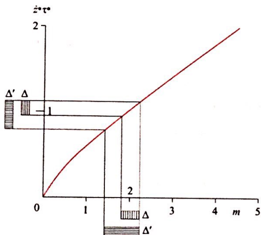
Рис. 3. Взаємозв'язок між визначальними параметрами процесів теплотворення
