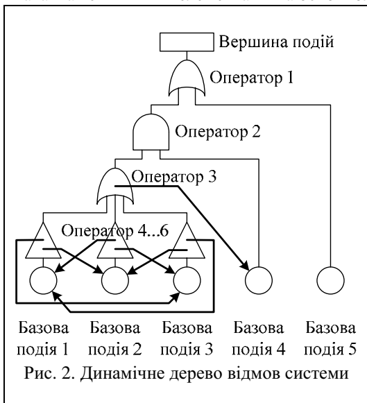
Рис. 2. Динамічне дерево відмов системи
