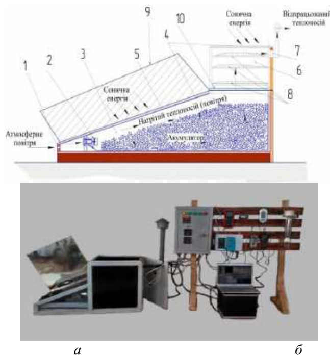
Рис. Геліосушарка з тепловим акумулятором та плоским дзеркальним концентратором: а – конструктивно-технологічна схема; б – загальний вигляд; 1 – вхідний канал; 2 – вентилятор з нагрівачем; 3 – повітропровід; 4 – повітряний колектор; 5 – теплоакумуючий матеріал (на основі гальки); 6 – сушильна камера; 7 – витяжний канал; 8 – решета; 9 – плоский дзеркальний концентратор; 10 – заслінка.
