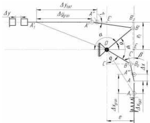
Рис. 2. Кінематична схема дезаксіального кривошипно-шатунного механізму переміщення контактів вимикача.
