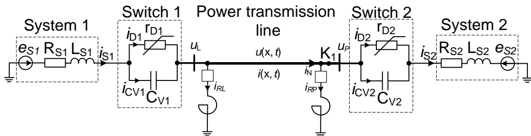
Рис. 1. Розрахункова схема досліджуваного фрагмента електричної мережі.
