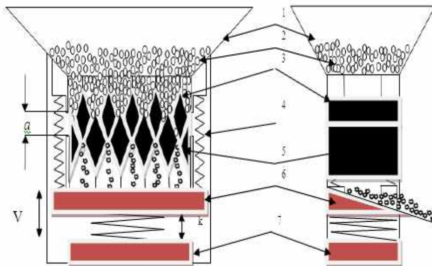
Рис. Зернова дробарка з електромагнітним віброзбудником: 1 – бункер; 2 – зерно; 3 – пасивні рифи; 4 – пружини; 5 – активні рифи; 6 – вібралоток; 7 – електромагнітний вібратор.
