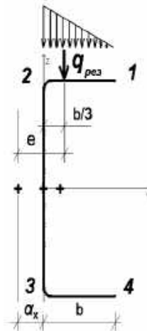
Рис. 1. Схема прикладеного навантаження.
