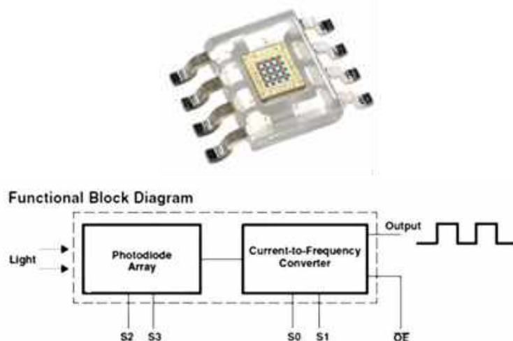
Рис. 2. Давач колірної температури та освітленості TCS3200 і принцип роботи давача освітленості.
