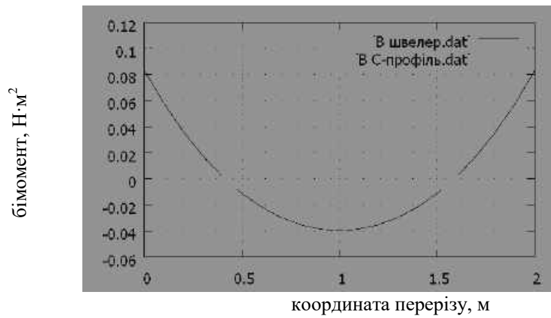
Рис. 2. Епюра бімоментів.
