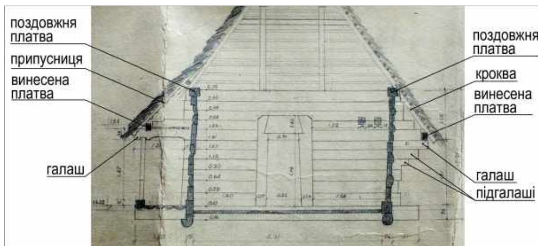
Рис. Пояснення до фрагмента розрізу житлового будинку 1792 р. зі села Орявчика.
