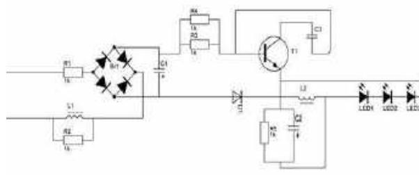
Рис. 4. Будова та електрична схема джерела світла «Osram».
