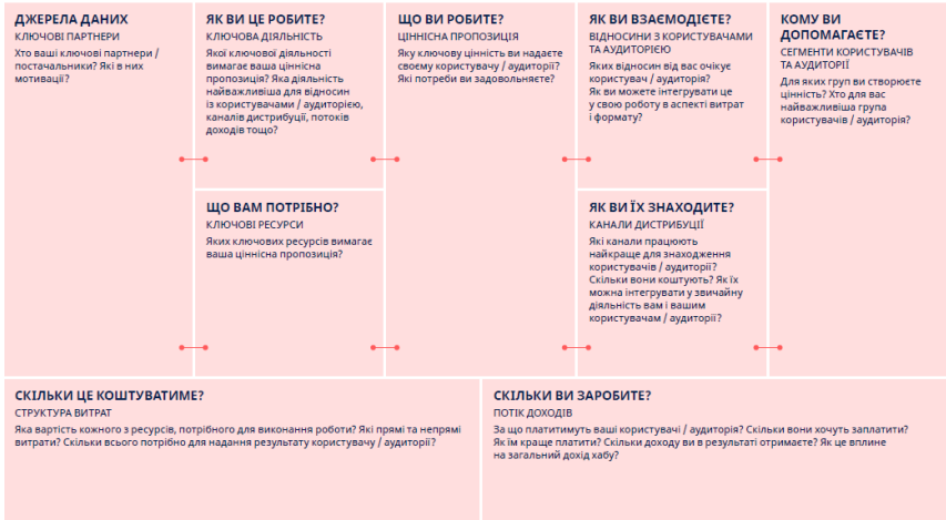
Рисунок 1. Канва бізнес-моделі
