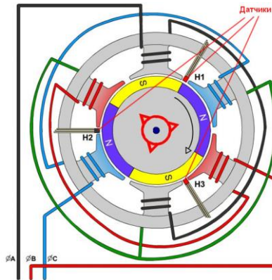
Рисунок 2 – Схема трифазного безколекторного двигуна постійного струму
