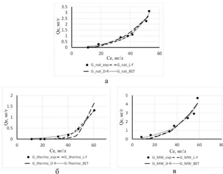
Продовження рисунка 1 – Ізотерми адсорбції \text{PO}_4^{3-} (а - вихідний зразок, б – прожарений 550 °С, в – мікрохвильове опроміннення)
