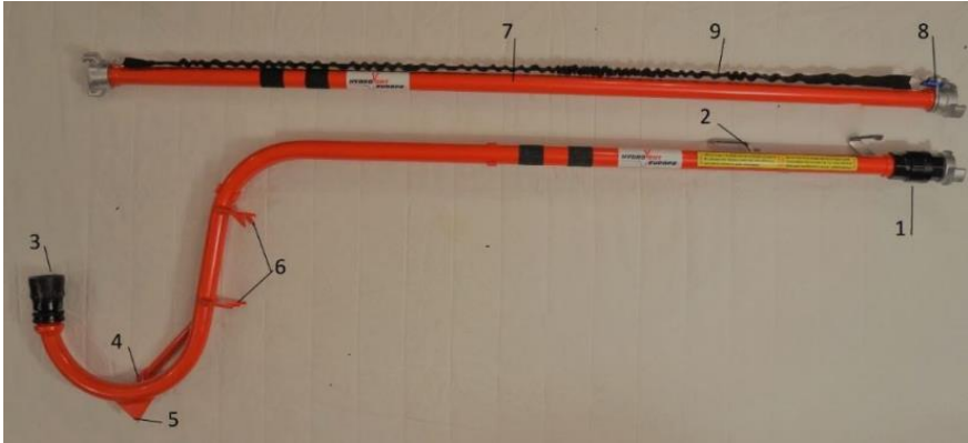
Рисунок 1 – Будова VT: 1. Засувка; 2. Вогнегасна засувка; 3. Вентиляційна насадка; 4. Вогнегасна насадка; 5. Скобійник; 6. Тримач; 7. Подовжувальна труба; 8. Замок; 9. Ролетний ремінь.
