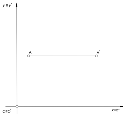
Рисунок 4 – Зсув точки пропорційно координаті y
