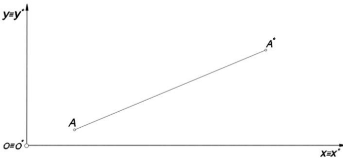
Рисунок 2 – Зміна масштабу на осях Ox та Oy
