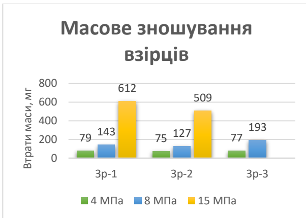
Рисунок 1 – Втрати маси зрізів при навантаженнях 4, 8, 15 МПа
