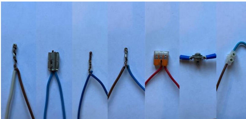
Рисуюнок 1 – Способи з'єднання контактів кабельних виробів, що досліджувалися
