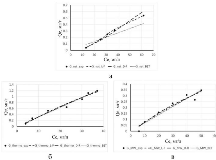
Рисунок 1 – Ізотерми адсорбції \text{NH}_4^+ (а - вихідний зразок, б – прожарений 550 °С, в – мікрохвильове опроміннення)
