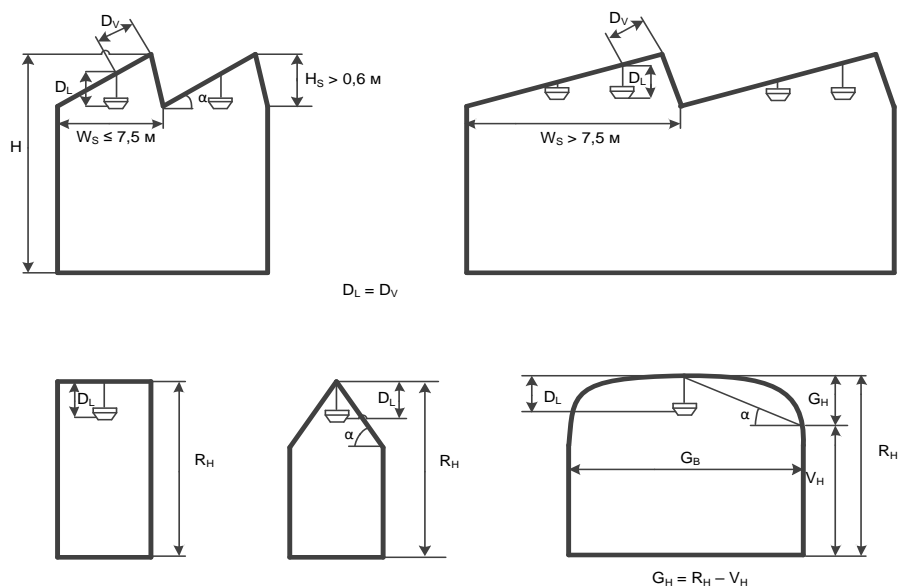
Рисунок 2 – Розміщення і розташування точкових димових пожежних сповіщувачів за різних форм стель і покриттів
