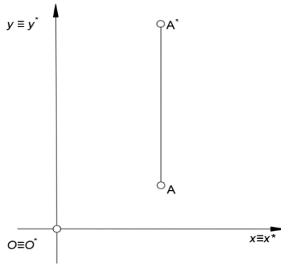
Рисунок 3 – Зсув точки пропорційно координаті x
