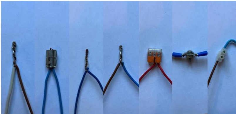
Рисуюнок 1 – Способи з'єднання контактів кабельних виробів, що досліджувалися
