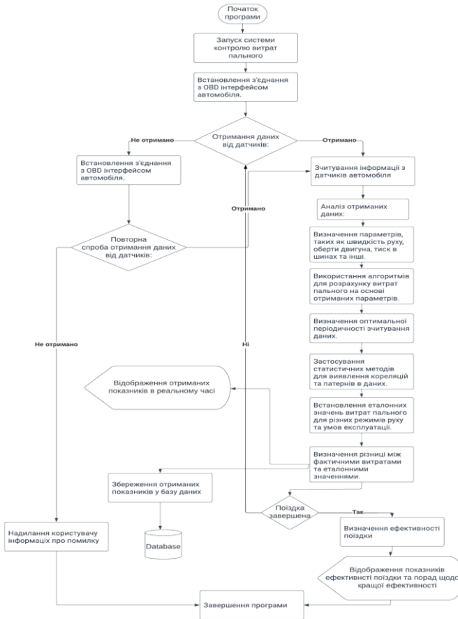
Рисunek 1 – Алгоритм зниження витрат пального
