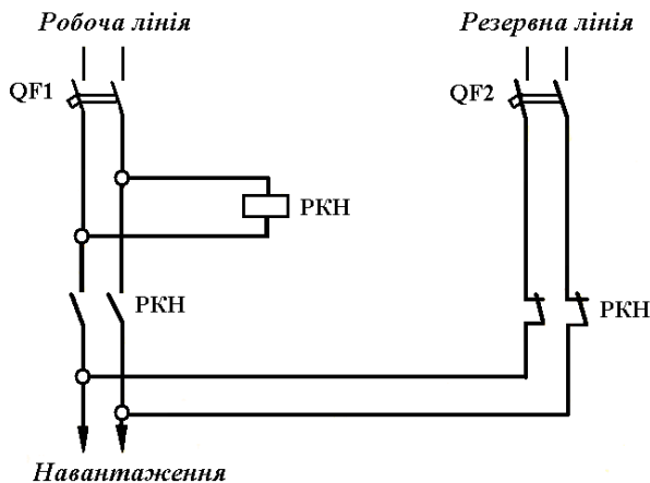
Рисунок 2 – Схема АУР в двопрото-віднікових мережах до 220В.
