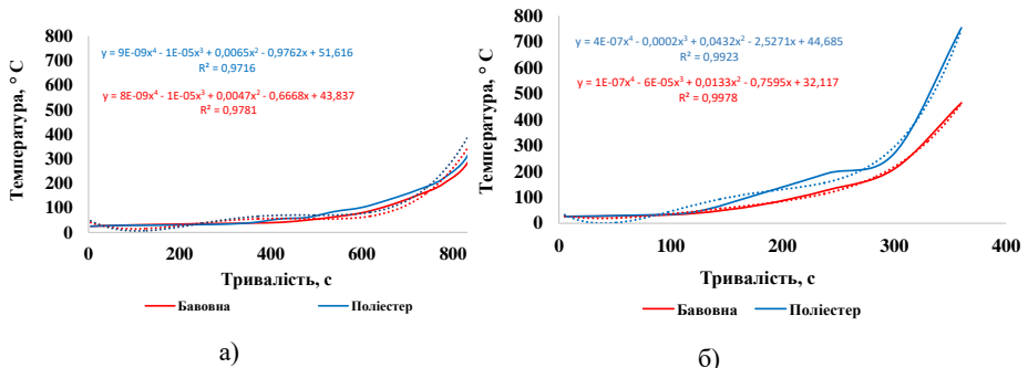
Рисунок 2 – Залежності температур від часу нагрівання ділянок з
