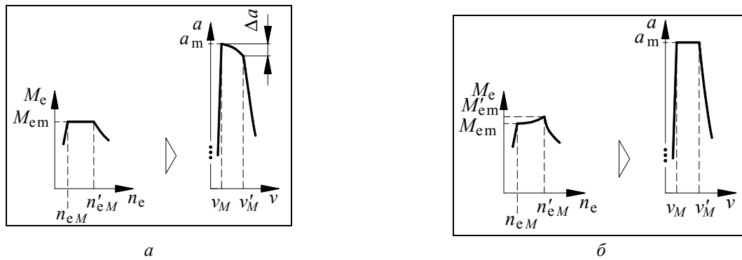
Рис. 6. Варіанти характеристик пришивидження автомобіля
