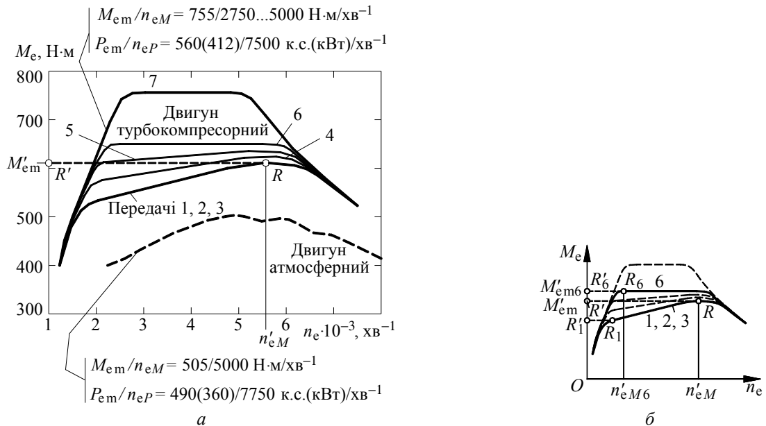
Рис. 8. Граничні швидкісні характеристики восьмициліндрових У-подібних бензинових з безпосереднім впорскуванням двигунів автомобілів штибу купе-кабриолет Ferrari California (двигун — атмосферний) та Ferrari California T (двигун — бітурбокомпресорний з турбінами штибу twin scroll (здовоєний равлик))
