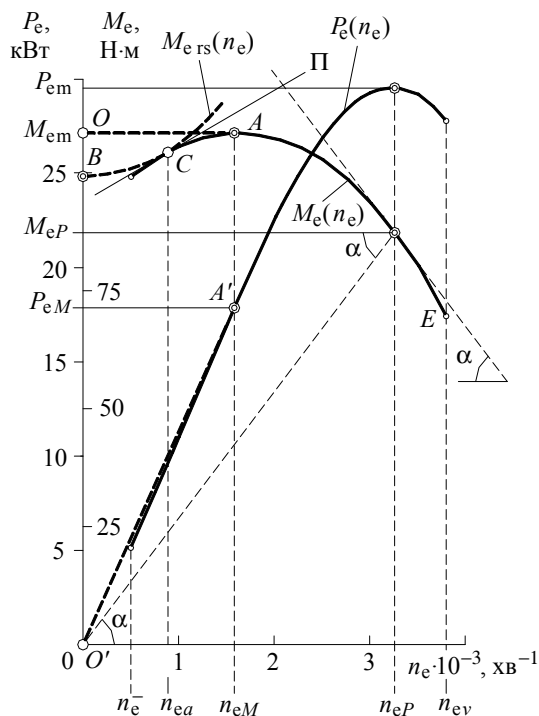
Рис. 1. Гранична швидкісна характеристика (радіше, її фрагмент, що охоплює залежність від частоти обертання вала лише потужності й моменту)
