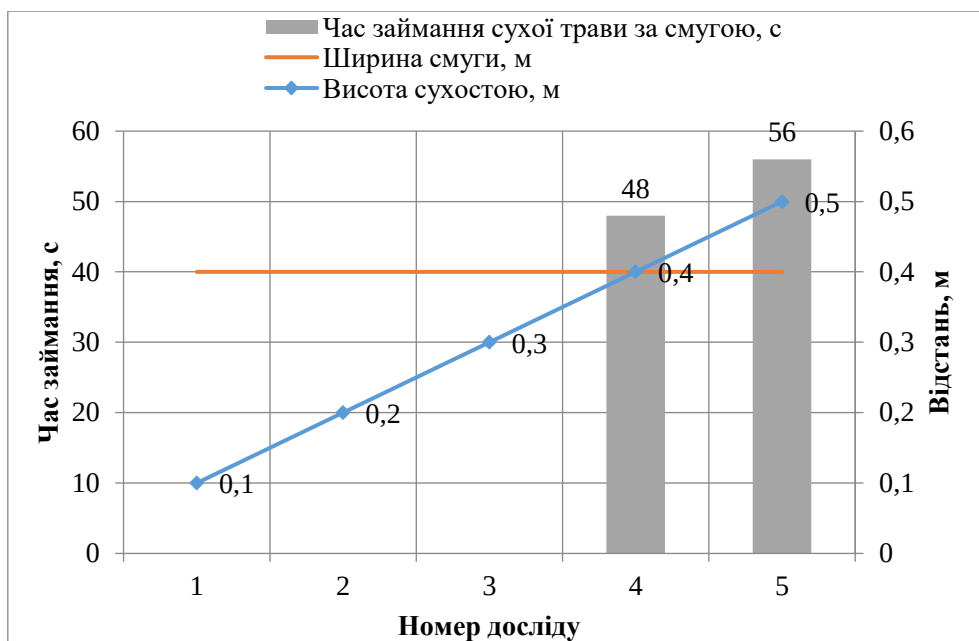
Рисунок 5. Час займання сухої лучної рослинності при ширині мінералізованої смуги 0,4 м
