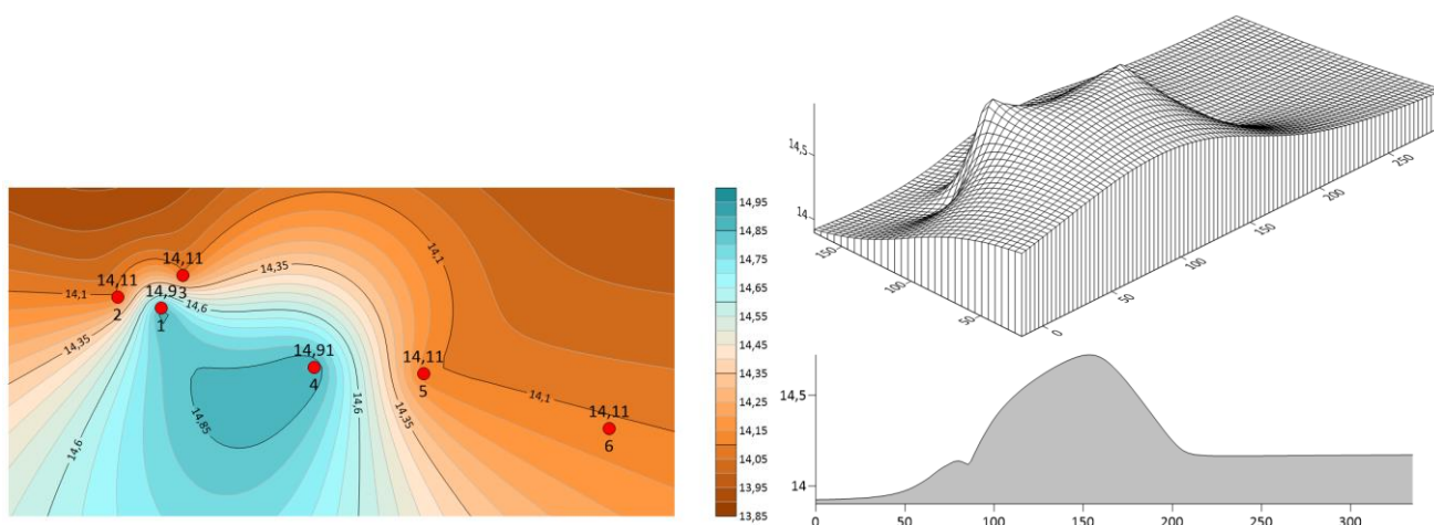
Рисунок 27. Моделювання поширення Ра у горизонті >15 см у межах впливу сміттєзвалища
