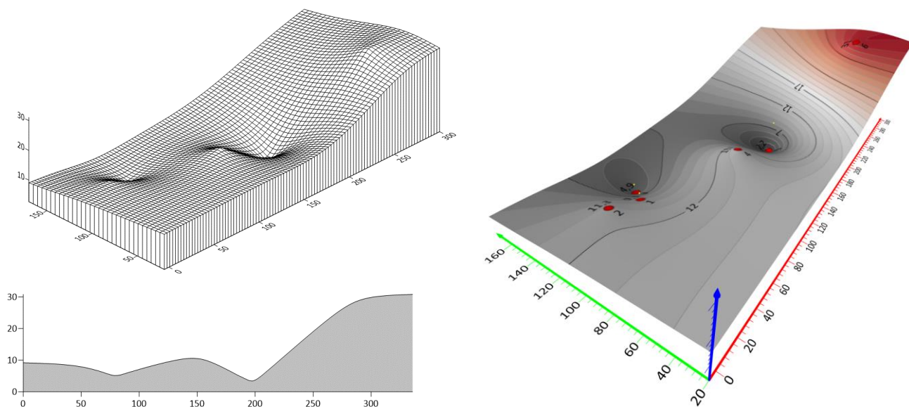
Рисунок 12. Моделювання поширення Zn у горизонті 5-15 см у межах впливу сміттєзвалища
