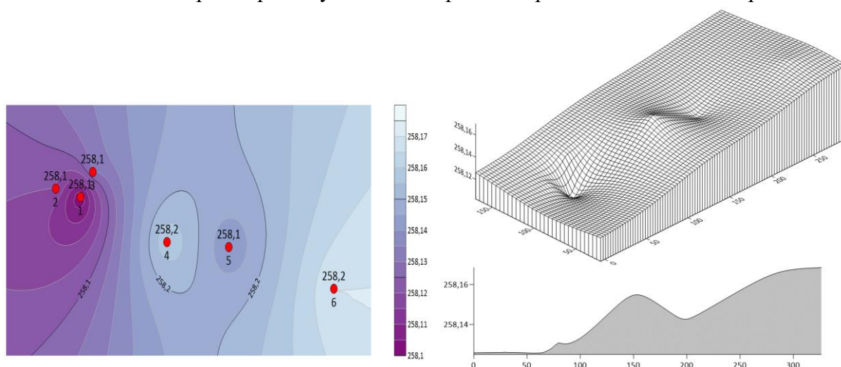
Рисунок 24. Моделювання поширення К у горизонті 5-15 см у межах впливу сміттєзвалища
