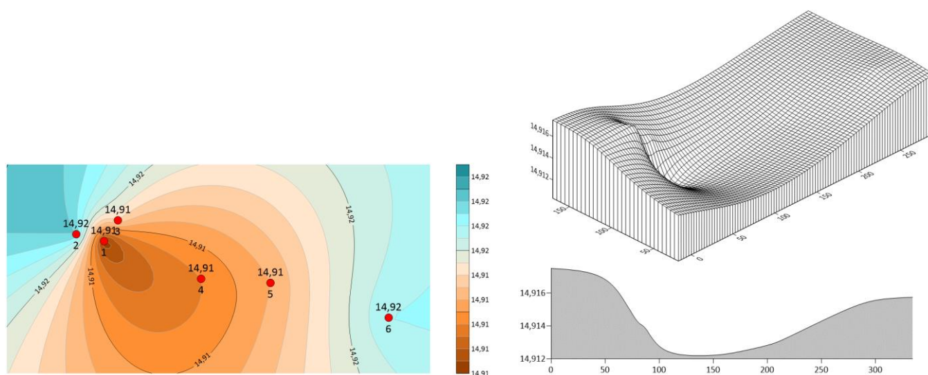
Рисунок 26. Моделювання поширення Ра у горизонті 5-15 см у межах впливу сміттєзвалища
