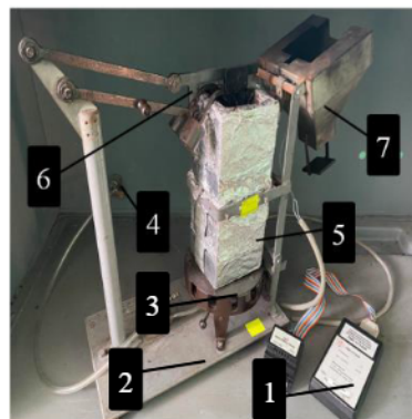
Рис. 2. Зовнішній вигляд установка для визначення вогнезахисної ефективності покриттів і просочень: 1 – ПВІ-111АК Перетворювач вимірний інтелектуальний з блоком комутації та носієм інформації мікро SD; 2 – металева підставка; 3 – газовий пальник; 4 – пристрій для регулювання подачі газу; 5 – керамічний короб; 6 – тримач зразка що випробується; 7 – зонт із термопарою
