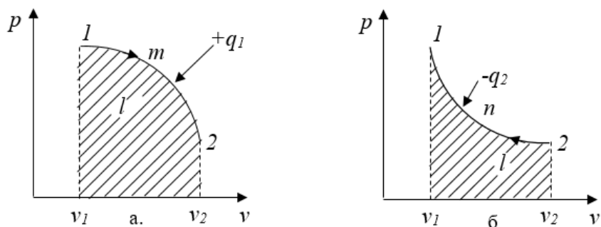
Рис. 1.9. Схема елементів циклу
