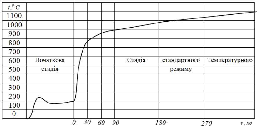
Рис. 2.17. Температурний режим в житлових і громадських спорудах
