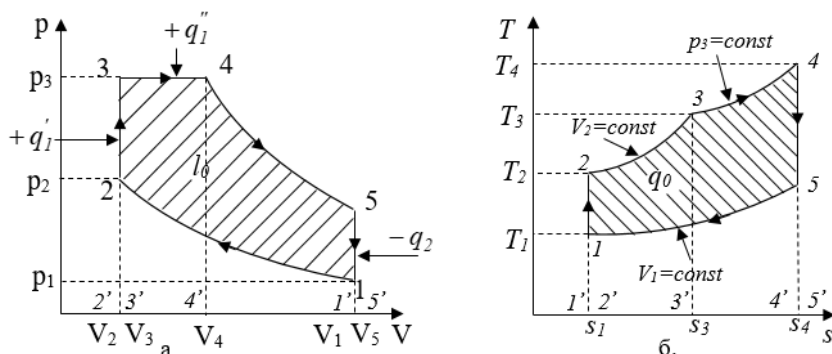
Рис. 1.15. Схема циклу із змішаним підведенням теплоти
