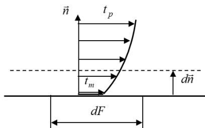
Рис. 2.9. Розподіл температурного поля в околі поверхні тіла
