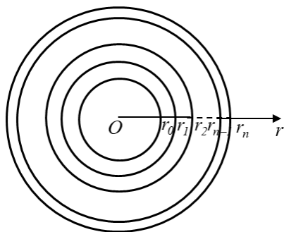
Рис. 2.8. Схема багатошарової сферичної стінки
