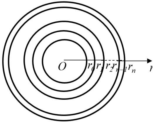
Рис. 2.7. Багатошарова циліндрична стінка
