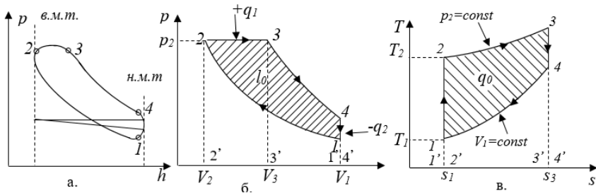
Рис. 1.14. Схема циклу з підведенням теплоти при сталому тиск
