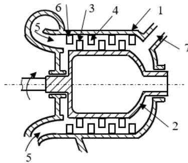
Рис. 1.18. Схема осьового компресора
