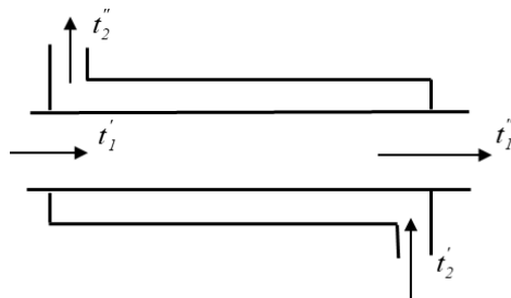
Рис. 2.20. Схеми теплообмінника "труба в трубі"
