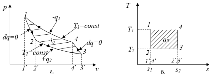
Рис. 1.11. Схема прямого циклу С. Карно
