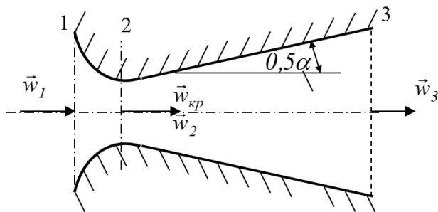
Рис. 1.22. Схема сопла Лаваля
