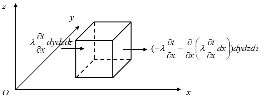
Рис. 2.1. Схема теплового потоку вздовж осі Ox
