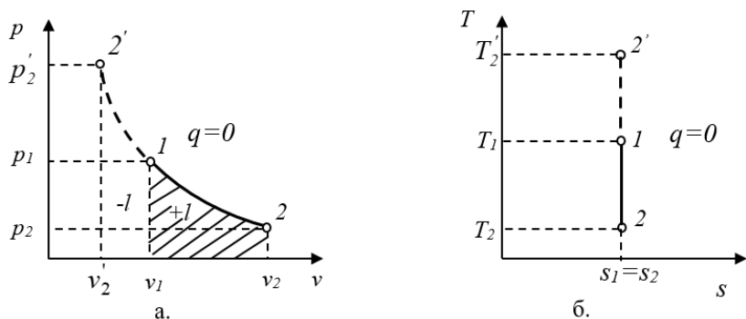
Рис. 1.8. Зображення адиабатного процесу в p, v та T, s координатах
