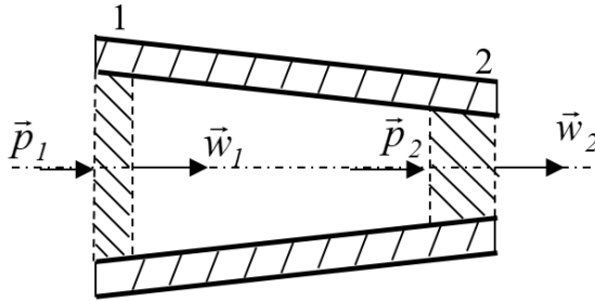
Рис. 1.20. Схематичне зображення циліндричного каналу
