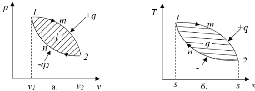
Рис. 1.10. Схема кругового циклу
