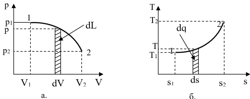
Рис. 1.4. Схематичне зображення виконаної роботи і підведеної теплоти
