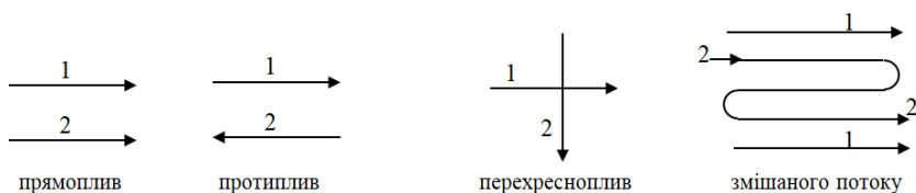
Рис. 2.19. Схеми руху теплоносіїв в теплообмінних апаратах
