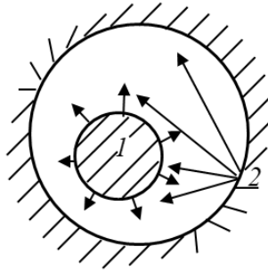
Рис. 2.13. Схема променевого теплообміну між тілом 1 і внутрішньою поверхнею тіла 2
