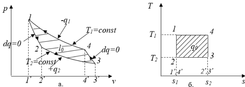
Рис. 1.12. Схема оберненого циклу С. Карно
