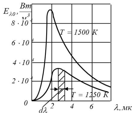
Рис. 2.11. Залежність спектральної інтенсивності випромінювання абсолютно чорного тіла від довжини хвилі і температури
