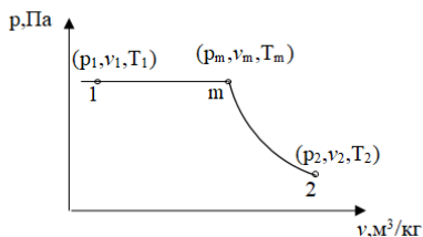
Рис. 1.2. Динаміка зміни термодинамічного стану робочого тіла
