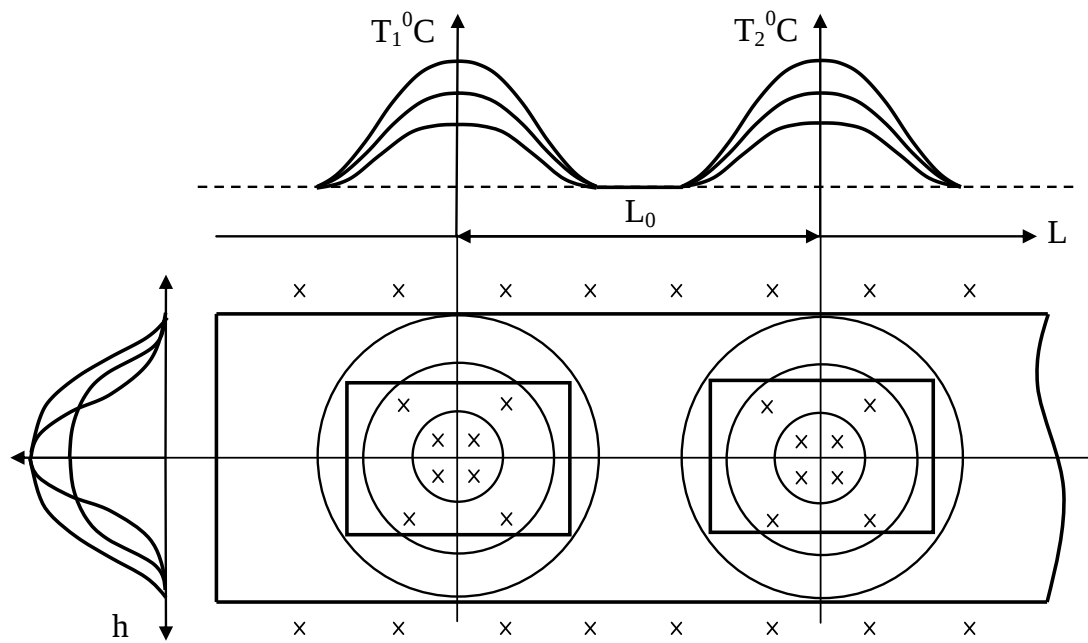
Рисунок 1 – Розподіл теплового поля від лампових випромінювачів на поверхні книжкових блоків
