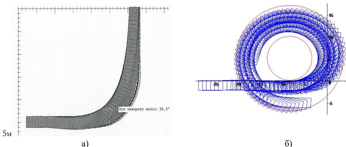
Рисунок 3 - Габаритна смуга руху автопоїзда при повороті на 90^{\circ} (а) і коловому русі (б)
