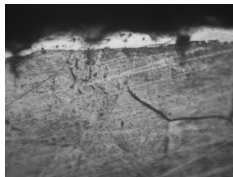
Рисунок 2 – Типові мікроструктури зміцненого поверхневого шару шипа зі сталі 45, отримані за використання як анод твёрдих сплавів ВК8 (а) та Т15К6 (б) (x500).
