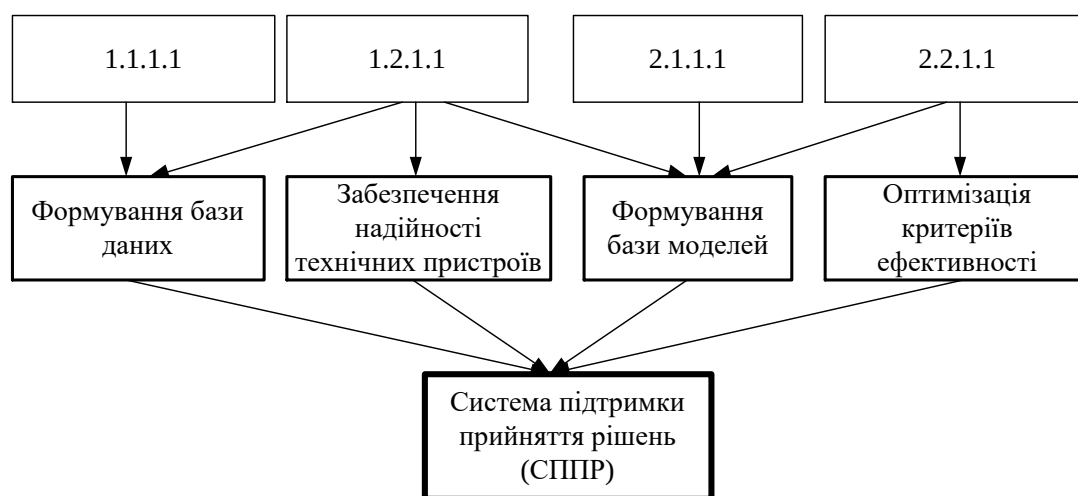
Рисунок 3 – Структура системи підтримки прийняття рішень
