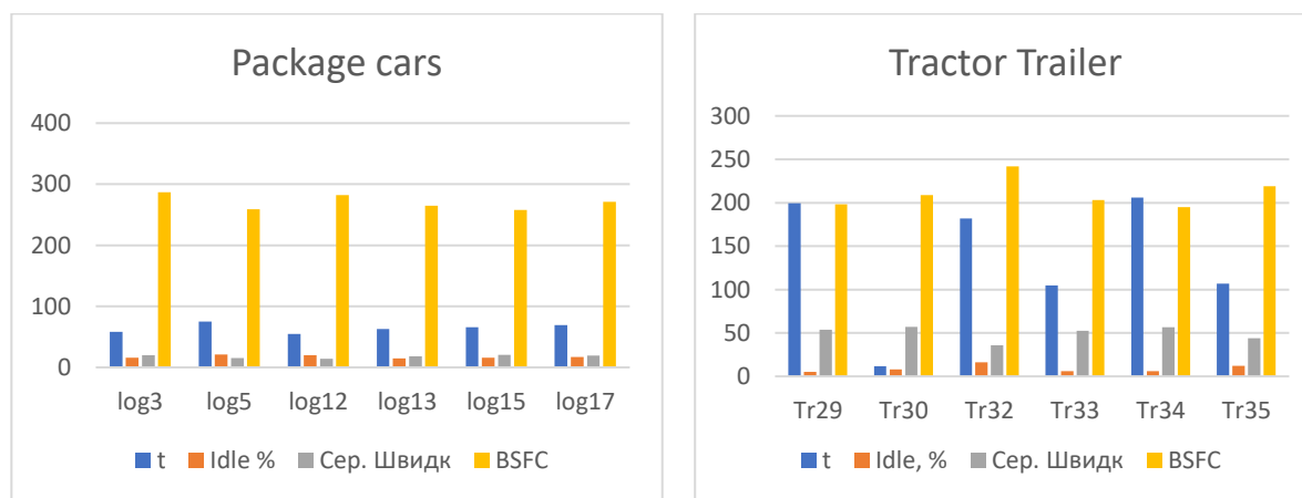
Рисунок 1 – Порівняння показників для шести автомобілів «Package car» та «Tractor trailers», що працюють на відновному дизельному паливі (t- час поїздки [год], idle - час простою [%], середня швидкість [миль/год], BSFC- питома витрата палива [г/кВт год])
