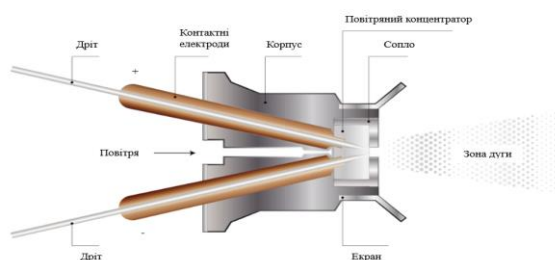
Рис. 3. Електродугове напилення
