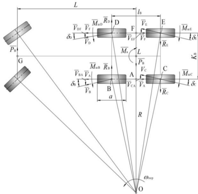
Рисунок 1 – Схема для визначення особливостей руху коліс візка триосового автомобіля по криволінійній траєкторії
