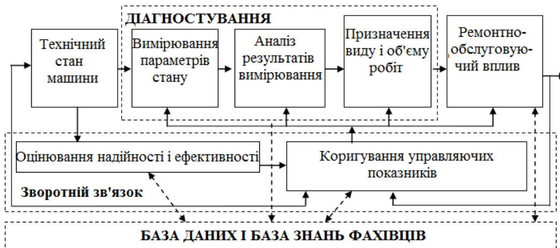
Рисунок 2 – Схема управління технічним станом вантажних автомобілів
