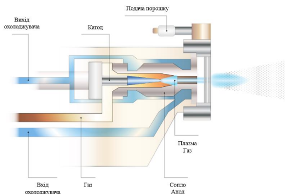
Рис. 4. Плазмове напилення
