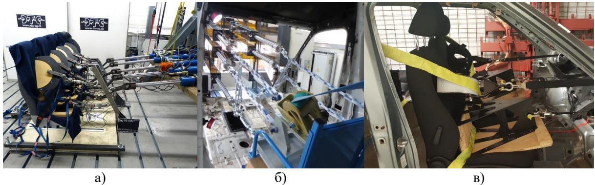
Рисунок 1 – Випробувальні стенди пасків безпеки: а) з інтегрованими пасками згідно R14/R16; б) анкери безпосередньо у кузові; в) прикладання сили для імітації умов аварійного навантаження на анкерні точки
