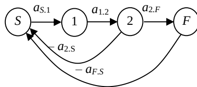
Рисунок 1 – Графічне моделювання обмежень на тривалість операцій: S, F – фіктивні операції, які представляють формальний початок і кінець процесу
