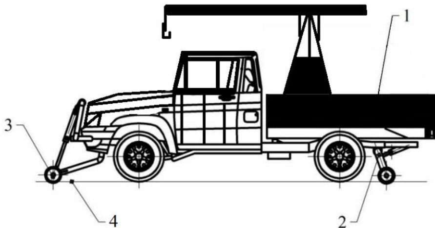
1 – автомобіль; 2, 3 – заднє та переднє залізничне шасі; 4 – поверхня катання рейок
