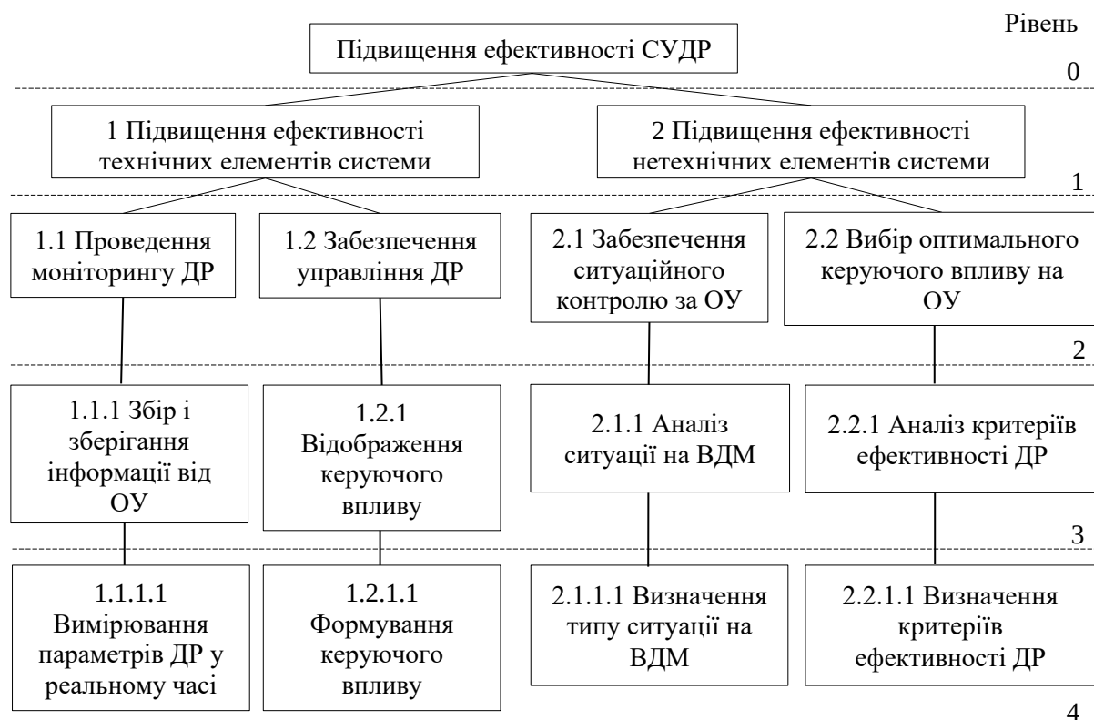
Рисунок 2 – Дерево цілей СУДР
