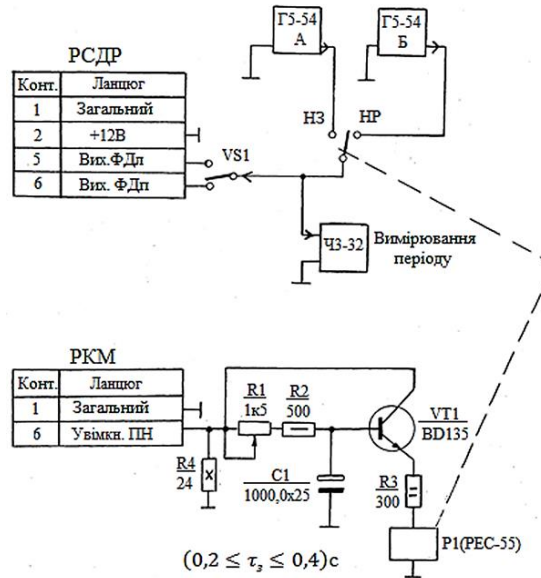
Рисунок 2 – Схема метрологічного контролю каналу ПС [2]
