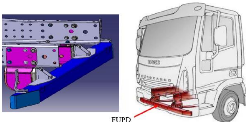
Рисунок 1. Ліворуч – 3D-зображення досліджуваного пристрою; праворуч – розташування FUPD на промисловому транспортному засобі [4].
