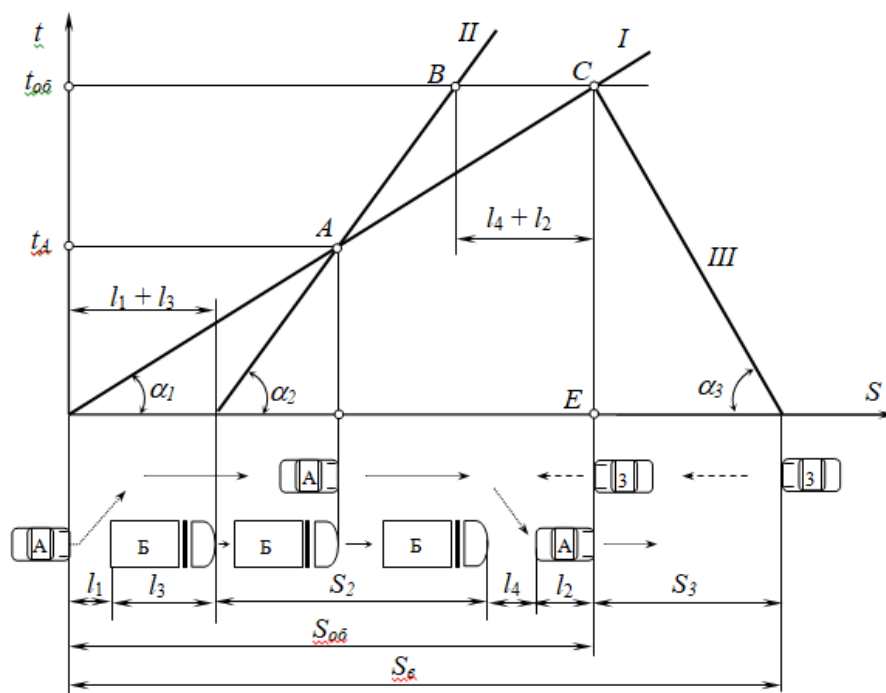
Рисунок 2 – Характеристика обгону під час рівномірного руху
