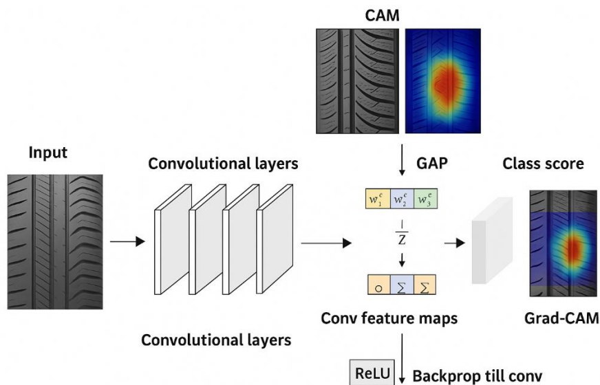
Рисунок 3 – Візуалізація результатів роботи моделі CNN (Grad-CAM)
