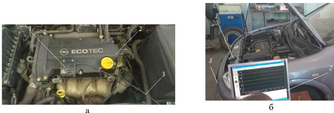
Рисунок 1 – Розміщення багатодатчикового модуля Steval-mki062v1 при діагностиці вібрацій системи «двигун Z14XEP – кузов автомобіля Opel Astra G»: а – двигун: 1 – багатодатчиковий модуль; 2 – кришка головки блоку циліндрів; 3 – провід USB; б – моторний відсік: 1 – багатодатчиковий модуль; 2 – монітор; 3 – провід USB
