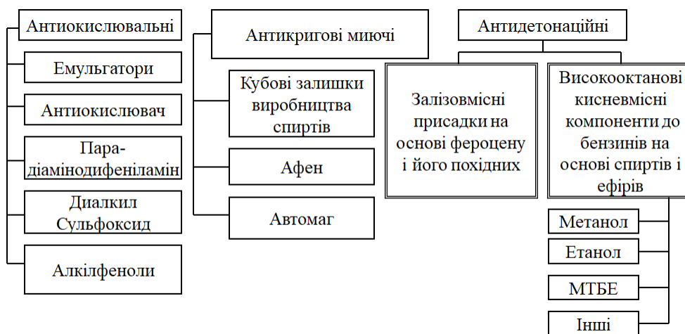
Рисунок 1 – Класифікація присадок до бензинових палив
