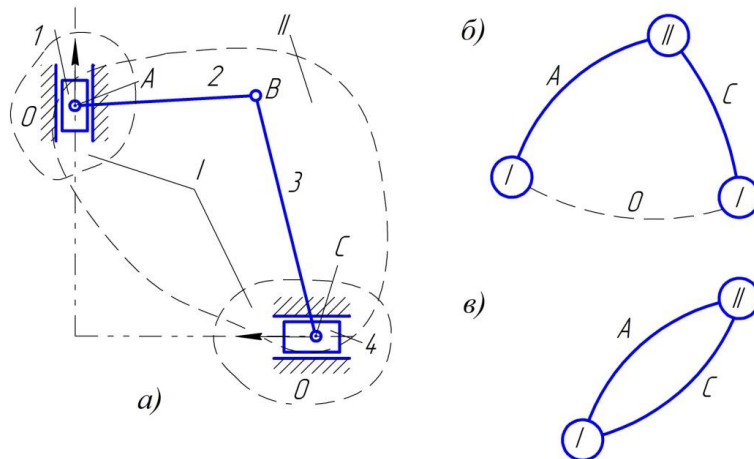
Рис.1. Двопозунковий механізм з двома механізмами I класу та його можливі графи
