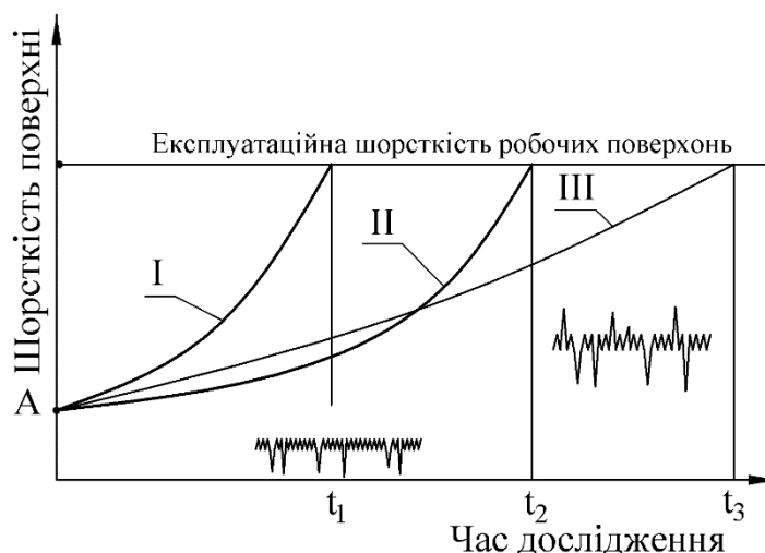
Рисунок 4 - Характери виходу трибоспряження на експлуатаційну шорсткість досліджуваного зразка
