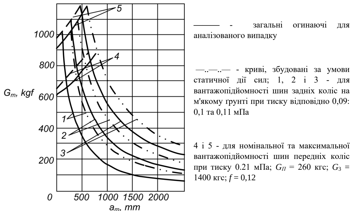
Рисунок 2 – Характеристика вантажопідйомності ТСШ Т-16МГ на транспортних роботах (для статичних та динамічних умов)
