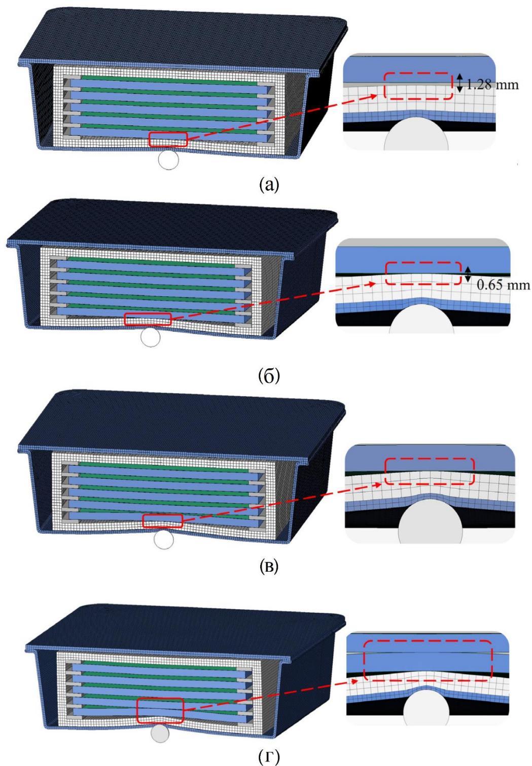
Рисунок 1 – Деформація корпусу батарей при різних швидкості удару: (а) 10 м/с, (б) 15 м/с, (в) 20 м/с та (г) 25 м/с
