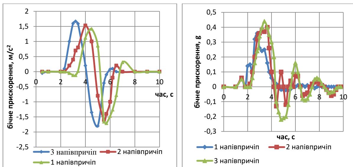
Рисунок 3 - Зміни бічного прискорення напівпричепів при виконанні типових маневрів «вхід в поворот» (а) і «переставка» (б) за швидкості автопоїзда 10 м/с
