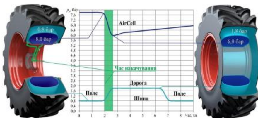
Рис. 1 Система AirCell від компанії Mitas
