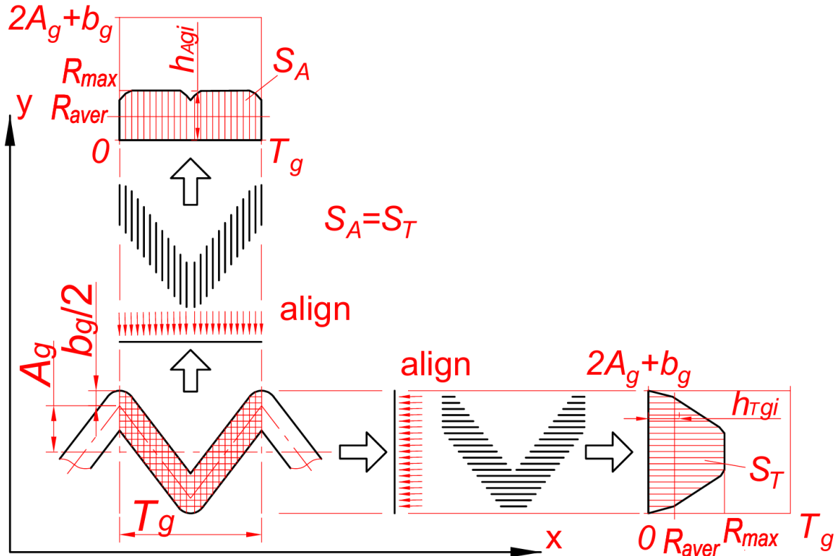
Рисунок 1 – Схема побудови графіків осьової та міжосьової площинної неоднорідності форм канавок мікрорельєфів
