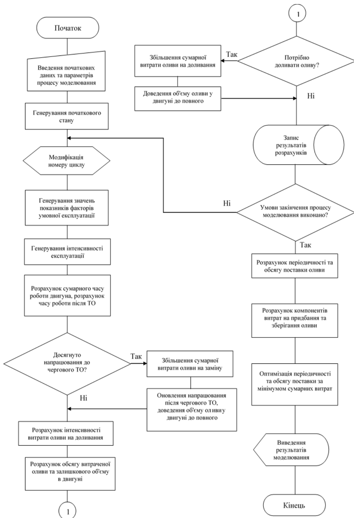
Рисунок 1 - Укрупнений алгоритм імітаційної моделі формування витрати моторної оливи при експлуатації автомобілів
