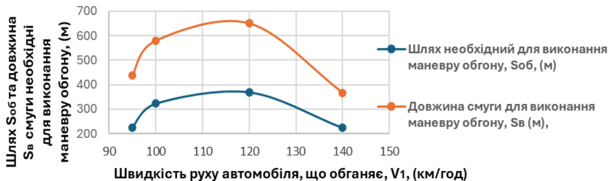
Рисунок 3 – Залежності шляху обгону S_{об} та довжини смуги S_е від швидкості руху V_1
