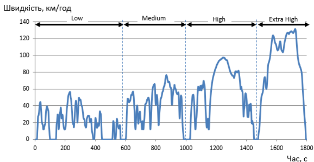
Рисунок 2 – Їздовий цикл Цикл WLTP ( Worldwide Harmonised Light Vehicles Test Procedure )
