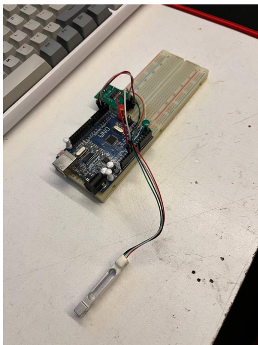
Рисунок 3 - Тензодатчик з мікросхемою
