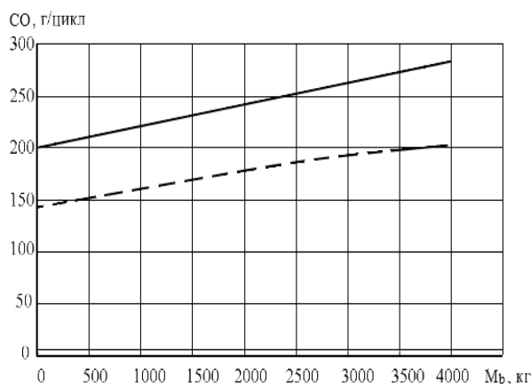
Рисунок 2 - Залежність масових викидів шкідливих речовин за цикл, приведених до CO від завантаження при роботі двигуна за дизельним і газодизельним циклами.
