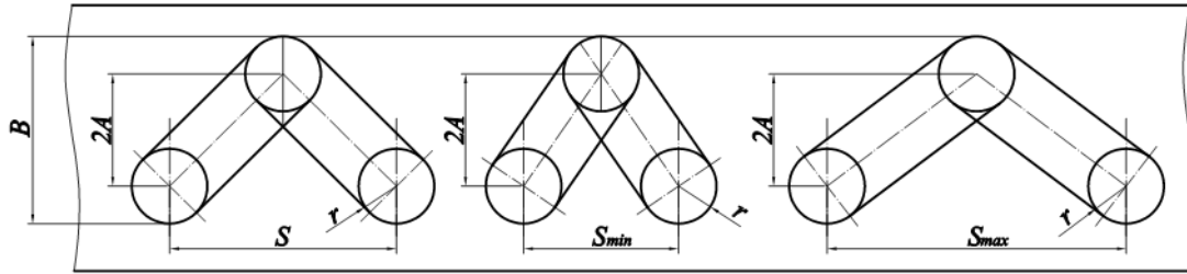
Рисунок 1 – Схема для визначення площ поверхонь із канавками мікрорельєфу
