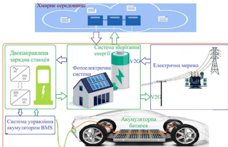
Рисунок 1 – Приклад використання Інтернету транспортних засобів при підключенні електромобіля до зарядної станції та до електричної мережі за технологією V2G
