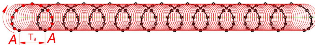
Рисунок 1 – Траєкторія руху деформувального елемента інструменту при обертання його навколо власної осі
