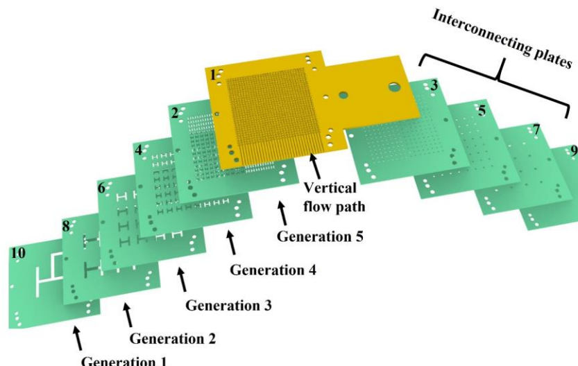
Рисунок 2 - Схематичний контур і порядок 2D плоских пластин друкованих плат (поколінь і з'єднувальних пластин), використаних для розробки 5-поколінної катодної фрактальної пластини з поточним полем. Пластина 1: з золотим покриттям; пластини 2 – 10: звичайні друковані плати.
