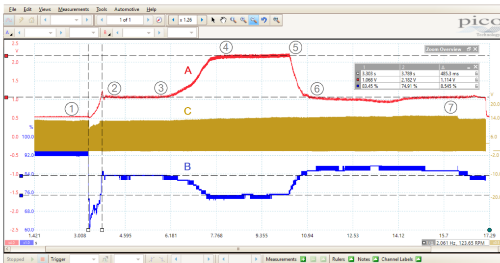
Рисунок 2 – Осцилограма перевірки продуктивності паливної системи Common Rail
