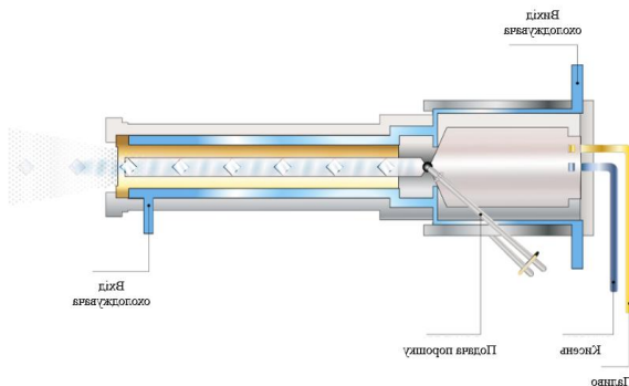
Рис. 5. Вискошвидкісне газополуменеве напilenня
