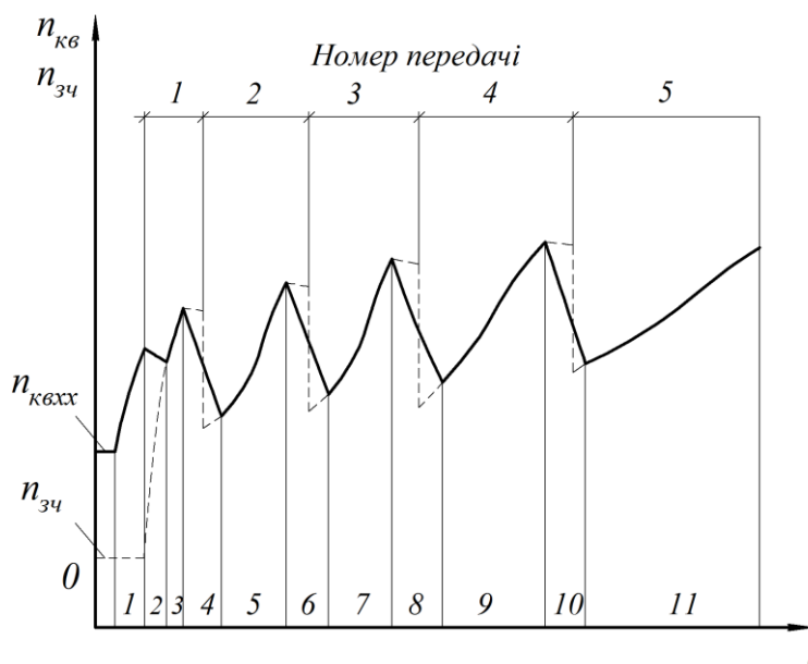
Рисунок 1 – Процес розгону автомобіля з місця з перемиканням передач від нижчої до вищої
