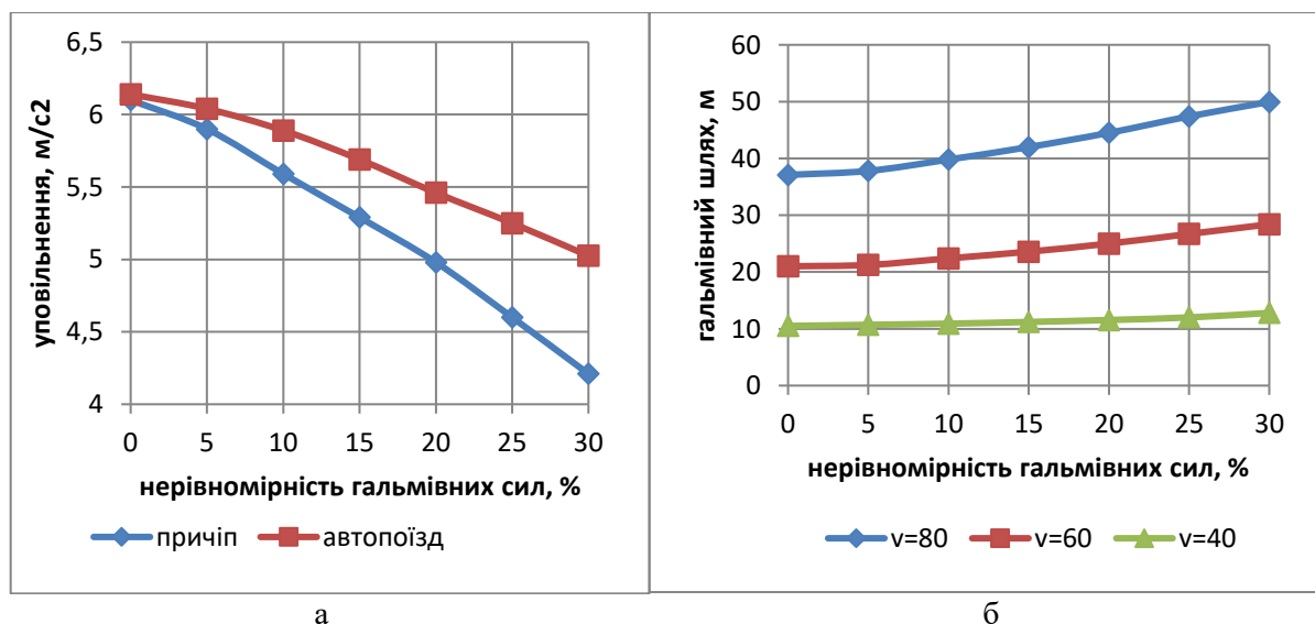
Рисунок 1 – Уповільнення (а) і шлях гальмування автопоїзда (б) в залежності від нерівномірності гальмівних сил на здвоєній осі причепа
