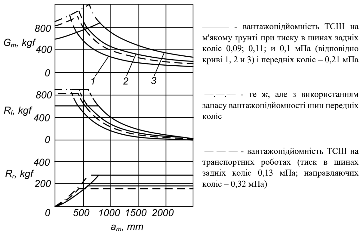
Рисунок 1 – Характеристика потенційної вантажопідйомності ТСШ Т-16МГ
