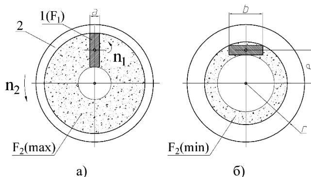
Рисунок 2 - Схема контакту трибоспряження та характер зміни K_{вп}
