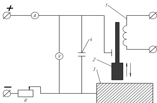
Рисунок 1 – Принципова схема електроіскрової установки “Элитрон -24А”:
