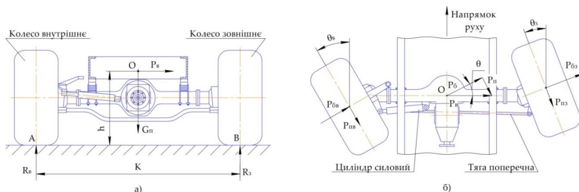
Рисунок 2 – Схема кінематики та динаміки керованих коліс під час руху ліворуч по криволінійній траєкторії
