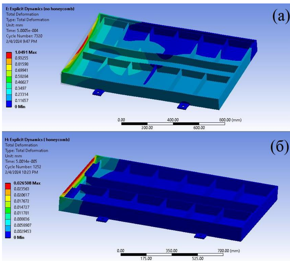
Рисунок 2. Порівняння деформації корпусів без стільникової структури (а) і з використанням стільникової структури (б) [3].
