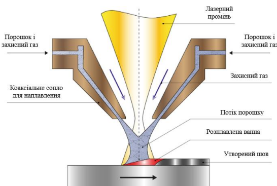
Рис. 7. Лазерне напилення
