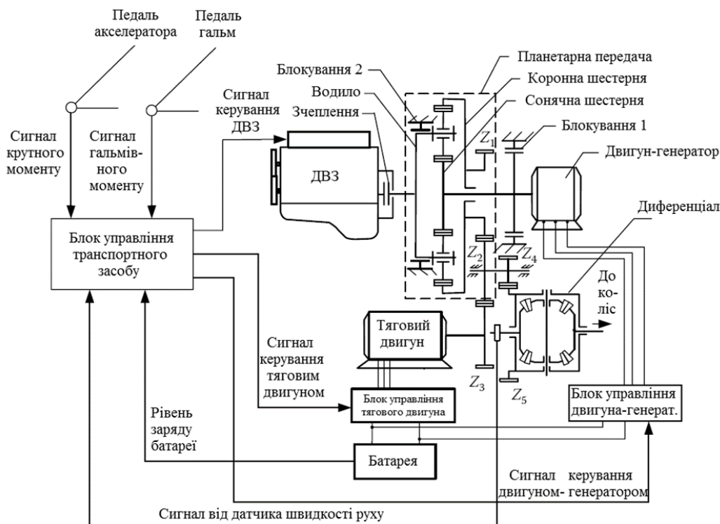
Рисунок 1 – Загальна схема конструкції гібридної силової установки з тягово-швидкісним зв'язком (комбінована)
