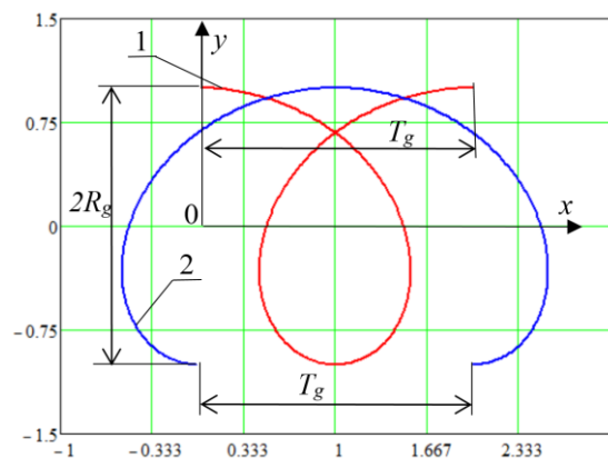
Рисунок 2 – Траєкторія руху деформувальних елементів при формуванні частково регулярних мікрорельєфів ротаційного виду на плоских поверхнях
