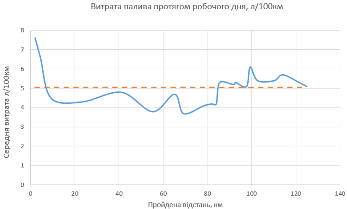
Рисунок 2 - Графік зміни середньої витрати палива на маршруті
