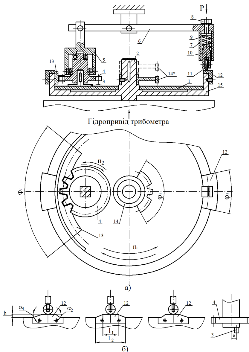
Рисунок 1 - Схема вузла тертя та механізм навантаження трибометра (а), варіанти виконання сегментів 12 та розміщення зразка 3 відносно зразкотримача 4 (б), \alpha_1 , \alpha_2 – кути підйому та сходження сегмента 12, h – висота підйому сегмента
