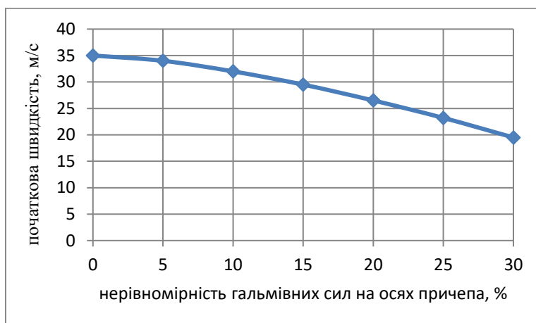
Рисунок 3 – Залежність початкової швидкості гальмування, за якої забезпечується стійкість руху автопоїзда, від нерівномірності гальмівних сил на осях причепа
