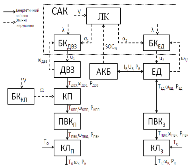
Рисунок 1 – Структурна схема автомобіля з ГСУ послідовного типу
