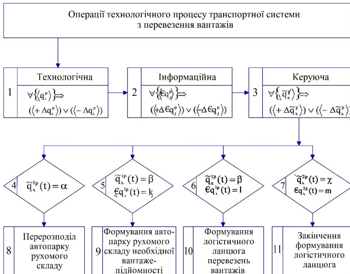
Рисунок 1 - Вигляд блок-схеми процесу ухвалення рішення на прикладі прибуття автопарку рухомого складу під навантаження в моделі логістичного вузла
