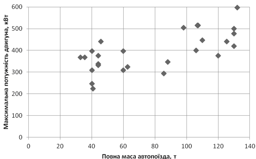
Рисунк 1 – Відповідність максимальної потужності двигуна до повної маси автопоїздів військового призначення
