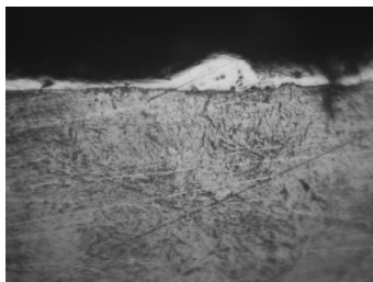
Рисунок 2 – Типові мікроструктури зміцненого поверхневого шару шипа зі сталі 45, отримані за використання як анод твёрдих сплавів ВК8 (а) та Т15К6 (б) (x500).
