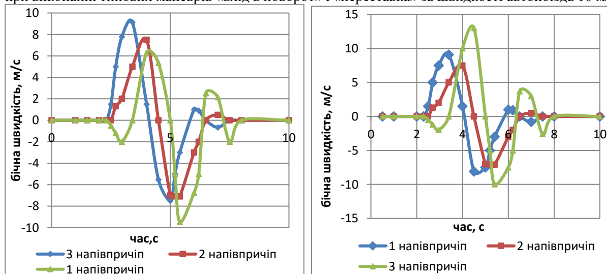
Рисунок 2 - Зміни бічної швидкості напівпричепів при виконанні типових маневрів «вхід в поворот» (а) і «переставка» (б) за швидкості автопоїзда 10 м/с
