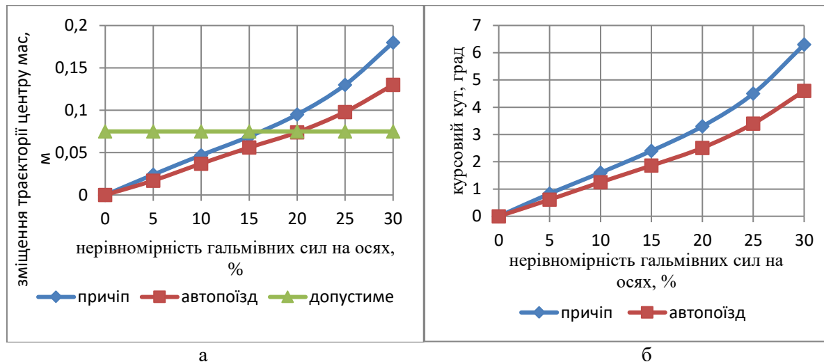
Рисунок 2 - Зміщення курсового кута (а) і зміщення траєкторії автомобіля і причепа від нерівномірності гальмівних сил на здвоєній осі причепа
