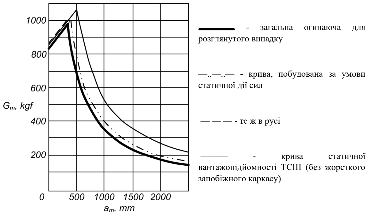
Рисунок 3 – Залежність значень граничної ваги, агрегатованої машини від величини горизонтальної координати її центру ваги (для статичних та динамічних умов)
