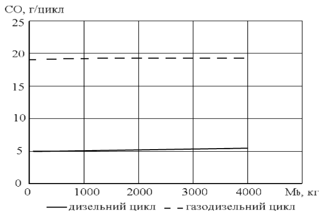
Рисунок 1 - Залежність масових викидів CO за цикл, в залежності від навантаження при роботі двигуна за дизельним і газодизельним циклами.
