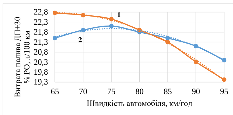
Рисунок 1 – Витрата біопалива (дизельне паливо + 30% за об'ємом ріпакової олії) автомобіля ГАЗ-33060 від швидкості руху: 1 – розрахункова; 2 – експериментальна.
