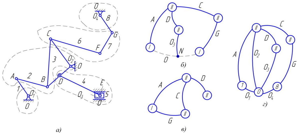
Рис.2. Багатоланковий плоский механізм з двома механізмами I класу та його можливі графи
