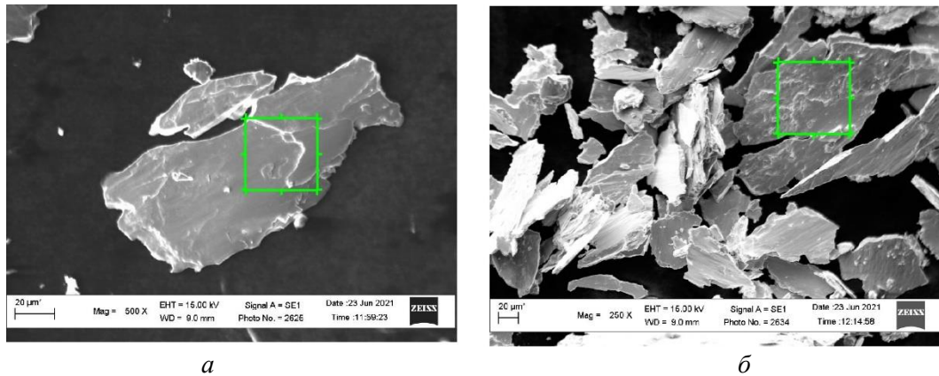
Рисунок 1. Фотографія частинок зносу, що утворилися в умовах сухого тертя ( p = 250 Н): без наводнення (а) та після електролітичного наводнення (б). Зеленим кольором окреслено квадрат, площа якого досліджувалася за допомогою системи комп'ютерного зору [4].
