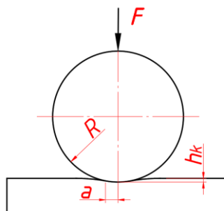
Рисунок 1 – Розрахункова схема для визначення зусилля формування канавок мікрорельєфу
