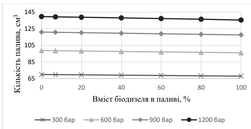
Рисунок 1- Розрахункова кількість палива при різному тиску і паливних сумішах
