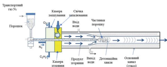
Рис. 6. Детонаційне напilenня
