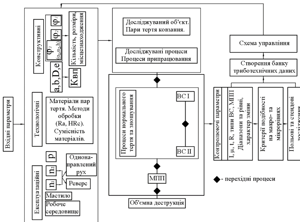
Рисунок 3 - Параметрична модель дослідження перехідних процесів в зоні фрикційного контакту важконавантажених трибоспряжень.
