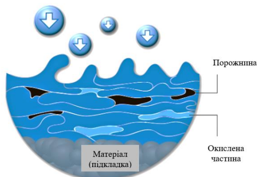
Рис. 1. Термічне напilenня металу
