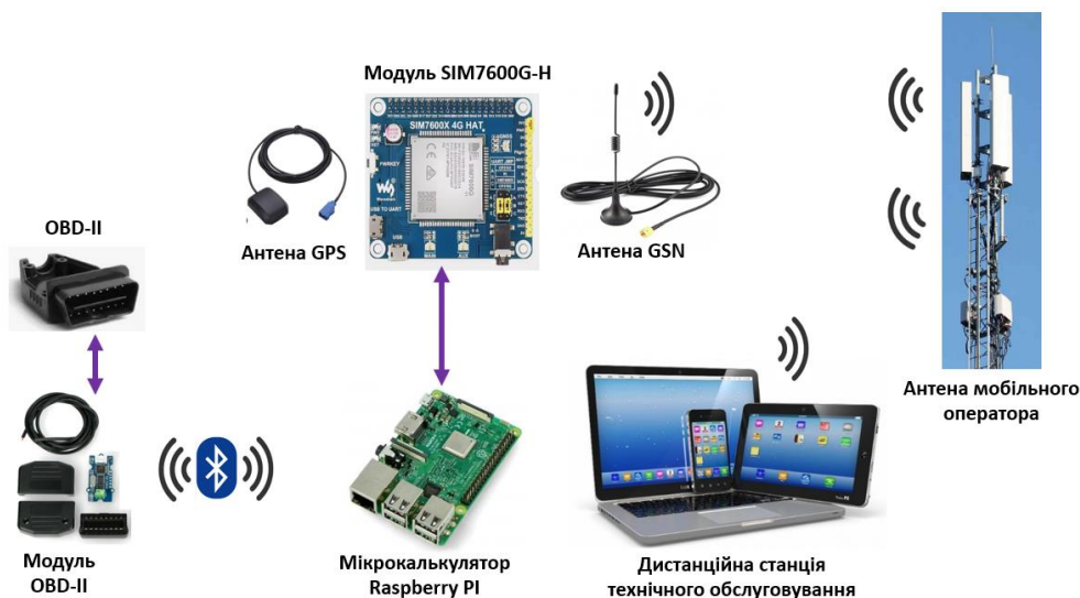
Рисунок 1 – Запропонована система пристрою дистанційної діагностики автомобіля
