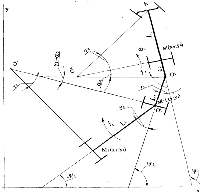
Рисунок 1 - Схема повороту автобусного поїзда
