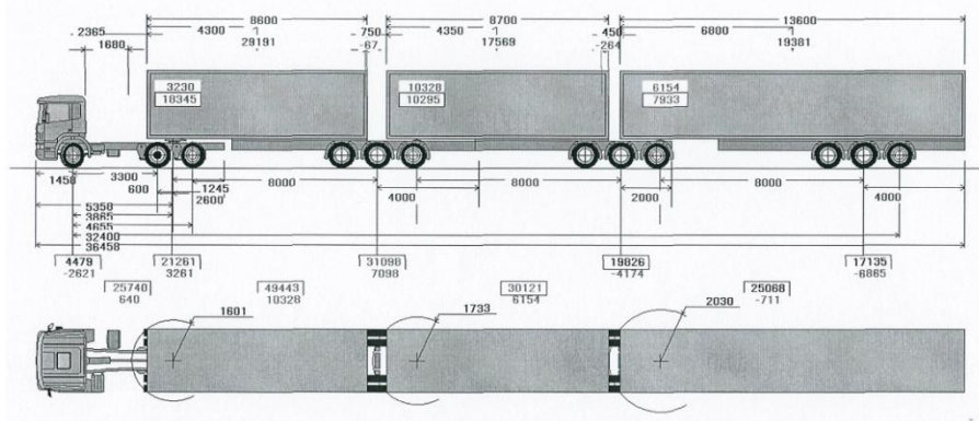
Рисунок 1 – Триланковий автопоїзд типу B-triple
