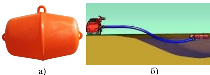
Рис. 1. Принцип використання буя: а) «поплавок» для всмоктуючої сітки; б) практичне використання «поплавок» при заборі води з водойми
