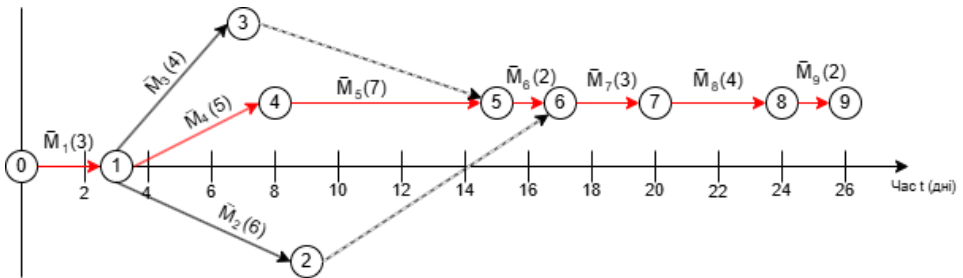
Рис. 1. Часовий мережевий графік проекту розробки модуля збору даних
