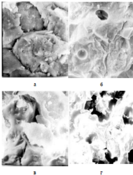
Рис. 2. Изменение микроструктуры защитного покрытия при нагревании:
