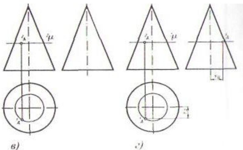
Рис. 1.9. Побудова проєкцій належної поверхні конуса точки
