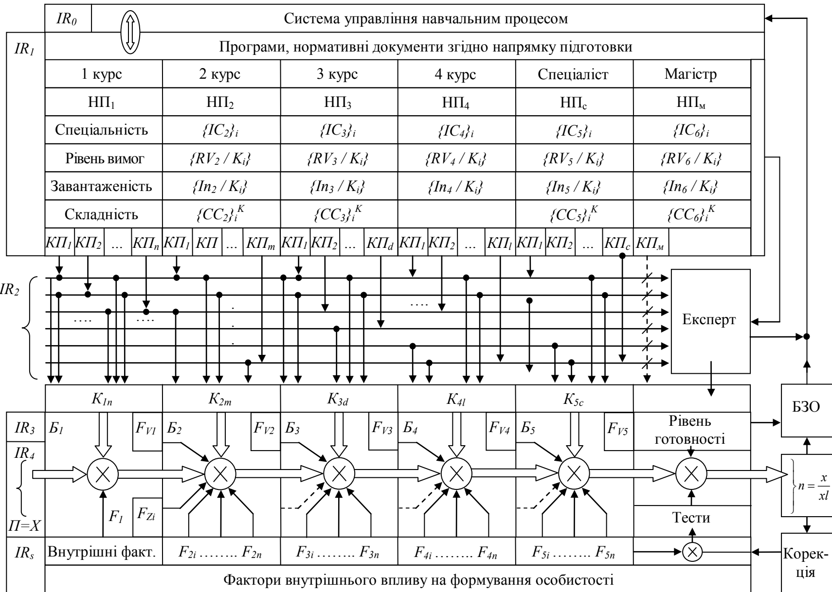
Рис. 3. Схема факторів впливу на компоненти навчального процесу
