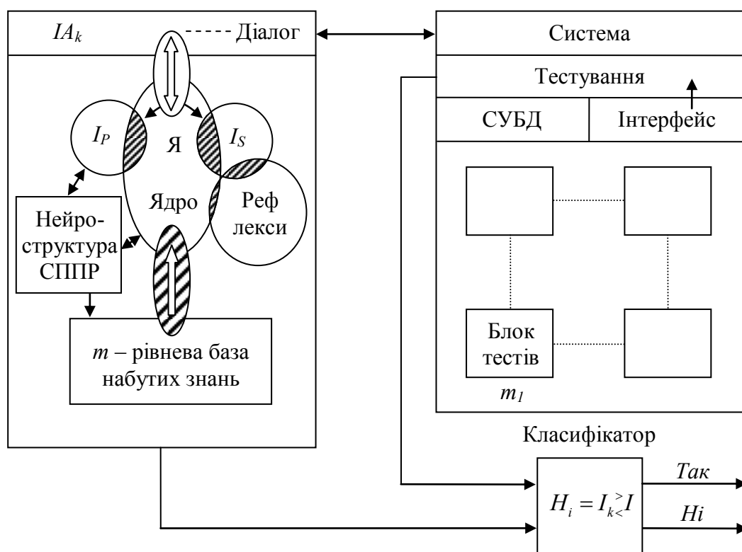
Рис. 5. Схема інтерфейсу діалогу тестування
