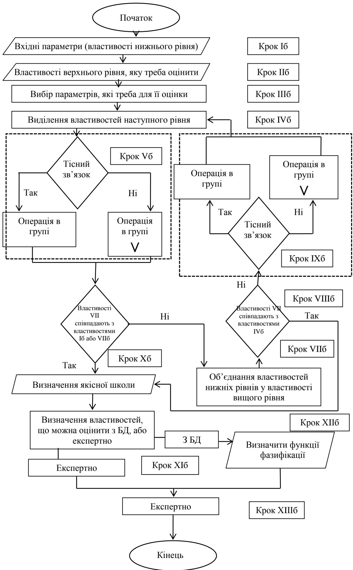
Рис. 3 Алгоритм побудови моделі №3
