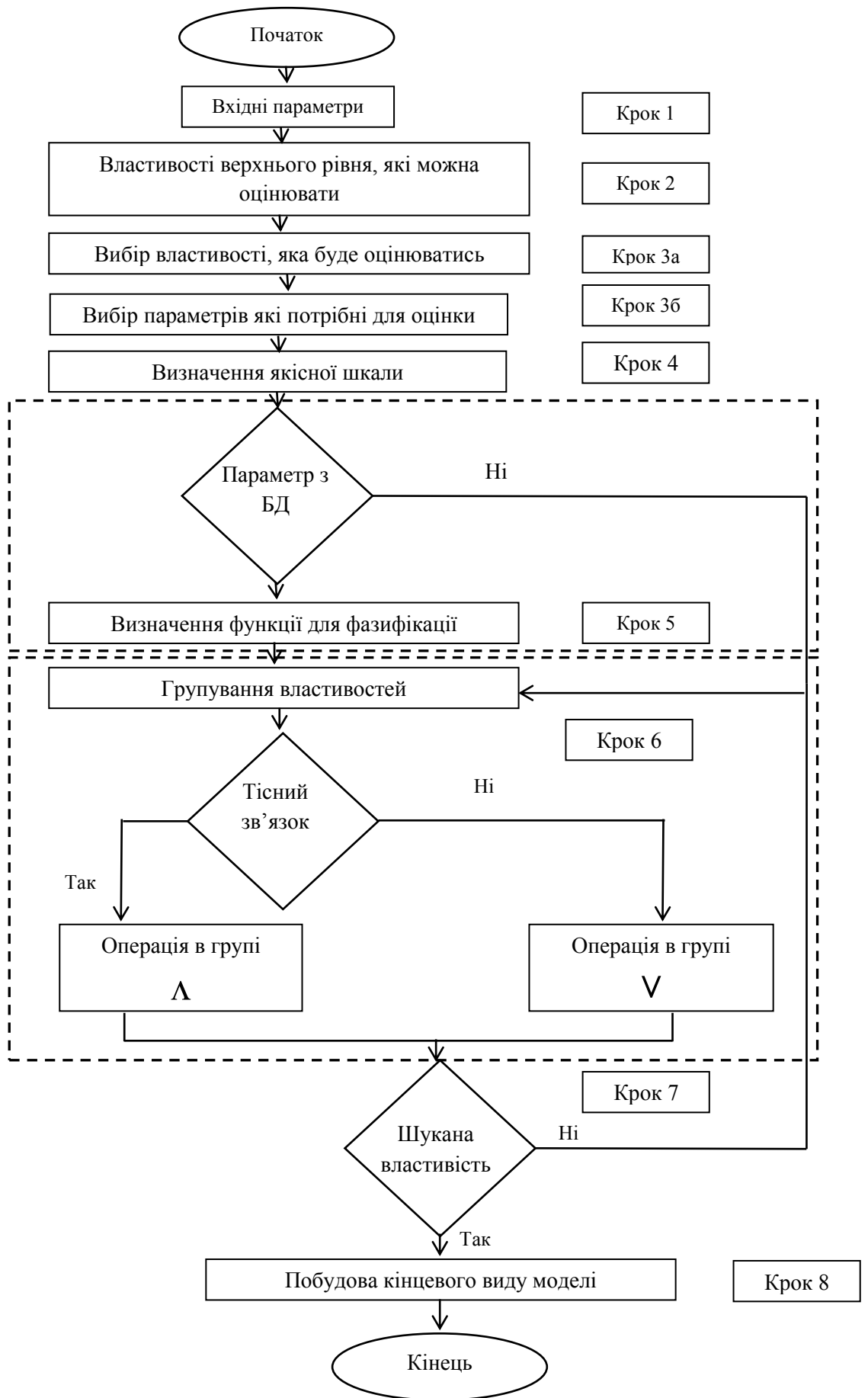
Рис. 1 Алгоритм синтезу “знизу-вверх” побудови моделі №1.
