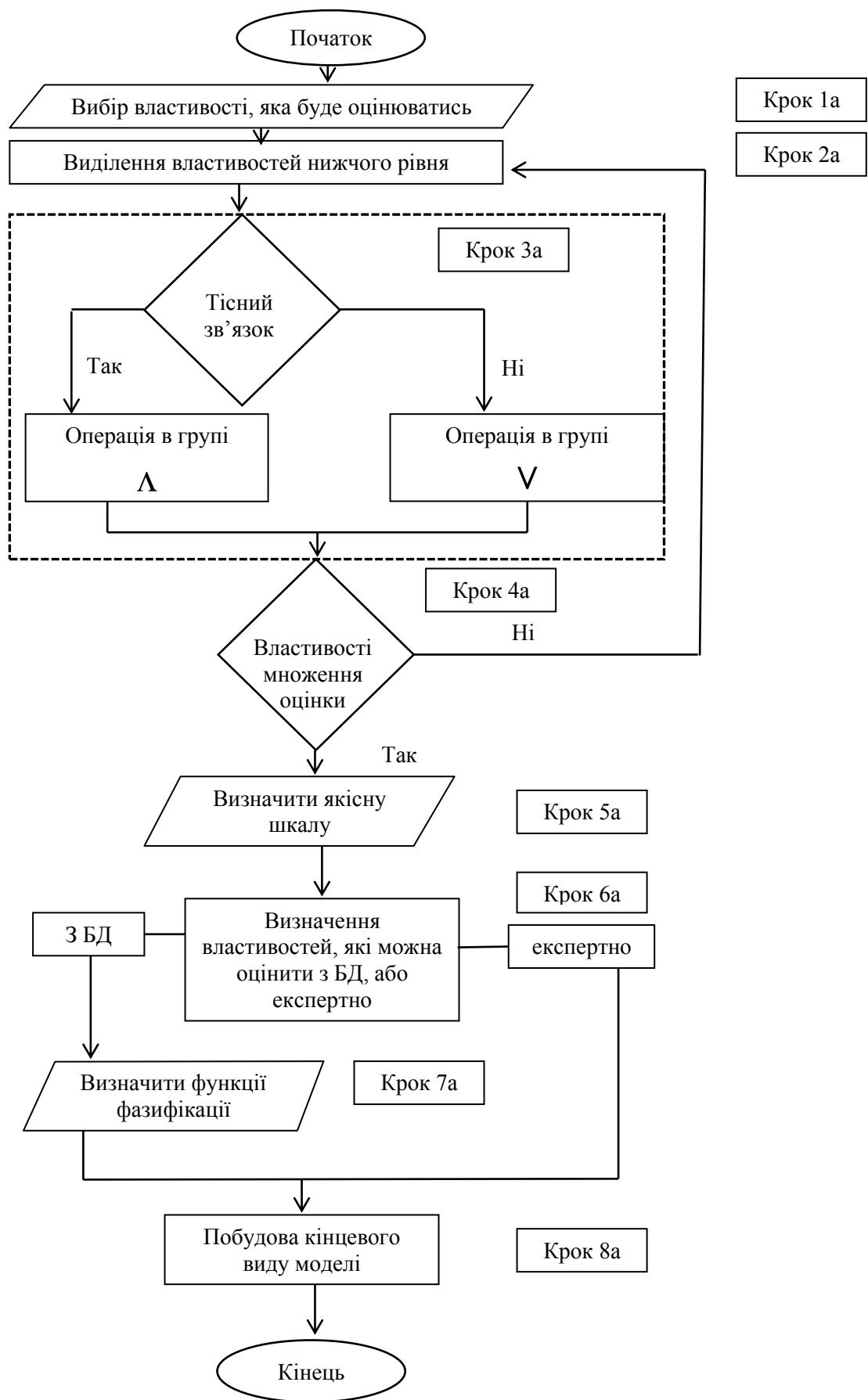
Рис. 2 Алгоритм аналізу “зверху-вниз” побудови моделі №2
