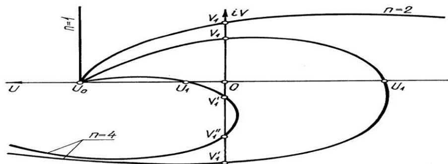
Рис.2.Годографи характеристичних рівнянь
