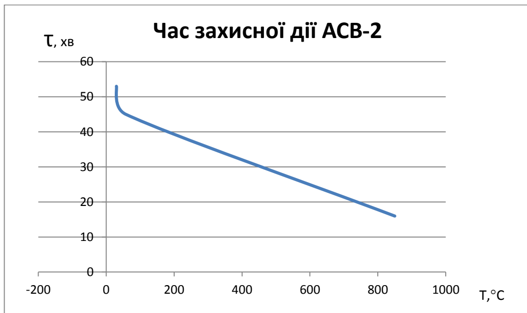
Рисунок 5 - Залежність часу захисної дії ЗДА від температури пожежі у приміщенні
