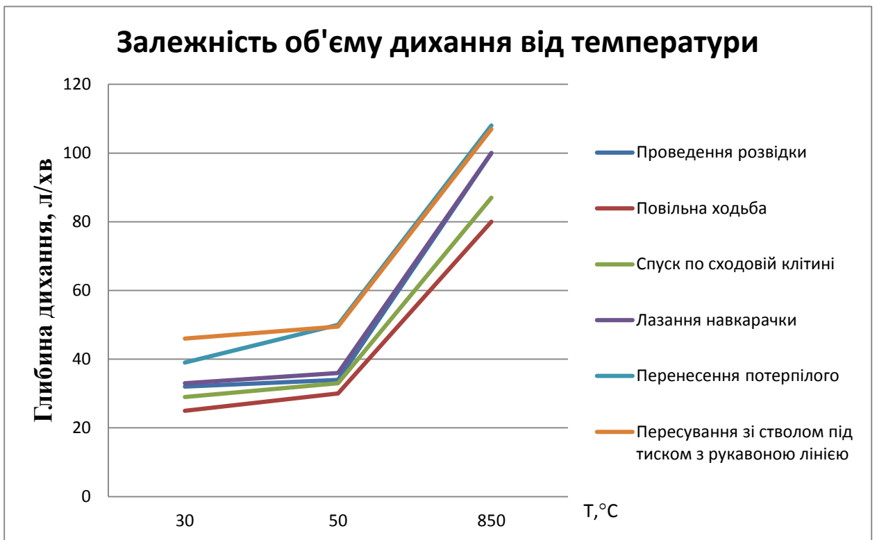
Рисунок 4 - Залежність витрати повітря від температури в приміщенні під час пожежі
