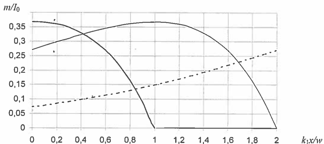
Рисунок 2 – Кривые распределения вдоль канала зоны горения в различные моменты времени (жирная линия – k_1\tau = 1 , тонкая линия – k_1\tau = 2 , штриховая линия – k_1\tau = 4 )
