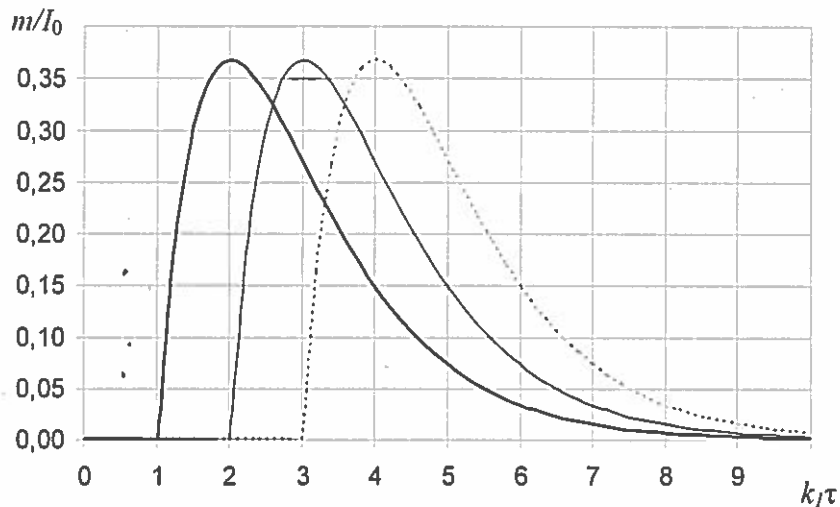
Рисунок 1 – Кривые развития и перемещения очага горения вдоль канала (жирная линия – k_1x/w = 1 , тонкая линия – k_1x/w = 2 , штрих-линия – k_1x/w = 3 )
