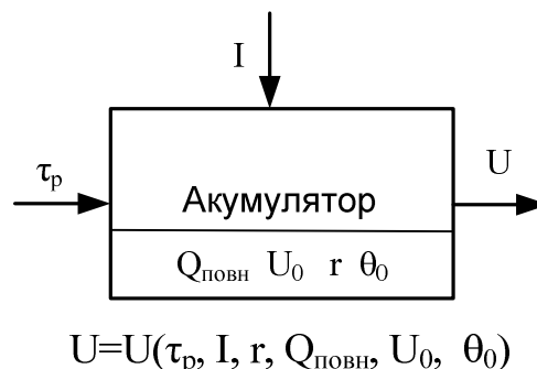
Рисунок 3 – Структура математичної моделі електромеханічного акумулятора в режимі розряду
