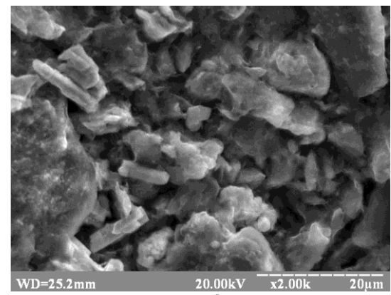
Рисунок 3 – Мікрофотографії поверхні бентоніту: а – нативного; б – «прямого опромінення».
