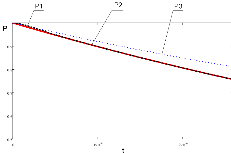
Рисунок 2 – Залежність ймовірності безвідмовної роботи систем електроживлення: P1- основної (P oc ), P2- резервованої системи з генераторною установкою, P3 - резервованої системи з генераторною установкою та акумуляторними батареями з інверторами напруги
