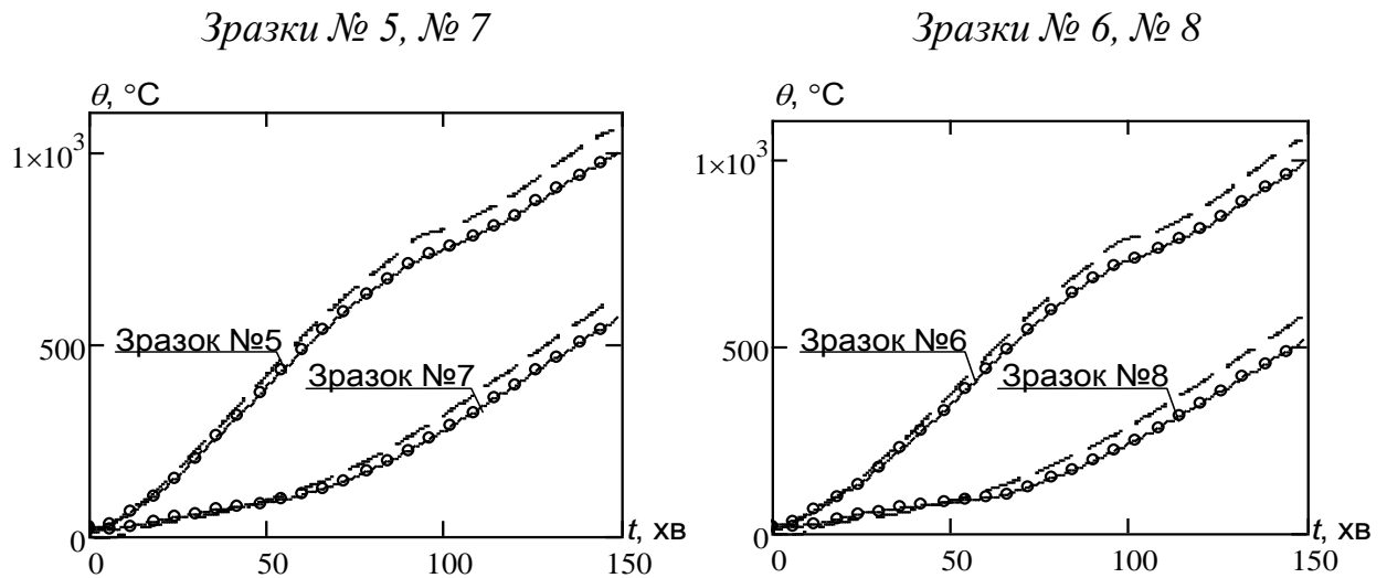
Рис. 3.14 Графіки температурних режимів прогрівання залежностей сталевих елементів стержнів із мінераловатним вогнезахисним облицюванням: \circ-\circ-\circ - експериментальні дані; --- - розрахункові дані.
