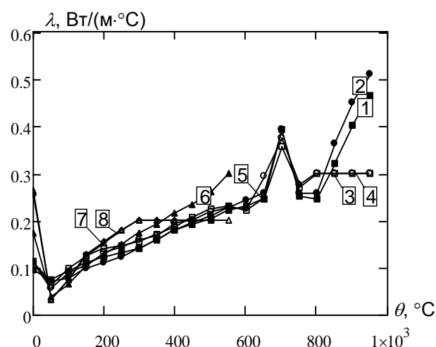
Рис. 3.12 Залежність усередненого значення коефіцієнта теплопровідності від температури зразків фрагментів сталевих стержнів із вогнезахисним облицюванням (1, 2, 3, ... – номери зразків)
