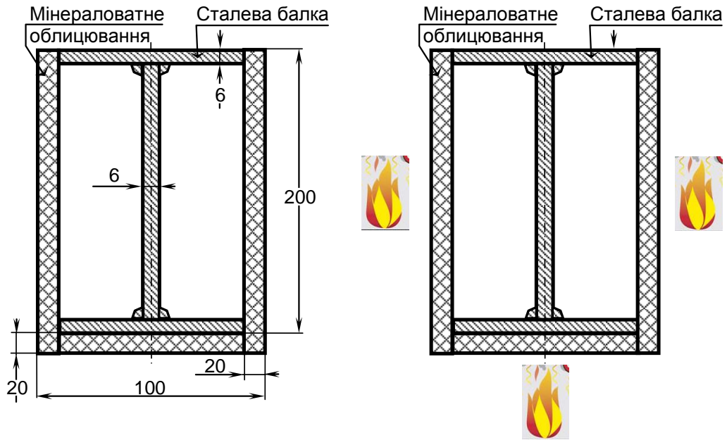
Рис. 4.1 Геометрична схема перерізу сталеві балки з мінераловатним вогнезахисним облицюванням (а) та схема теплового впливу пожежі на переріз балки (б)
