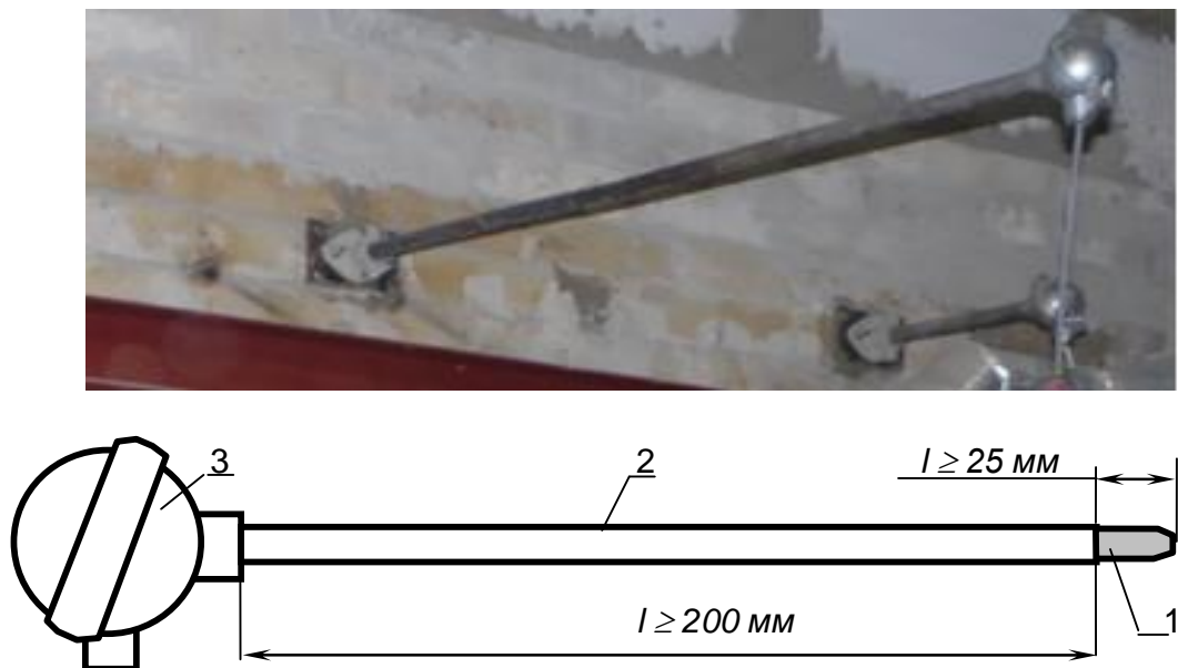
Рис. 2.4. Зовнішній вигляд та схема термопар для вимірювання температури у вогневій камері печі: 1 – вимірювальний спай термопар; 2 – захисний кожух; 3 – теплозахисна оболонка.
