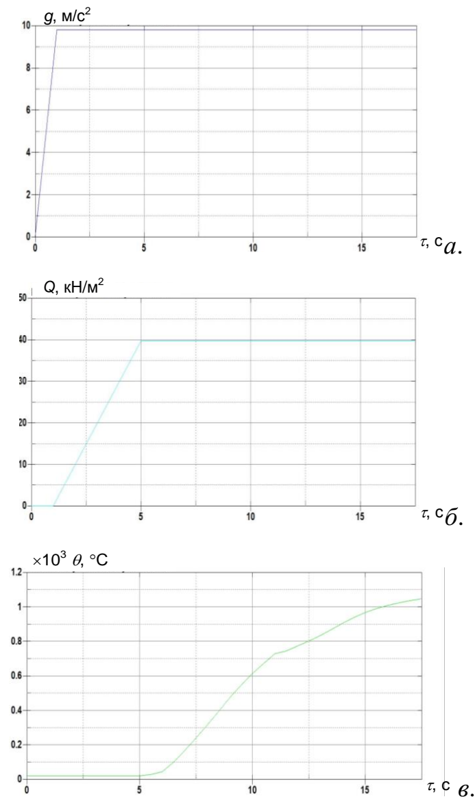
Рис. 4.14 Графіки залежності прикладених навантажень від часу: а – графік прискорення вільного падіння для врахування власної ваги; б – графік прикладення розподіленого навантаження; в – графік прикладення температурного навантаження
