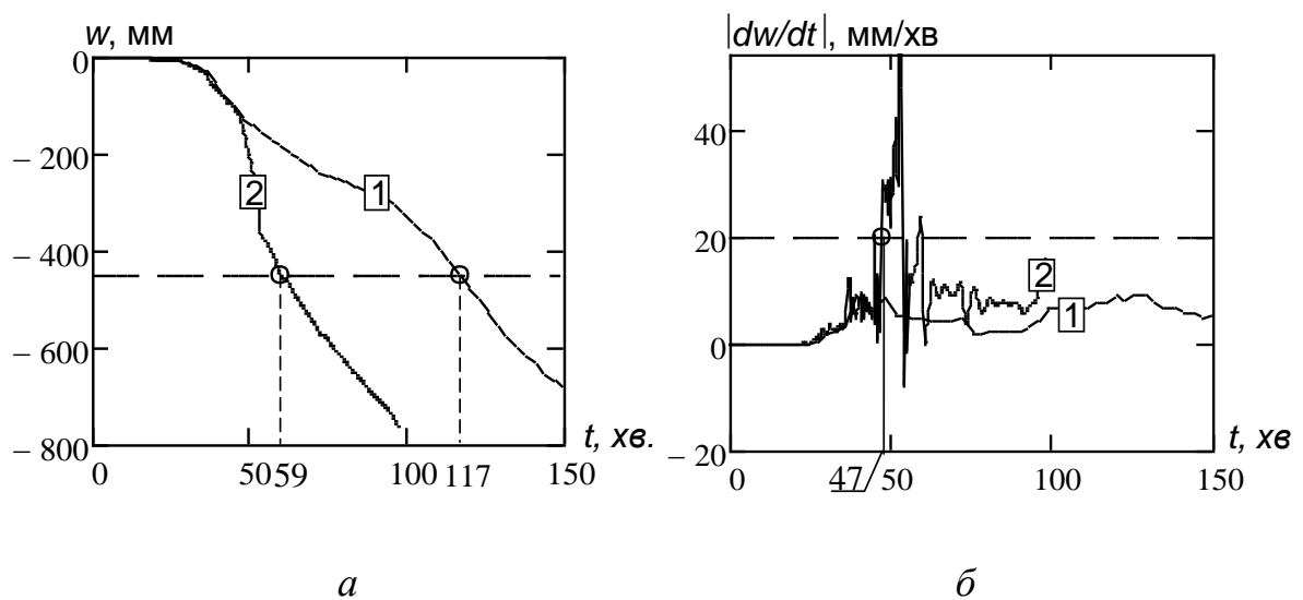
Рис. 5.4 Графіки зміни максимального прогину балки (а) та швидкості нарощування максимального прогину (б) залежно від часу впливу стандартного температурного режиму пожежі: 1 – для балки з мінераловатним вогнезахистом, що не втрачає своєї цілісності; 2 – для балки з мінераловатним вогнезахистом, що втрачає свою цілісність і вогнезахисну здатність.
