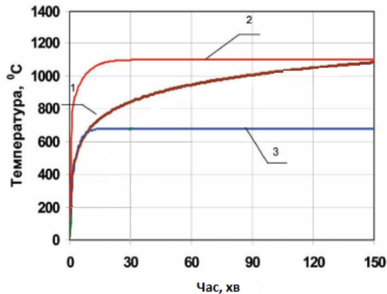
Рис. 1.5 Графік кривих температура-час номінальних температурних режимів: 1 – крива стандартної пожежі; 2 – крива вуглеводневої пожежі; 3 – крива зовнішньої пожежі
