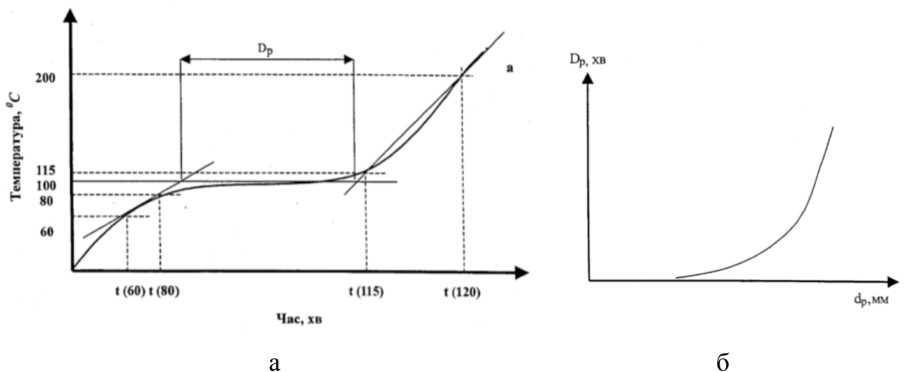
Рис. 2.10. Криві тривалості ізоtermічної ділянки, на якій зменшується вологість покриття: а – оцінювання тривалості ізоtermічної ділянки, де зменшується вологість покриття під час випробування; б – залежність тривалості ізоtermічної ділянки, на якій зменшується вологість покриття від його товщини.
