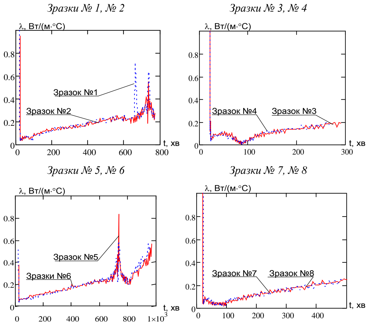
Рис. 3.11 Графіки залежностей коефіцієнта теплопровідності мінераловатного облицювання зразків фрагментів сталевих стержнів, згідно з температурою нагрівання фрагменту сталевого стержня
